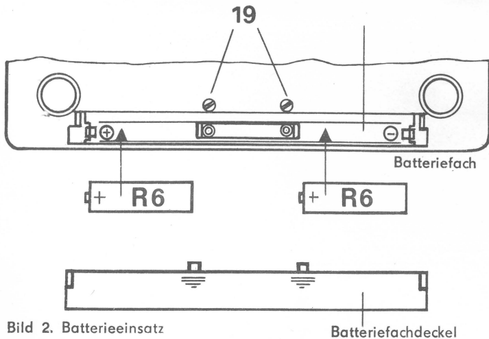
Bild 2. Batterieeinsatz
