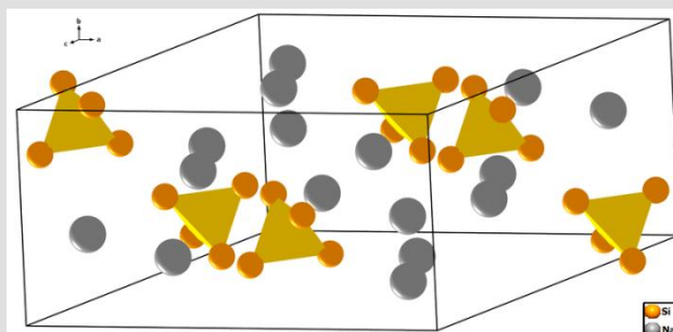
Struktur von NaSi mit Si 4 - -Tetraedern / -ZINTL-Ionen Q: de.wikipedia.org (Muskid)
