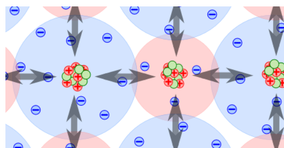
Ionen-Bindung (schematisch)
