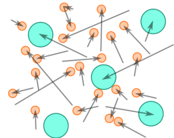
Ursache der BROWNSchen Molekular-Bewegung
