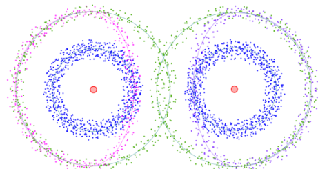
kombinierte Molekül-Orbitale (für das theoretische \text{He}_2 )
