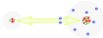
polare Atom-Bindung (gerichtete Bindung)
