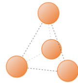
Struktur von weißem Phosphor
