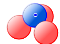
Dipol: Ammoniak
