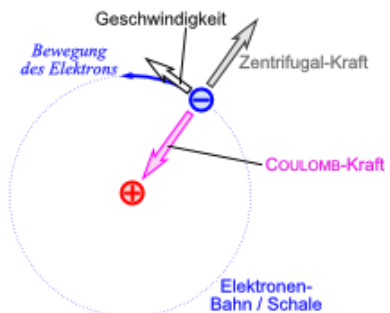
Kräfte im BOHRschen Atom-Modell
