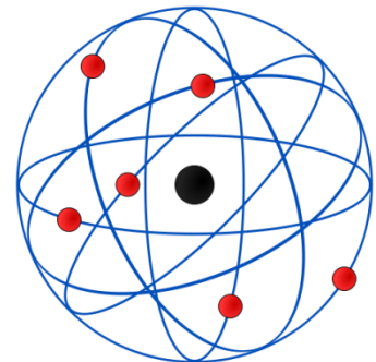
RUTHERFORDSches Atom-Modell
