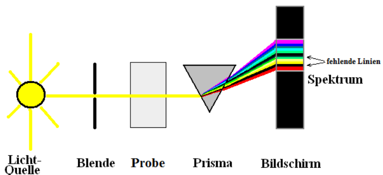
Energie-Auf- bzw. Abgabe im Atom-Modell von BOHR
