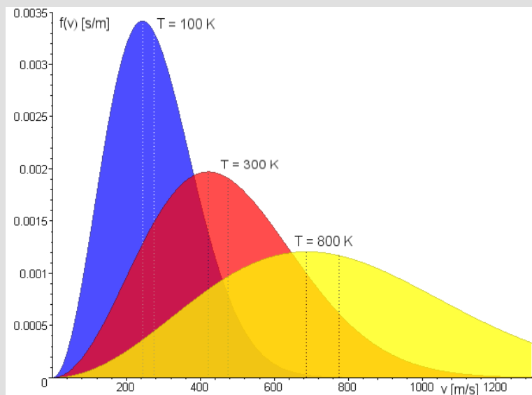
MAXWELL-BOLTZMANN-Verteilung für Stickstoff-Teilchen bei verschiedenen Temperaturen Q: de.wikipedi.org (Fred Stober)
