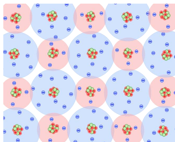
Ionen-Bindung (schematisch)
