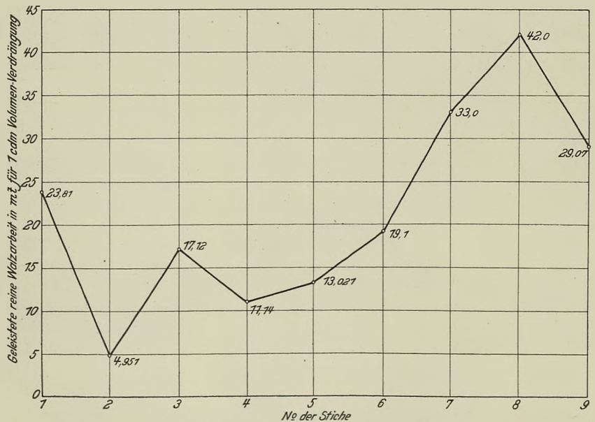
Abbildung 7. Versuche an einer Schwungradampfmaschine in Völklingen. (Zu Zahlentafel A auf S. 26 gehörig.)
