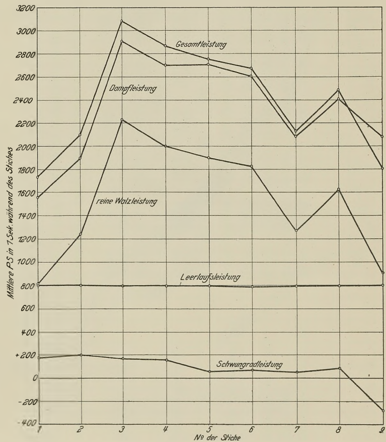
Abbild. 8. Versuche an einer Schwungraddampfmaschine in Völklingen. (Zu Zahlentafel A auf S. 26 gehörig.)
