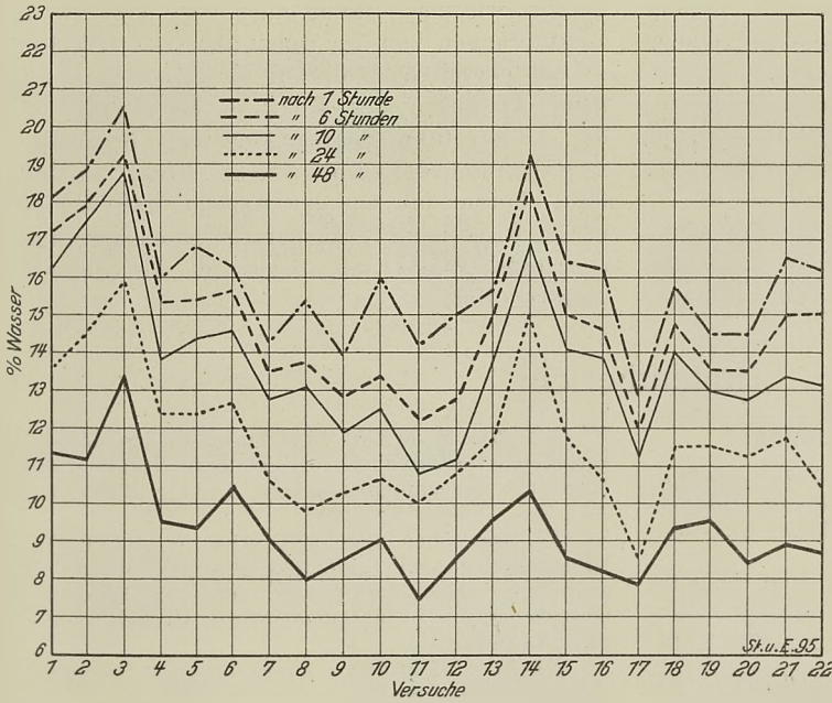
Schaubild 3. Hochofenkoks.
