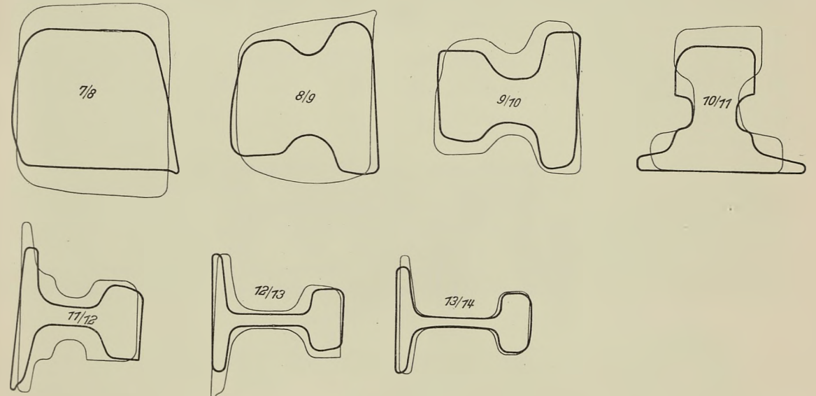
Probenummrisse des 7. bis 14. Stiches.
