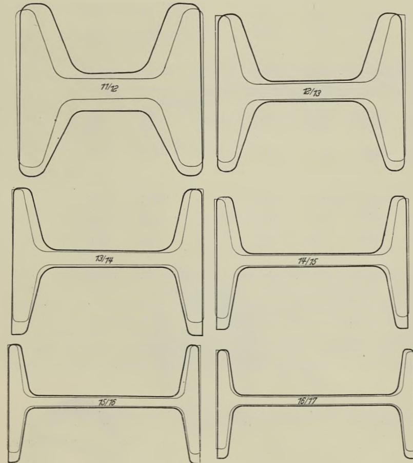
Zu Zahlentafel 57: Probenummisse des 8. bis 17. Stiches.
