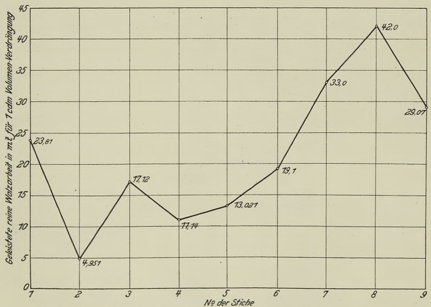
Abbildung 7. Versuche an einer Schwungradampfmachine in Völklingen. (Zu Zahlentafel A auf S. 26 gehörig.)
