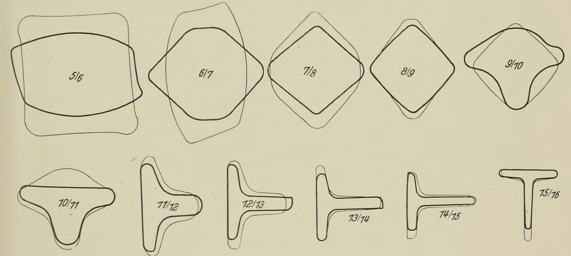
Probenummisse des 5. bis 16. Stiches.
