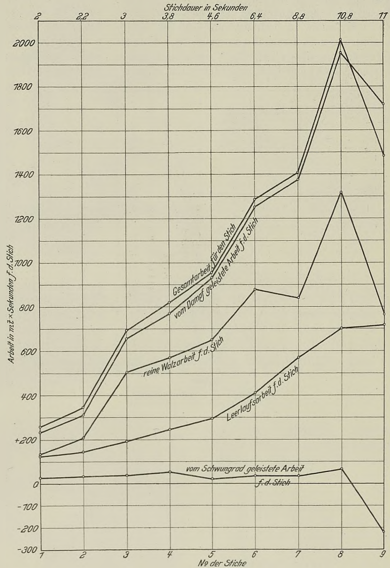
Abbild. 9. Versuche an einer Schwungrad dampfmaschine in Völklingen. (Zu Zahlentafel A auf S. 26 gehörig.)
