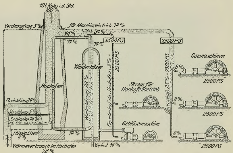
Abbildung 1. Wärmebilanz eines Hochofens von 250 t Tagesleistung.
