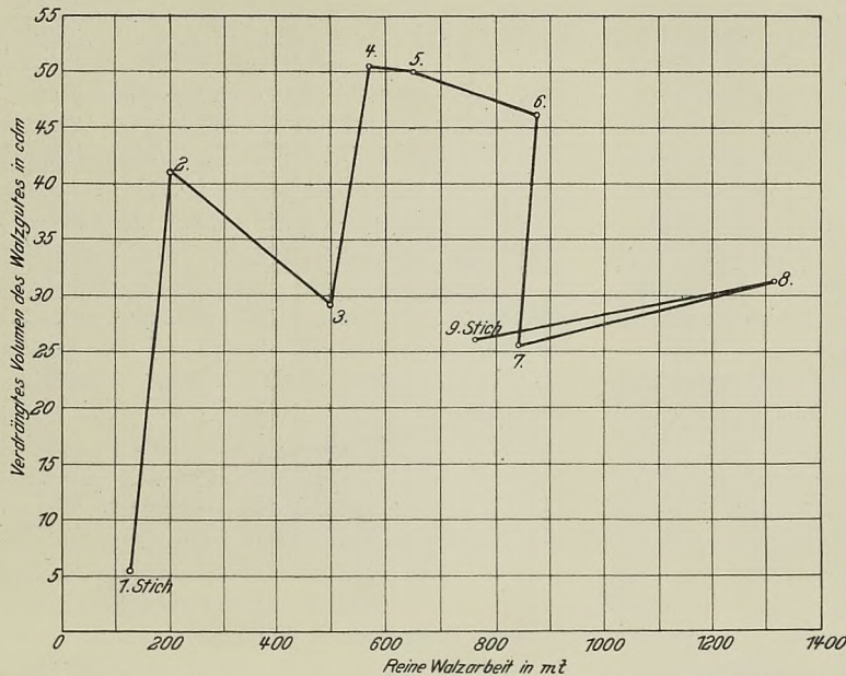
Abbildung 6. Versuche an einer Schwungradampfmaschine in Völklingen. (Zu Zahlentafel A auf S. 26 gehörig.)
