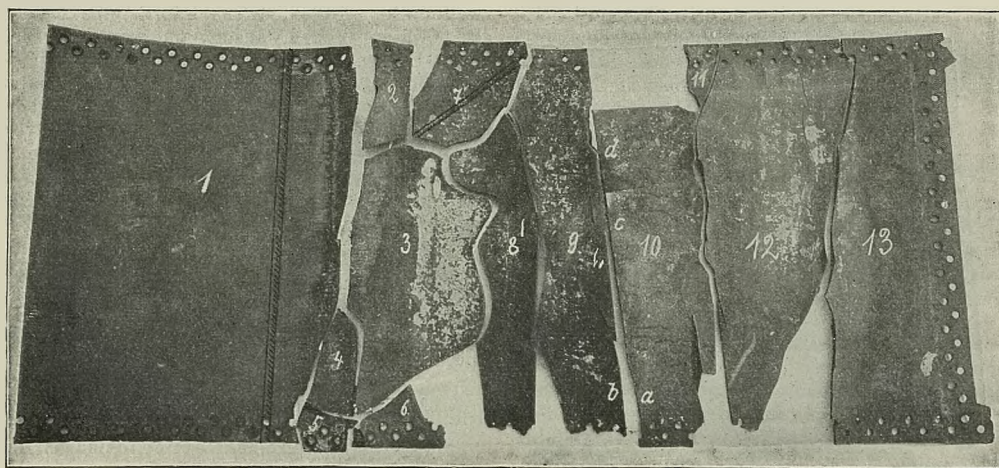
Abbildung 1. Bruchstücke des untersuchten Kesselbleches.
