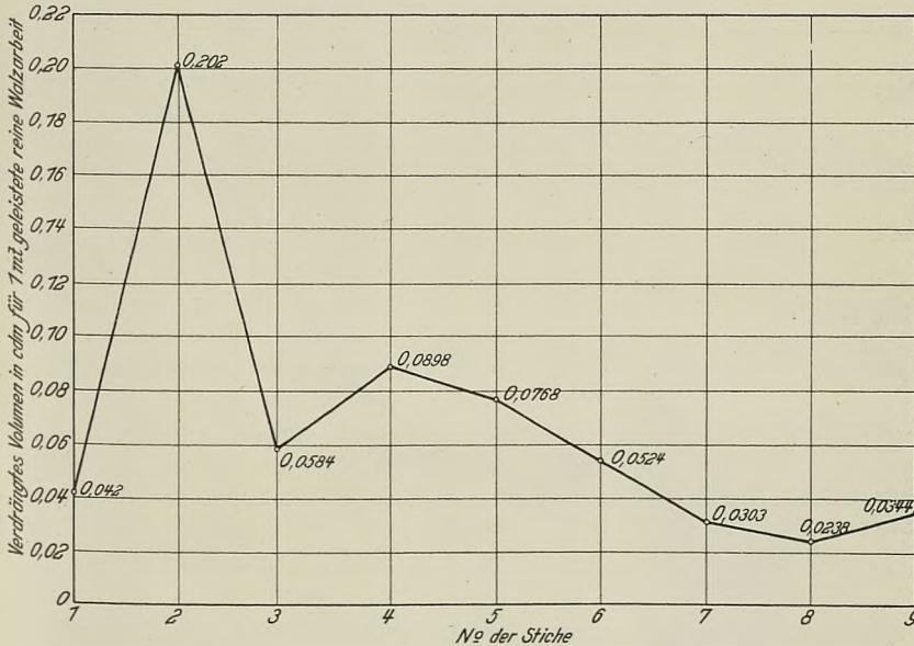
Abbildung 5. Versuche an einer Schwungradampfmaschine in Völklingen. (Zu Zahlentafel A auf S. 26 gehörig.)
