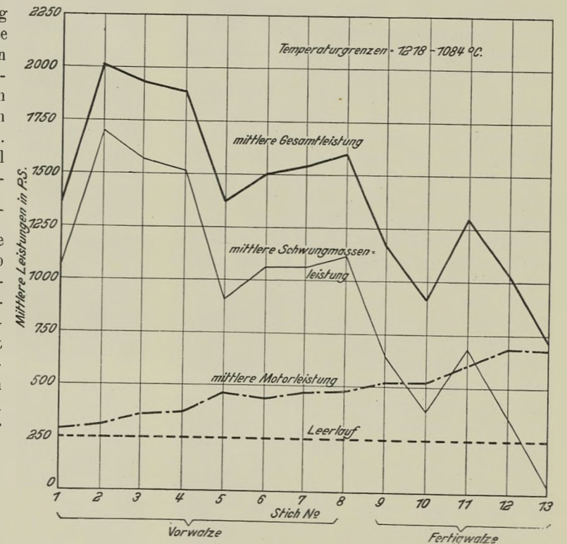
Abbildung 3. Graphische Darstellung der mittleren Leistungen beim Auswalzen eines Blockes (400,8 kg Fertiggewicht von ~ 135 × 135 mm zu Grubenschienen von ~ 13,9 kg f. d. lfde. Meter).
