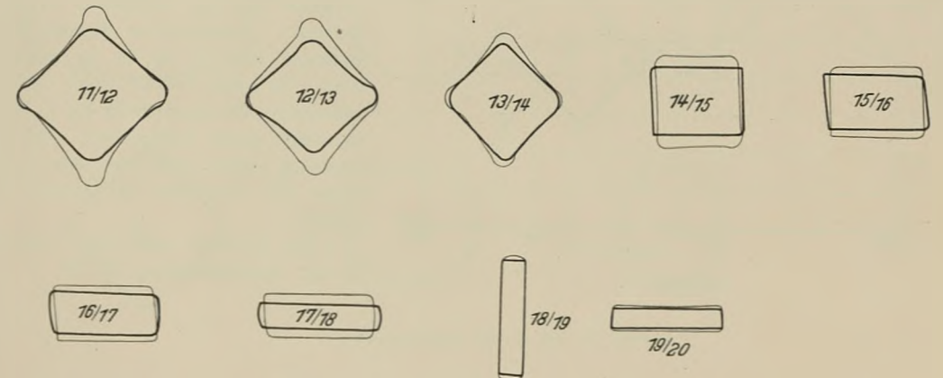
Probenumrisse des 11. bis 20. Stiches.
