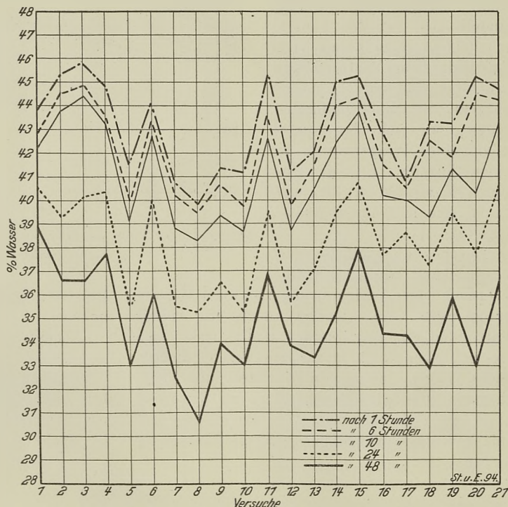
Schaubild 2. Gießereikoks.
