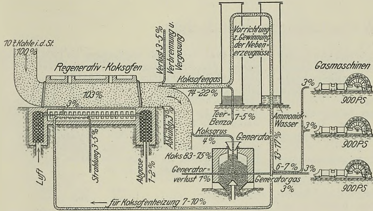
Abbildung 2. Wärmebilanz eines Koksofens von 200 t Tagesleistung.
