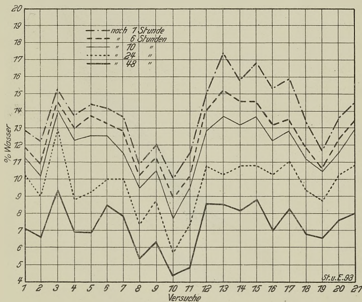
Schaubild 1. Gießereikoks.
