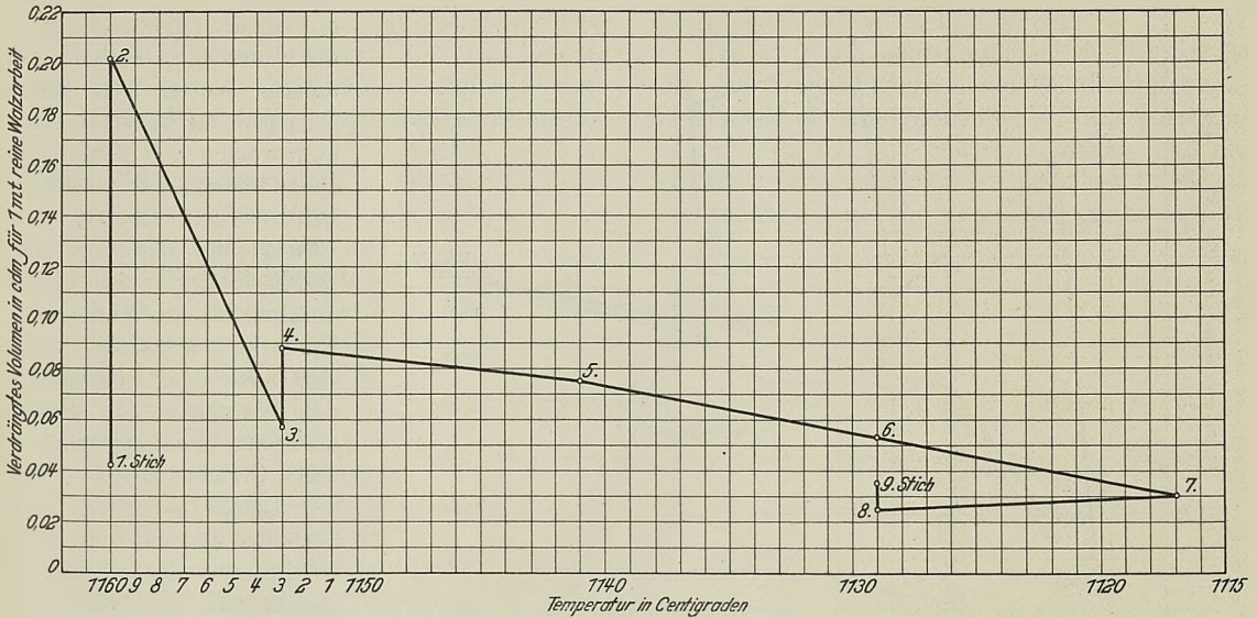
Abbildung 4. Versuche an einer Schwungrad dampfmaschine in Völklingen. (Zu Zahlentafel A auf S. 26 gehörig.)
