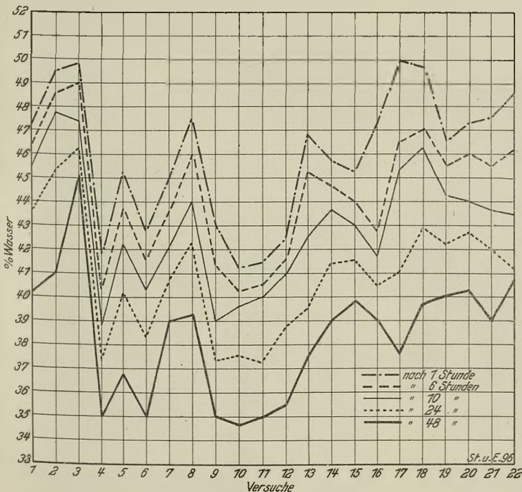
Schaubild 4. Hochofenkoks.
