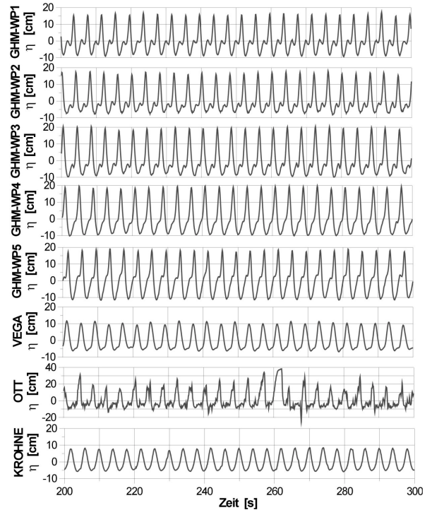
Abbildung 5-1: Wasserspiegellage als Funktion der Zeit ( H = 0,20 m, T = 4 s, WKS)
