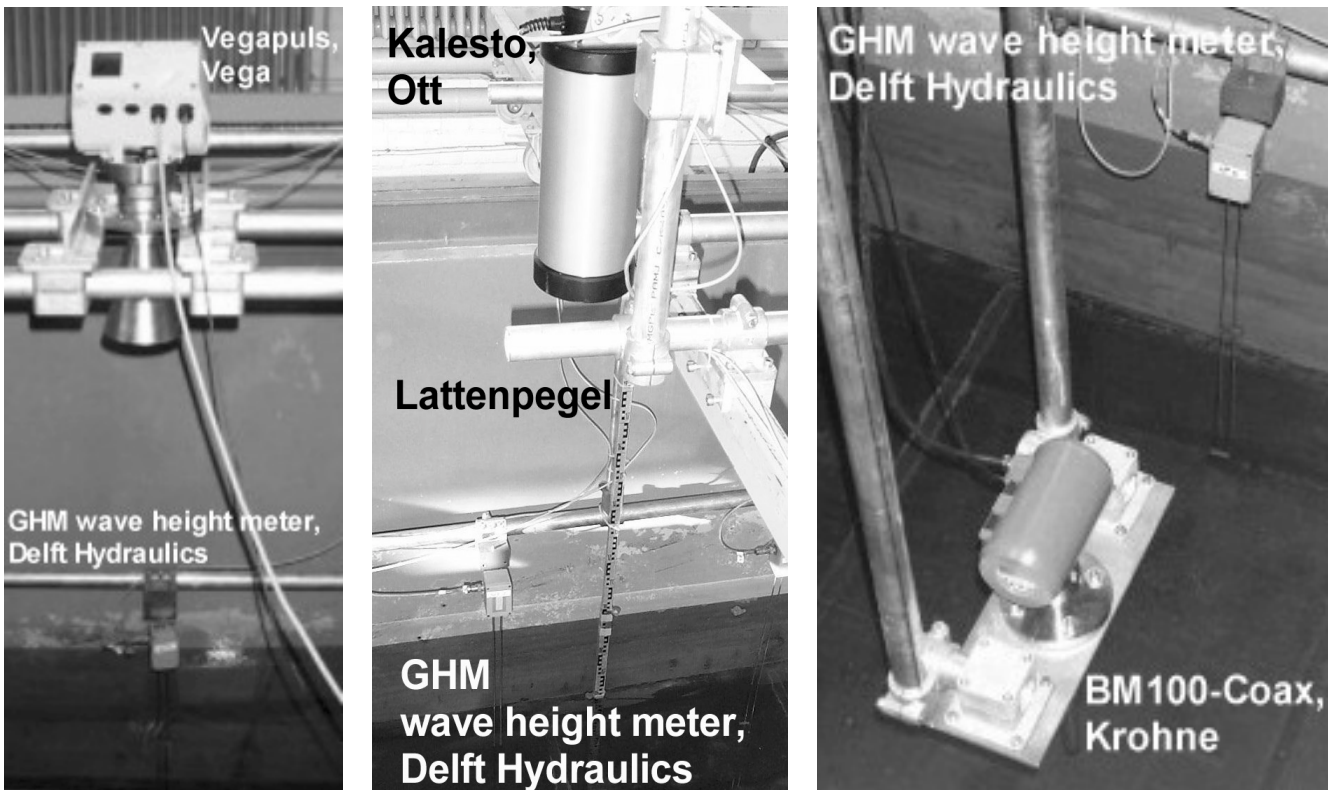
Abbildung 4-2: Zuordnung traditioneller Wellenpegel zu Radar-Sensoren
