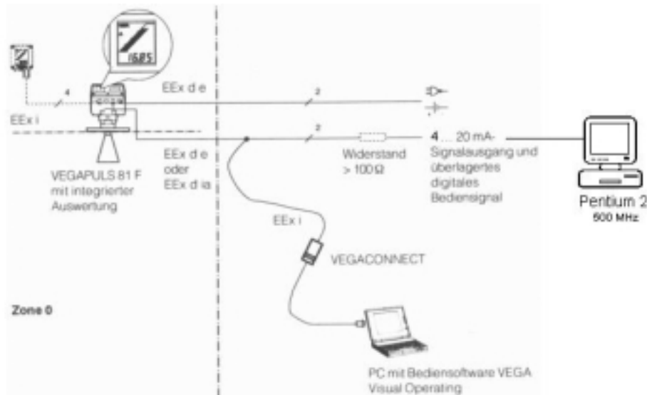
Abbildung 3-8: Meßwertfassung und Steuerung des Sensors VEGAPULS [nach VEGA GRIESHABER KG, 1999a]
