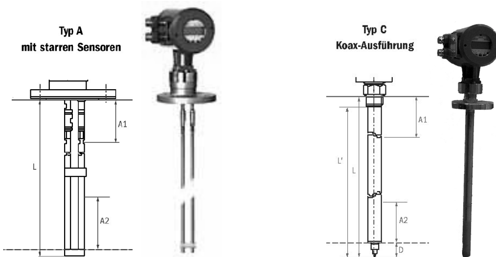
Abbildung 3-14: Skizze und Ansicht des Radar BM100, links: TYP A, rechts: TYP C [KROHNE MEßTECHNIK GMBH & Co. KG, 1996]
