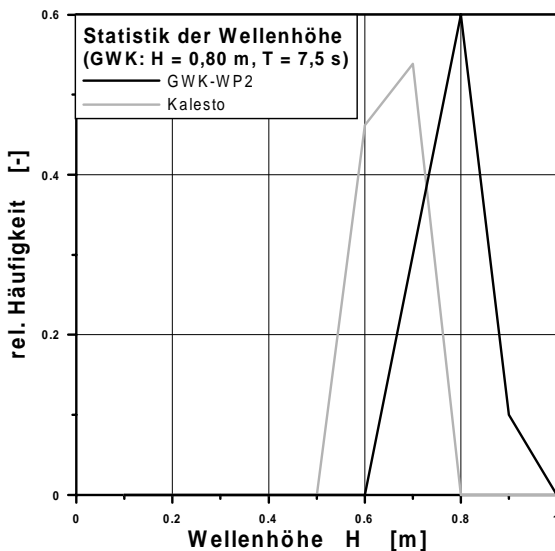
Abbildung 6-28: Statistik der Wellenhöhe im GWK bei regelmäßigem (links) und unregelmäßigem Seegang (rechts)
