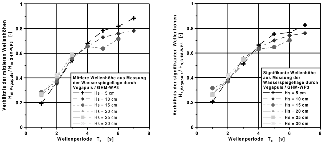
Abbildung 6-5: Verhältnis der mit den Sensoren VEGAPULS und GHM-WP3 im WKS ermittelten mittleren (links) und signifikanten Wellenhöhen (rechts) bei unregelmäßigem Seegang und seine Abhängigkeit von Wellenperiode und -höhe
