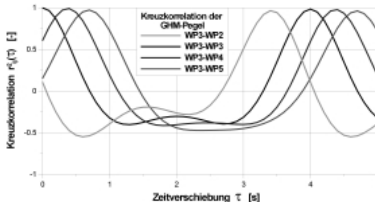
Abbildung 5-2: Kreuzkorrelation – beispielhaft für mit die mit zwei Wellenpegeln des Typs GHM gemessene Wasserspiegelauslenkung (Versuch im WKS mit regelmäßigen Wellen: H = 20 cm, T = 4,0 s)
