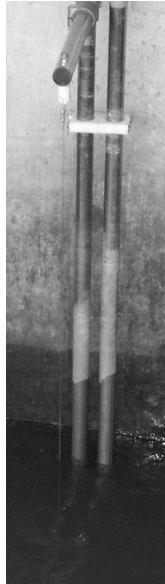
Abbildung 3-4: Ansicht des GWK-Drahtwellenpegels
