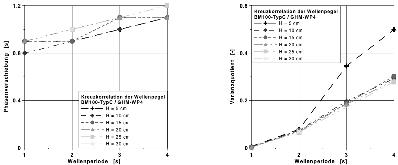
Abbildung 6-42: Abhängigkeit der Phasenverschiebung zwischen den Zeitreihen der mit den Sensoren BM100-Typ C und GHM-WP4 gemessenen Wasserspiegelauslenkung (links) und des Varianzverhältnis (rechts) von Wellenperiode und -höhe bei regelmäßigem Seegang
