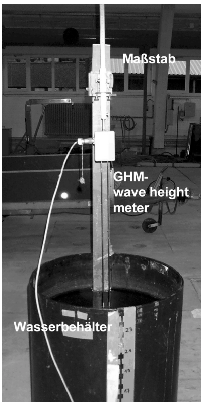
Abbildung 3-3: Eichung der Wellenpegel GHM
