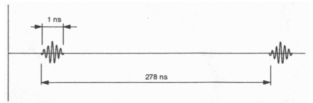
Abbildung 3-8: Zeitliche Folge der emittierten Radar-Pulse beim Sensor VEGAPULS [VEGA GRIESHABER KG, 1999a]
