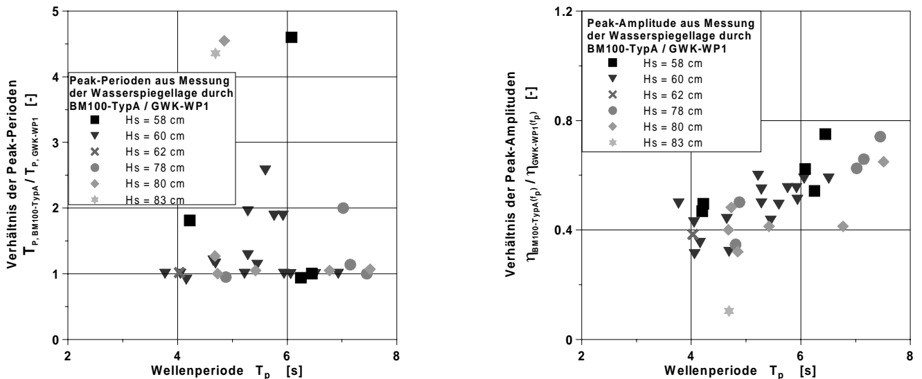
Abbildung 6-56: Verhältnis der aus Messungen von BM100-TYP A und GWK-WP2 im GWK bestimmten Peak-Perioden (links) und Peak-Amplituden (rechts)
