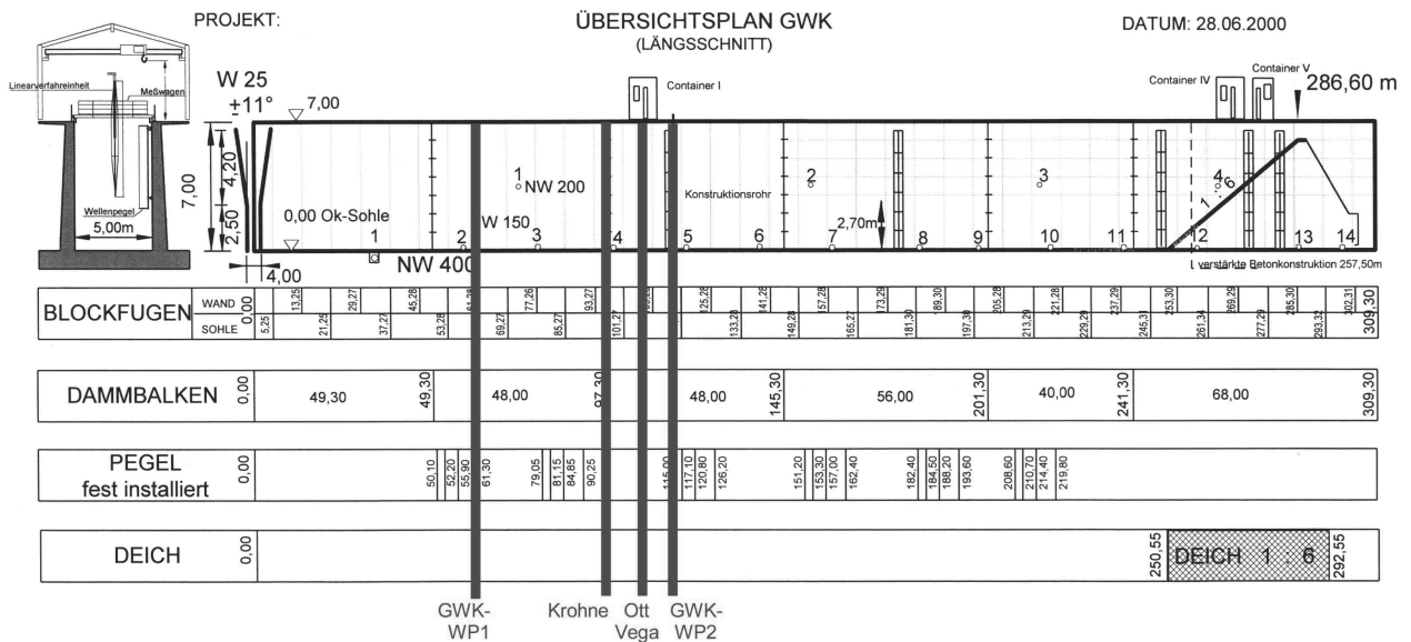
Abbildung 4-6: Position der Meßinstrumente im GROßEN WELLENKANAL GWK
