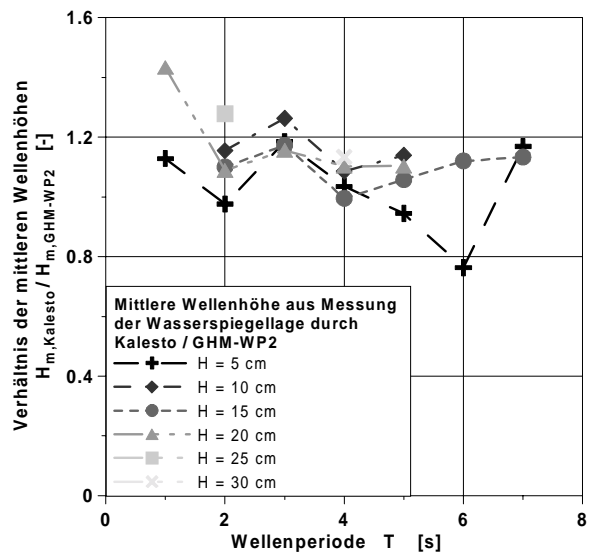
Abbildung 6-24: Verhältnis der mit den Sensoren KALESTO und GHM-WP2 im WKS ermittelten mittleren Wellenhöhen bei regelmäßigem Seegang und seine Abhängigkeit von Wellenperiode und -höhe
