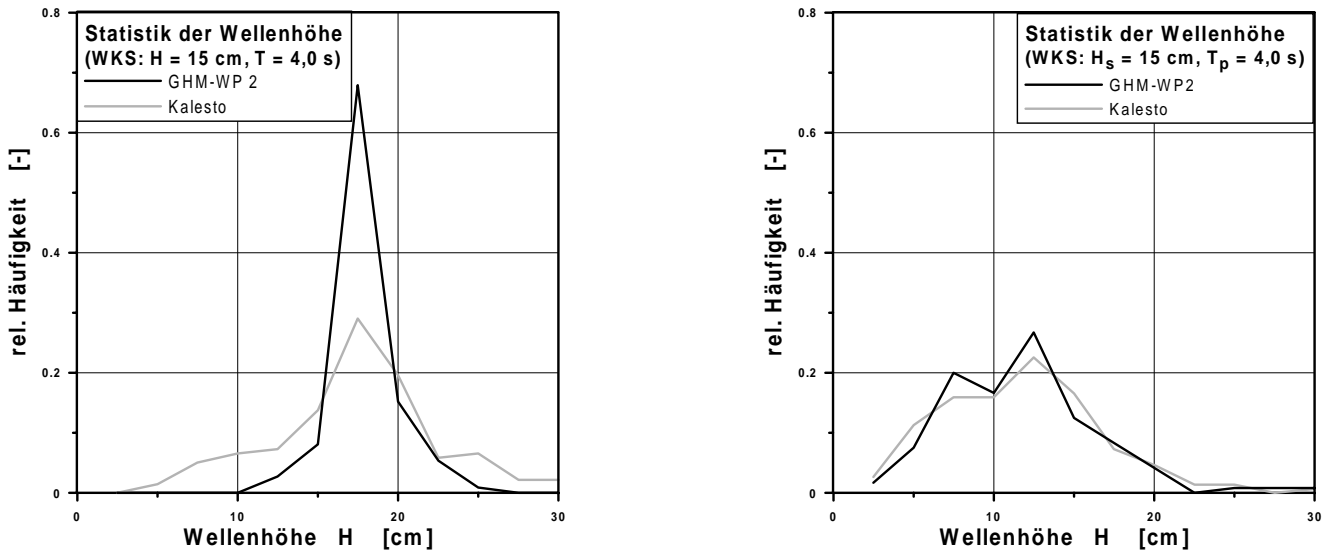
Abbildung 6-23: Statistik der Wellenhöhe im WKS bei regelmäßigem (links) und unregelmäßigem Seegang (rechts)
