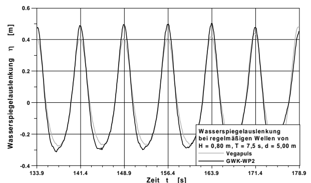
Abbildung 6-6: Zeitreihe der mit den Sensoren GWK-WP2 und VEGAPULS im GWK gemessenen Wasserspiegelauslenkung
