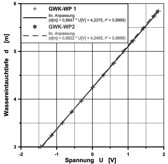
Abbildung 3-5: Eichung der GWK-Wellenpegel
