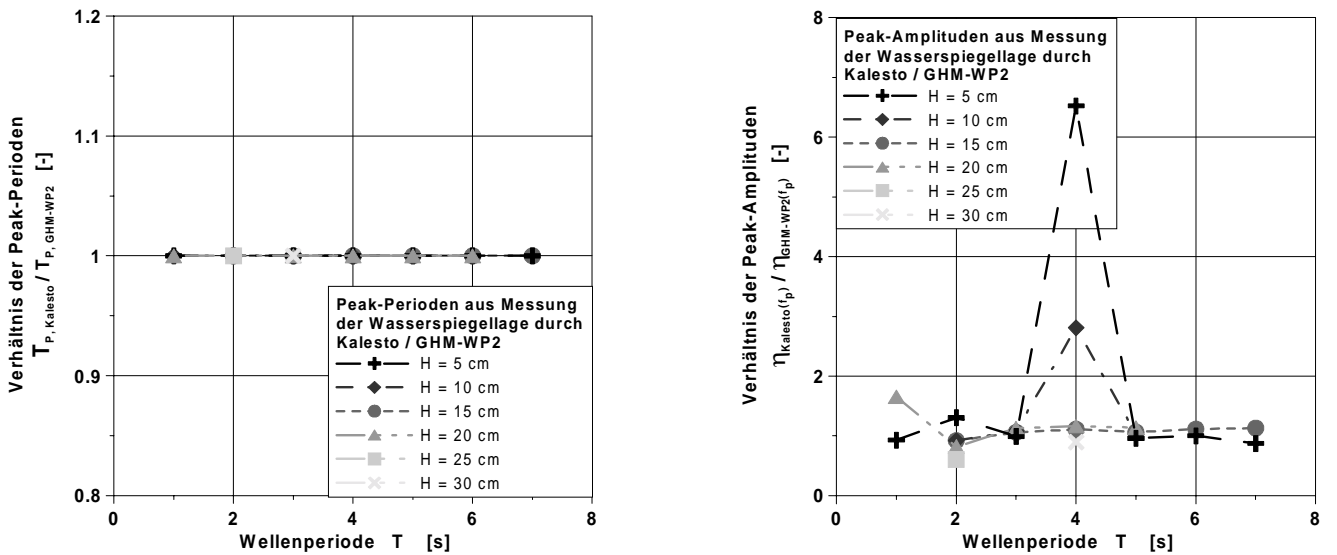
Abbildung 6-32: Verhältnis der aus Messungen von KALESTO und GHM-WP2 im WKS bestimmten Peak-Perioden (links) und Peak-Amplituden (rechts) bei regelmäßigen Wellen
