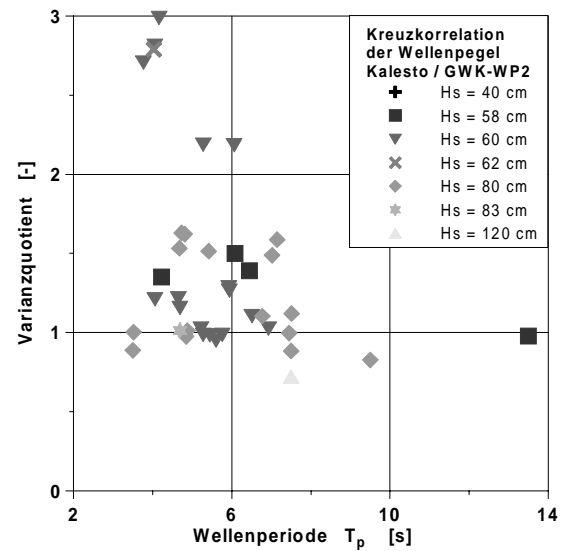
Abbildung 6-27: Abhängigkeit des Varianzverhältnisses zwischen den Zeitreihen der mit den Sensoren KALESTO und GWK-WP2 gemessenen Wasserspiegelauslenkung von Wellenperiode und -höhe bei regelmäßigem (links) unregelmäßigem Seegang (rechts)
