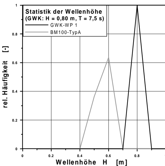
Abbildung 6-53: Statistik der Wellenhöhe bei regelmäßigem (links) und unregelmäßigem Seegang (rechts)
