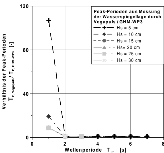
Abbildung 6-13: Verhältnis der aus Messungen von VEGAPULS und GHM-WP3 im WKS bestimmten Peak-Perioden (links) und Peak-Amplituden (rechts) bei unregelmäßigen Wellen
