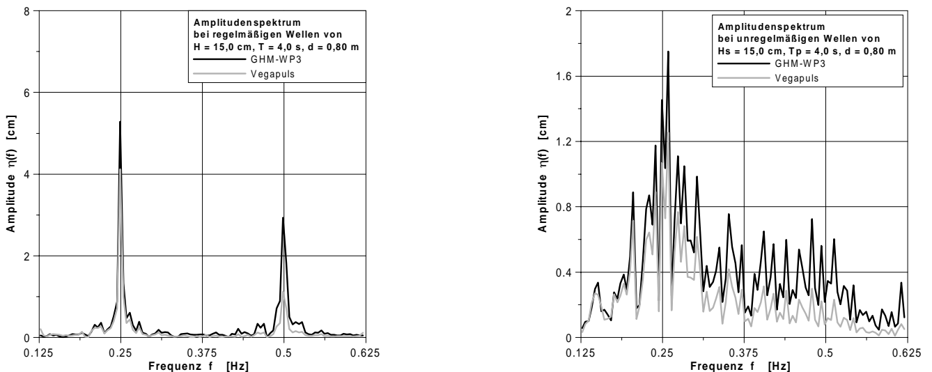
Abbildung 6-11: Amplitudenspektrum der mit den Sensoren GHM-WP3 und VEGAPULS im WKS gemessenen Wasserspiegelauslenkung bei regelmäßigen Wellen (links) und bei unregelmäßigen Wellen (rechts)
