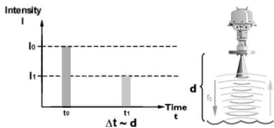
Abbildung 2-7: Meßprinzip des Radar – Wasserstandspegels – Puls-Verfahren [MAI UND ZIMMERMANN, 2000]
