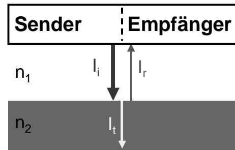
Abbildung 2-6: Schema des Strahlenganges der Mikrowellen
