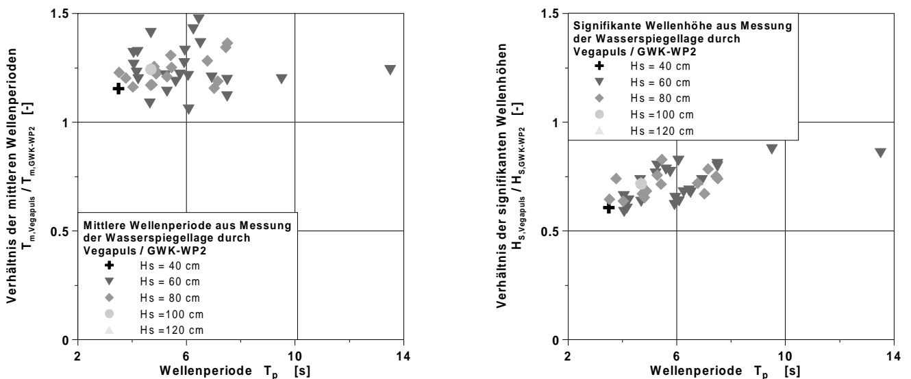
Abbildung 6-20: Verhältnis der aus Messungen von VEGAPULS und GWK-WP2 im GWK bestimmten mittleren Wellenperioden (links) und signifikanten Wellenhöhen (rechts) bei unregelmäßigen Wellen
