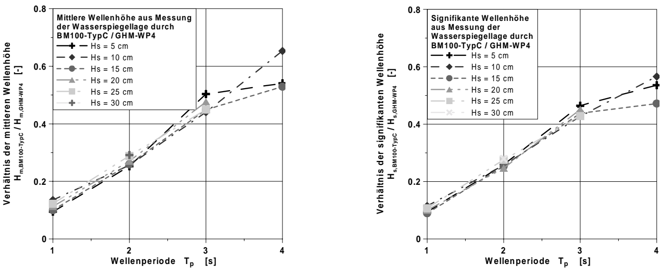
Abbildung 6-45: Verhältnis der mit den Sensoren BM100-Typ C und GHM-WP4 ermittelten mittleren (links) und signifikanten Wellenhöhen (rechts) bei unregelmäßigem Seegang und seine Abhängigkeit von Wellenperiode und -höhe
