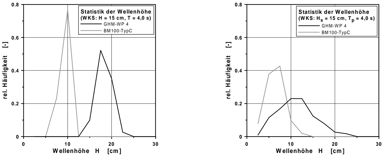
Abbildung 6-43: Statistik der Wellenhöhe bei regelmäßigem (links) und unregelmäßigem Seegang (rechts)
