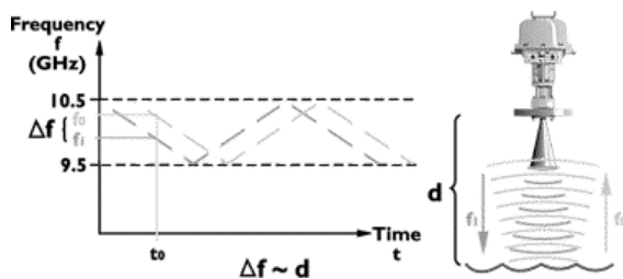
Abbildung 2-8: Meßprinzip des Radar – Wasserstandspegels – FMCW-Verfahren [C & G INDUSTRIAL SUPPLY, 1998]
