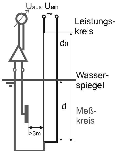
Abbildung 2-3: Meßprinzip von Drahtwellenpegeln (Verfahren B)
