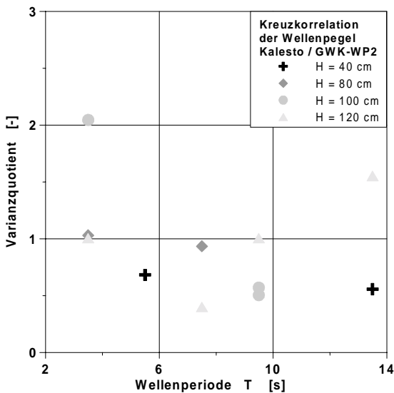
Abbildung 6-27: Abhängigkeit des Varianzverhältnisses zwischen den Zeitreihen der mit den Sensoren KALESTO und GWK-WP2 gemessenen Wasserspiegelauslenkung von Wellenperiode und -höhe bei regelmäßigem (links) unregelmäßigem Seegang (rechts)
