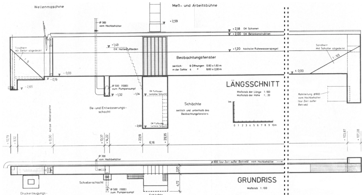
Abbildung 4-3: Position der Meßbühne im WELLENKANAL SCHNEIDERBERG WKS [nach GRÜNE, 1976]
