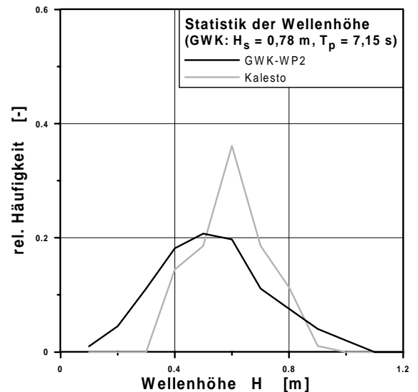
Abbildung 6-28: Statistik der Wellenhöhe im GWK bei regelmäßigem (links) und unregelmäßigem Seegang (rechts)
