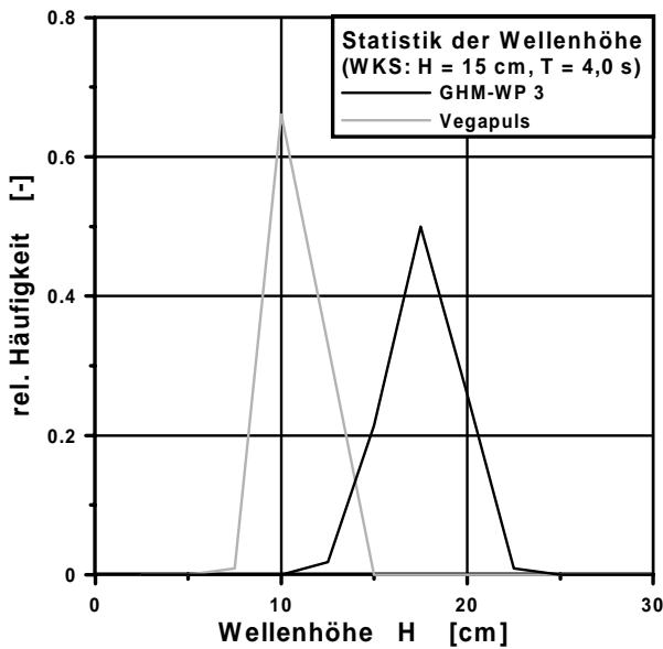
Abbildung 6-3: Statistik der Wellenhöhe im WKS bei regelmäßigem (links) und unregelmäßigem Seegang (rechts)
