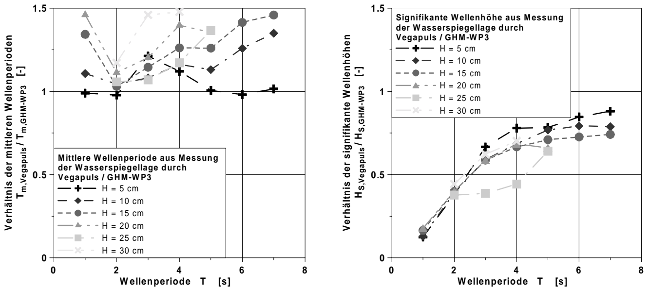
Abbildung 6-14: Verhältnis der aus Messungen von VEGAPULS und GHM-WP3 im WKS bestimmten mittleren Wellenperioden (links) und signifikanten Wellenhöhen (rechts) bei regelmäßigen Wellen
