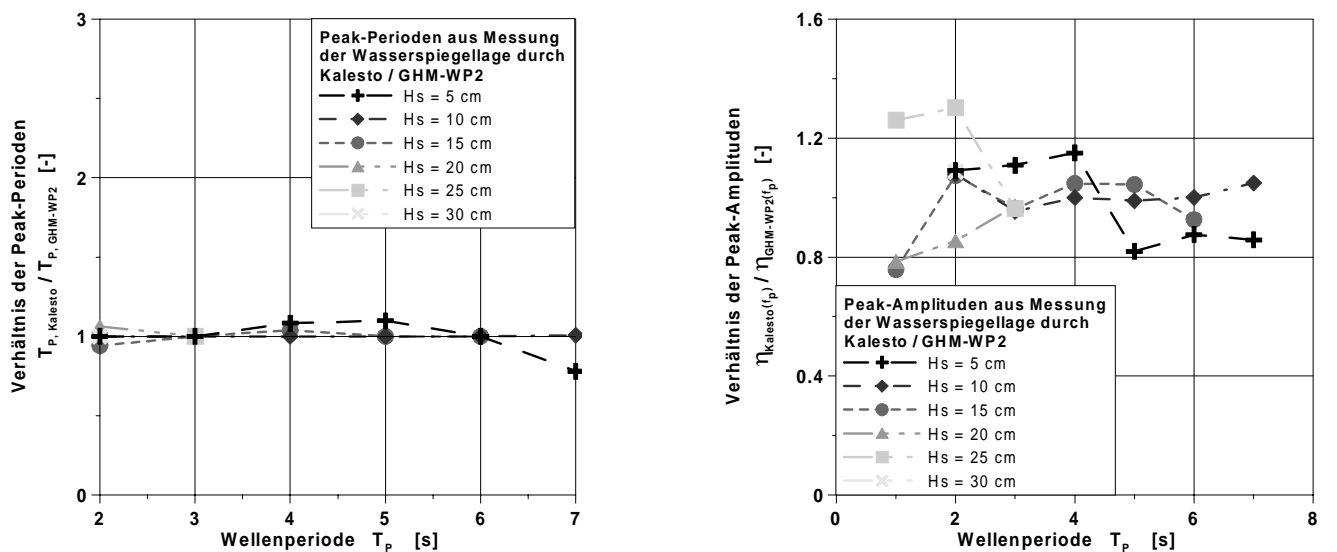
Abbildung 6-33: Verhältnis der aus Messungen von KALESTO und GHM-WP2 im WKS bestimmten Peak-Perioden (links) und Peak-Amplituden (rechts) bei unregelmäßigen Wellen
