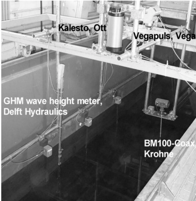
Abbildung 4-1: Instrumentierung des WELLENKANALS SCHNEIDERBERG WKS
