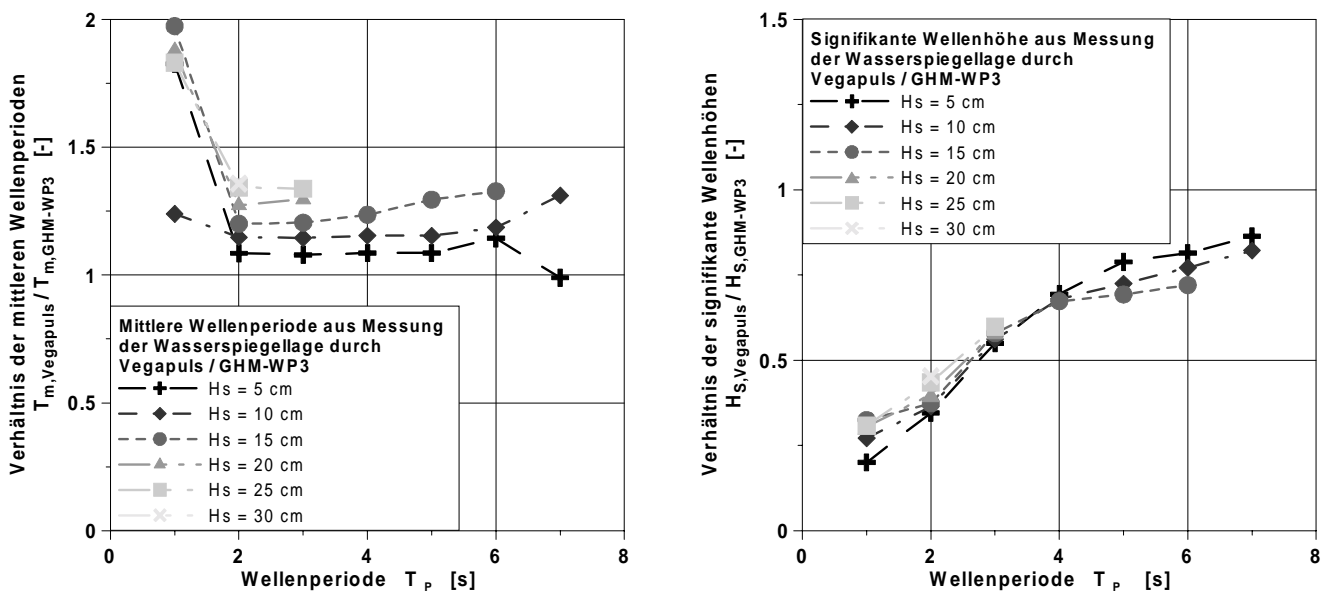
Abbildung 6-15: Verhältnis der aus Messungen von VEGAPULS und GHM-WP3 im WKS bestimmten mittleren Wellenperioden (links) und signifikanten Wellenhöhen (rechts) bei unregelmäßigen Wellen
