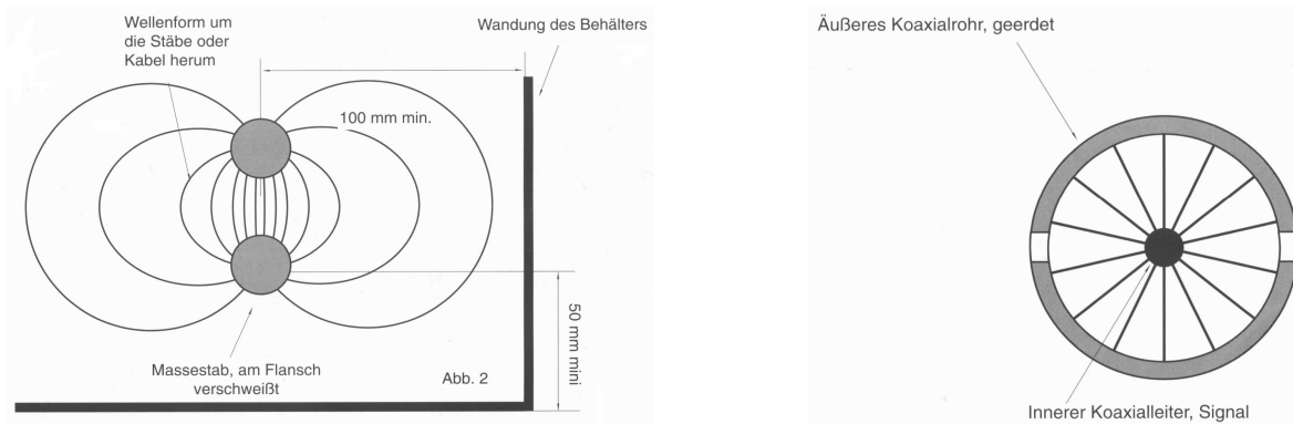
Abbildung 3-15: Feldlinien des elektrischen Feldes, links: BM100 Typ A, rechts: BM100 Typ C [KROHNE MEßTECHNIK GMBH & Co. KG, 1996]
