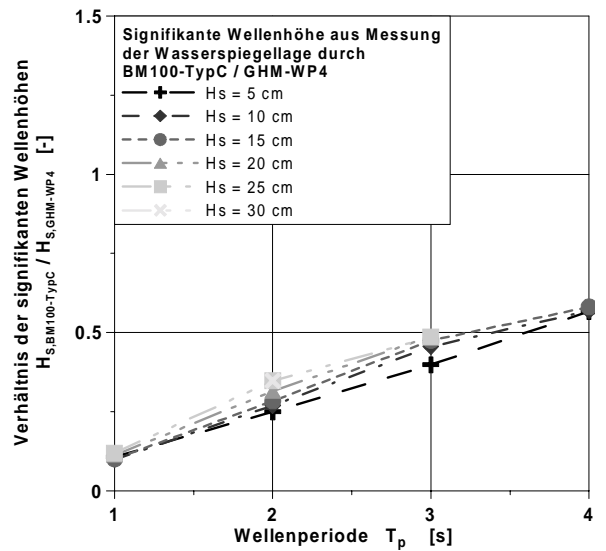
Abbildung 6-50: Verhältnis der aus Messungen von BM100-TYP C und GHM-WP4 im WKS bestimmten mittleren Wellenperioden (links) und signifikanten Wellenhöhen (rechts) bei unregelmäßigen Wellen
