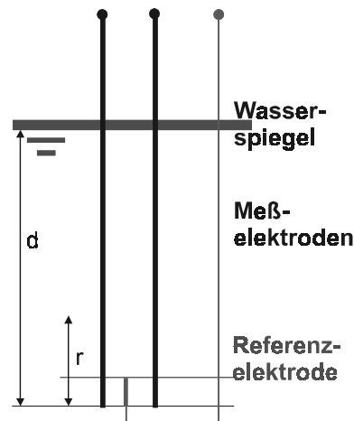
Abbildung 2-1: Meßprinzip von Drahtwellenpegeln (Verfahren A)
