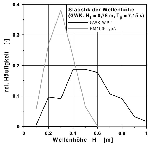
Abbildung 6-53: Statistik der Wellenhöhe bei regelmäßigem (links) und unregelmäßigem Seegang (rechts)
