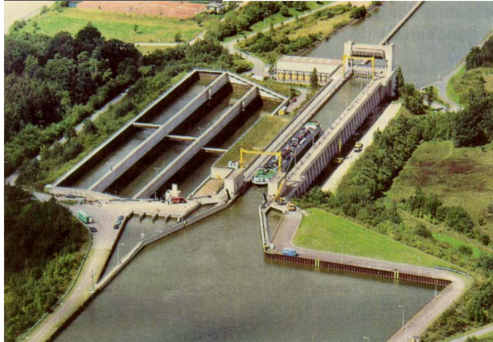
Schachtschleuse mit offenen Sparbecken
