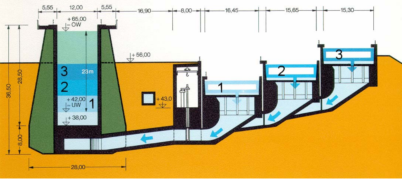
4 Füllen der Kammer (Bergschleusung)
