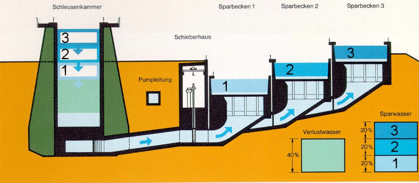
4 Füllen der Kammer (Bergschleusung)
