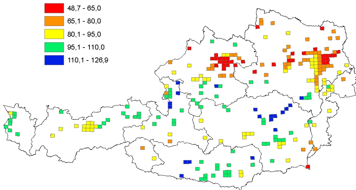
Abbildung 6 Räumliche Verteilung der empfohlenen Bemessungsregenspenden für r_{90,10} nach BMfLFUW (2006)
