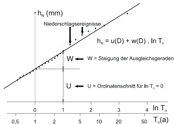
Abbildung 1 Ermittlung der ortsabhängigen Parameter u(D) und w(D) nach BMfLFUW (2006)
