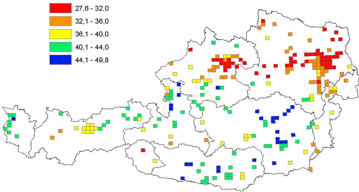
Abbildung 5 Räumliche Verteilung der empfohlenen Bemessungsregenspenden für r_{90,1} nach BMFLFUW (2006)
