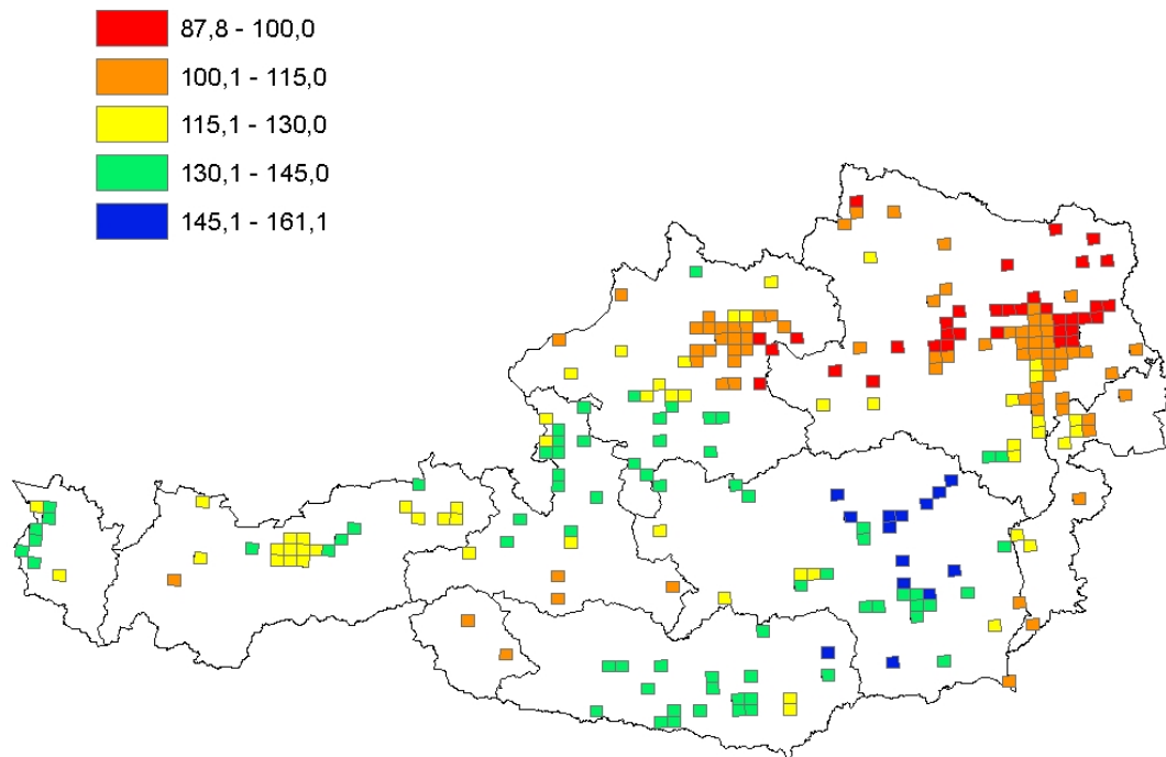
Abbildung 3 Räumliche Verteilung der empfohlenen Bemessungsregenspenden für den r_{15,1} nach BMfLFUW (2006)
