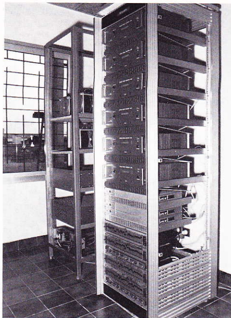
In einem eigenen Raum sind alle STUDER-Leistungsverstärker in einem Rack zusammengefasst.
