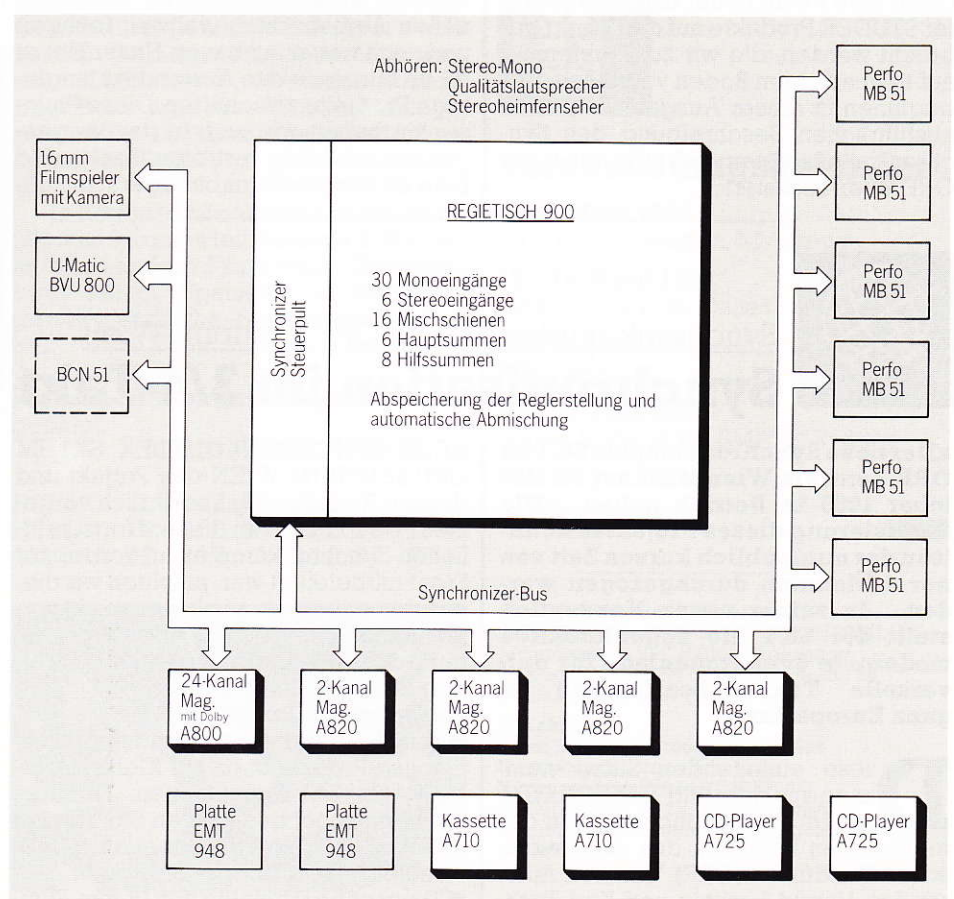
Blockdarstellung des Regieplatzes SK 1.
