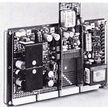
Mutterprint (EUROPA-Karte) mit vier Subprints.
