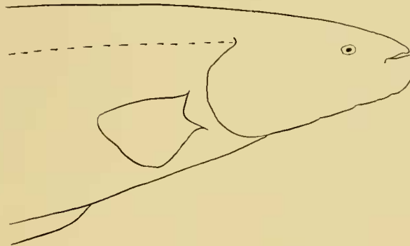
FIG. 2. Gymnotus carapo Linnæus.
