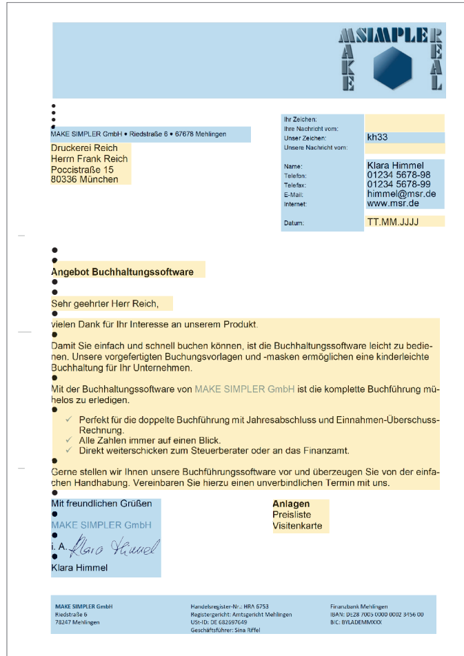
1 Geschäftsbrief
