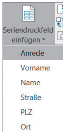
1 Seriendruckfeld einfügen
