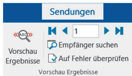
2 Vorschau wählen
