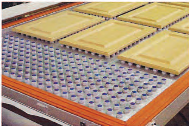
Magnetic Pin System Sistema magnético de pernos Système à broches magnétiques Magnetisches Pinsystem
