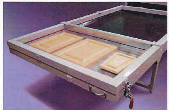
Tray Minimizer with rubber sheet Charola minimizadora con hoja de caucho Réducteur de plateau avec feuille de caoutchouc Separator zum Unterteilen des Tisches
