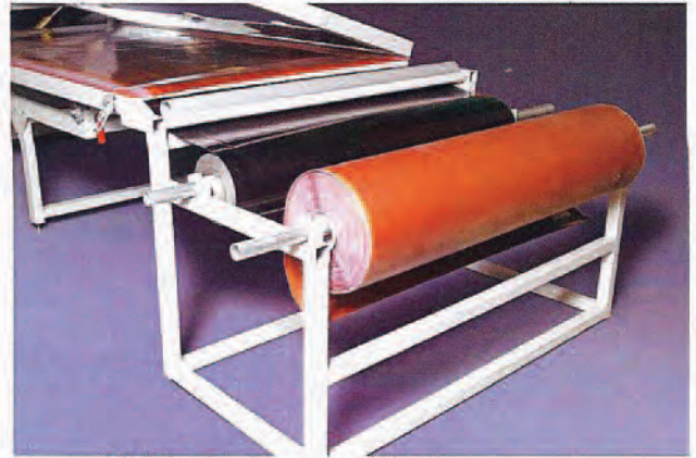
Thermofoil Stand Rack para rollos de vinyl Banc Thermofoil Vorrichtung für die Folientnahme und Lagerung
