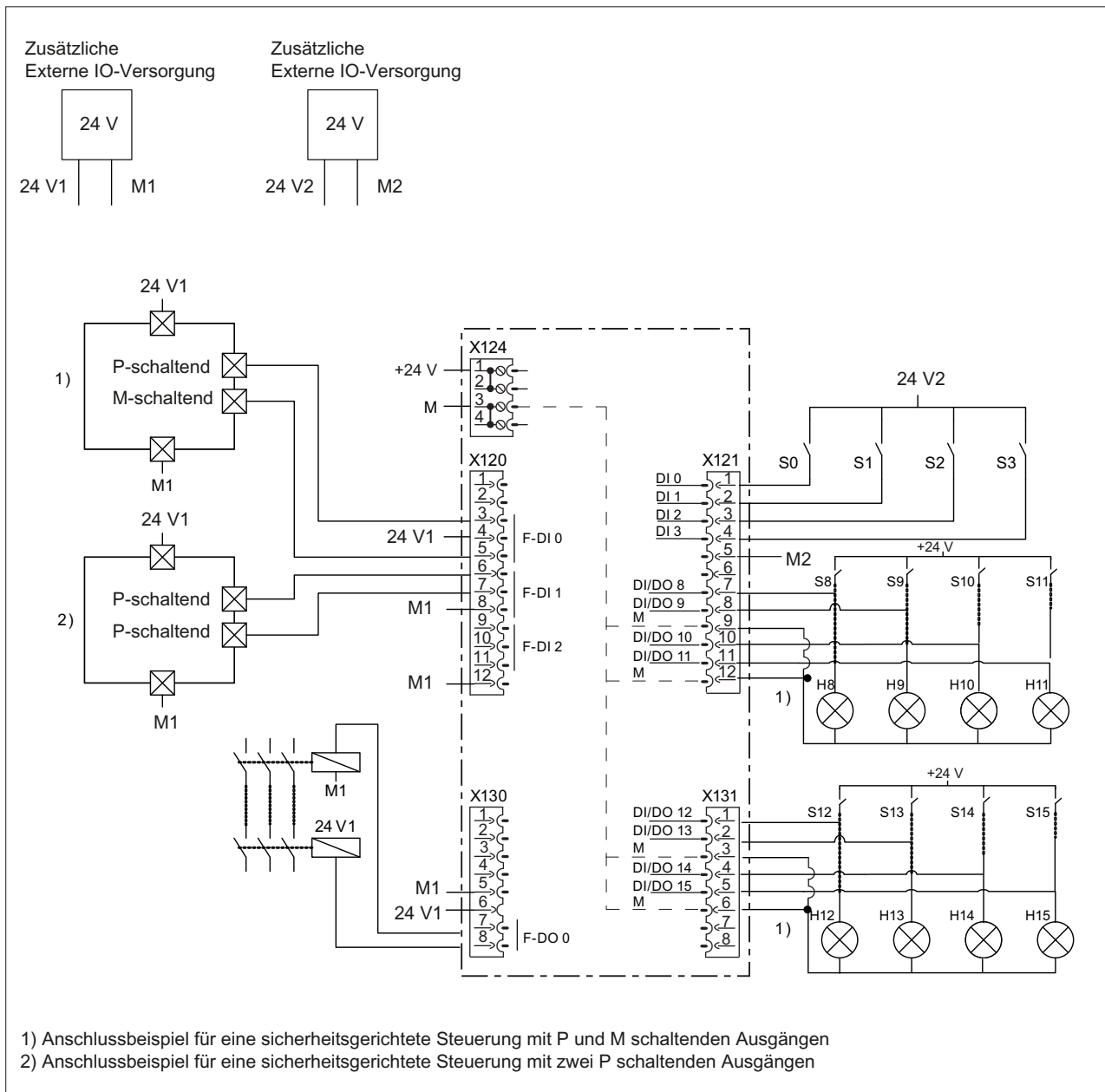
Bild 4-9 Beschriftungsbeispiel der F-DI und F-DO mit Safety Integrated Extended und Advanced Functions
