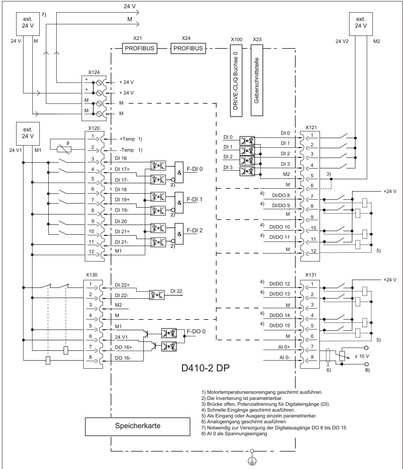
Bild 4-4 Anschlussbeispiel SIMOTION D410-2 DP mit Safety Integrated Extended und Advanced Functions
