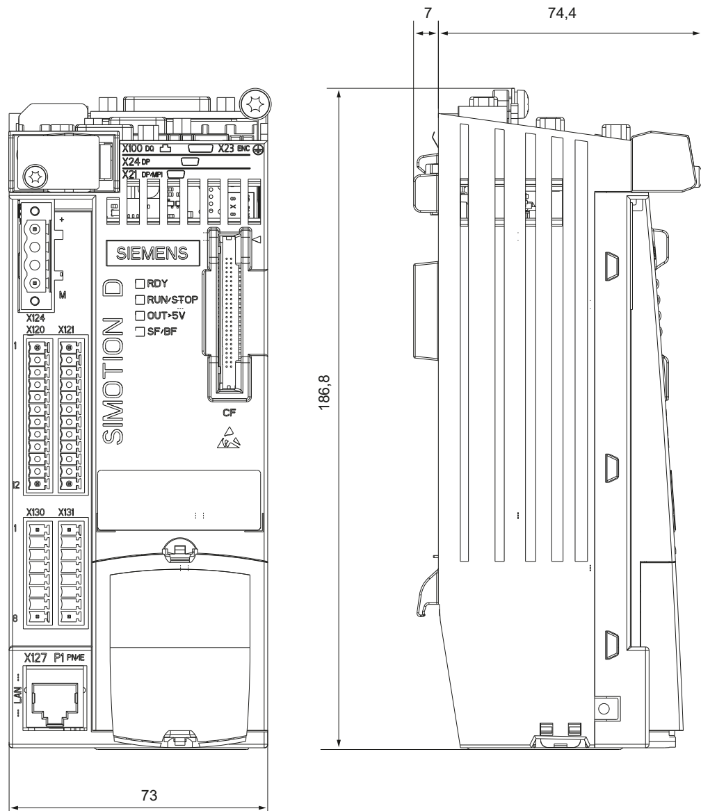
Bild 6-1 Maßbild SIMOTION D410-2 DP (Angaben in mm)
