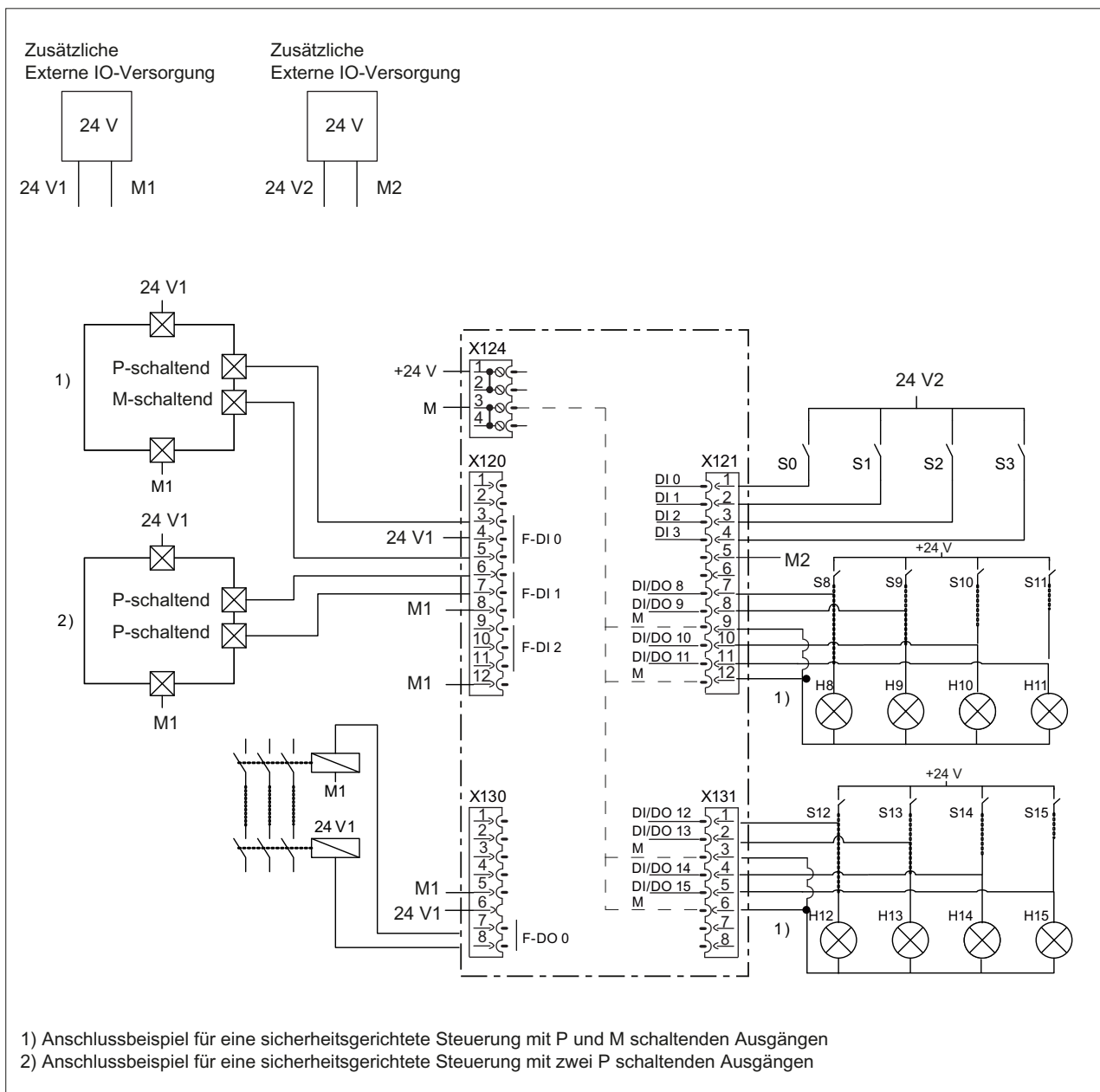
Bild 4-5 Beschriftungsbeispiel der F-DI und F-DO mit Safety Integrated Extended und Advanced Functions
