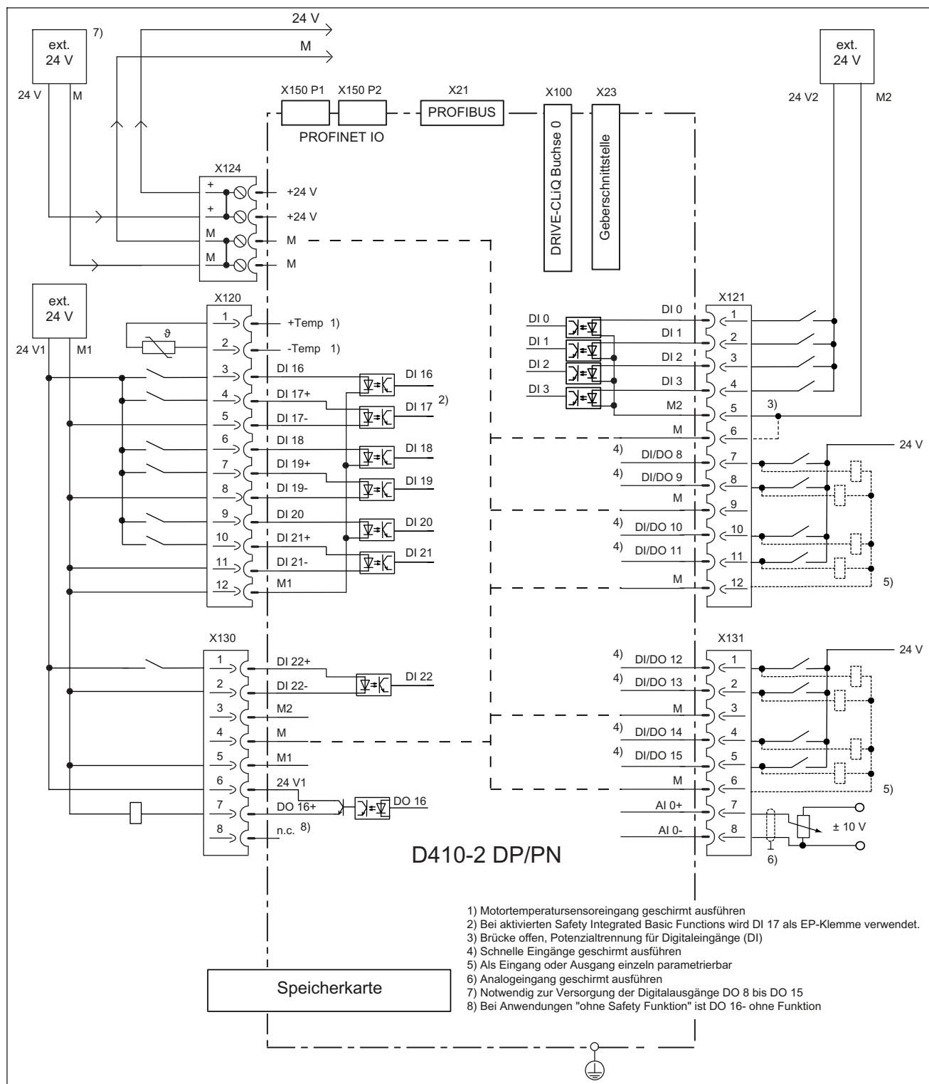
Bild 4-7 Anschlussbeispiel SIMOTION D410-2 DP/PN ohne Safety Integrated Extended und Advanced Functions
