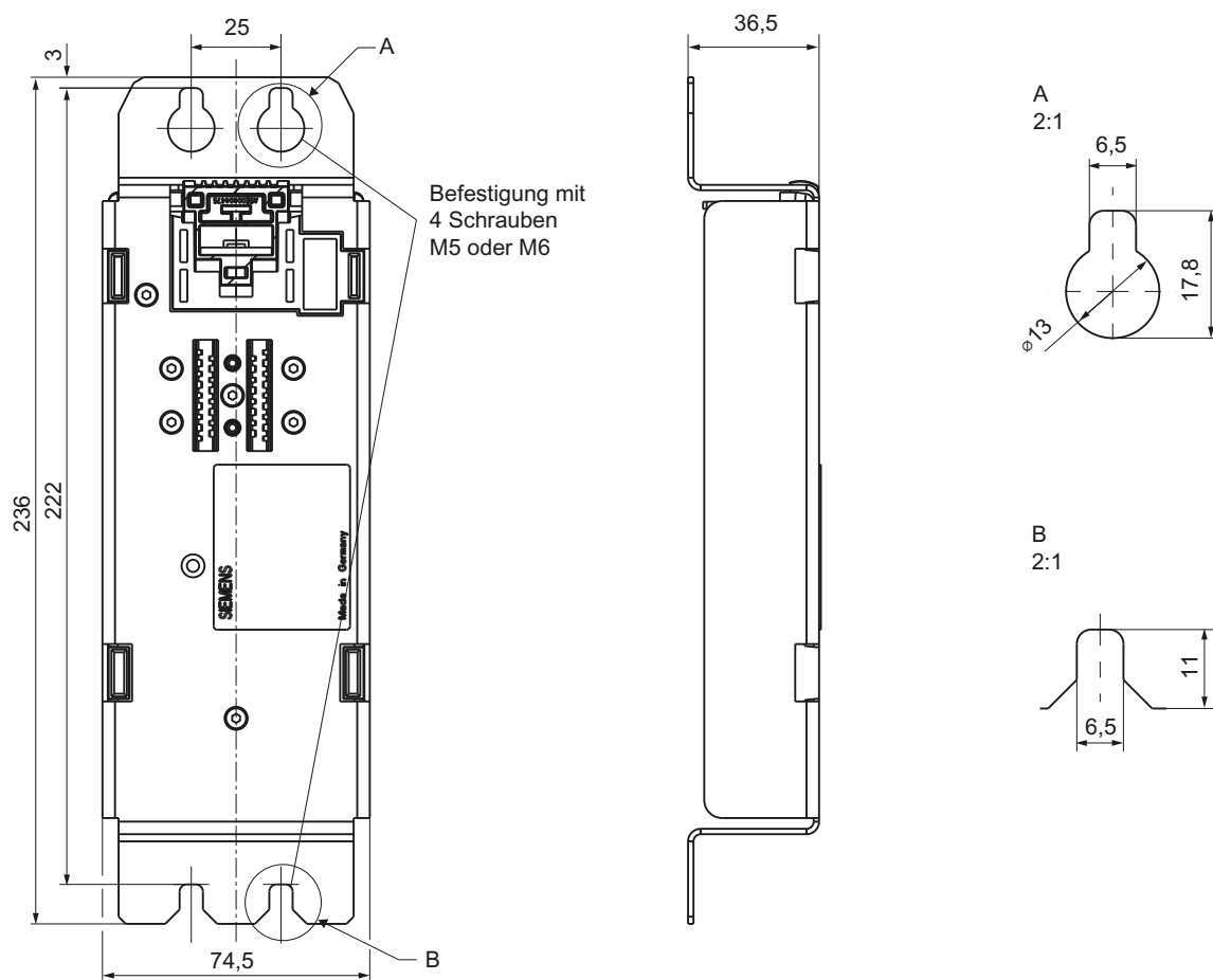
Bild 6-3 Maßbild Montageplatte (Angaben in mm)
