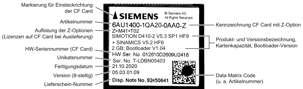
Bild 2-10 CompactFlash Card (Beispiel für 2 GB CF Card)
