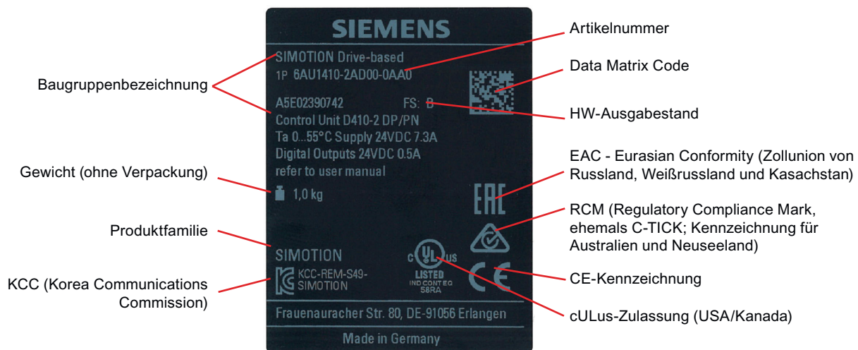
Bild 2-8 Typenschild am Beispiel von SIMOTION D410-2 DP/PN
