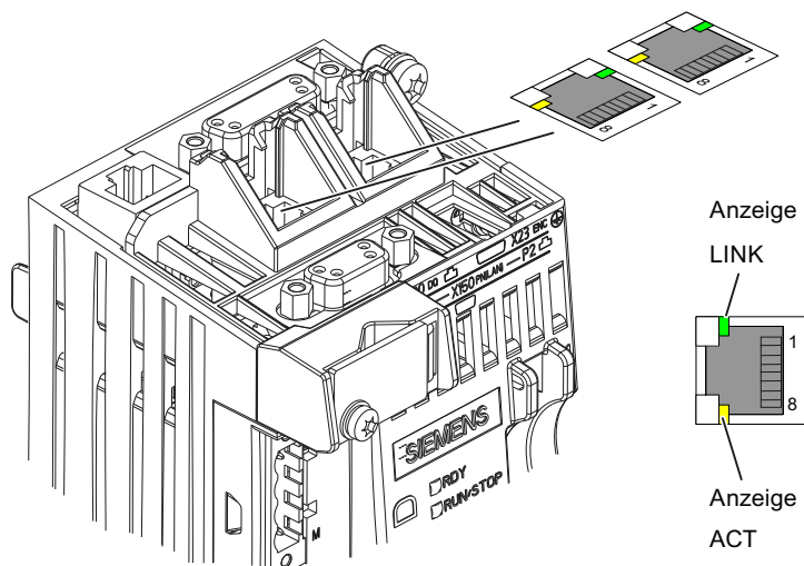
Bild 4-1 PROFINET-Ports der D410-2 DP/IPN
