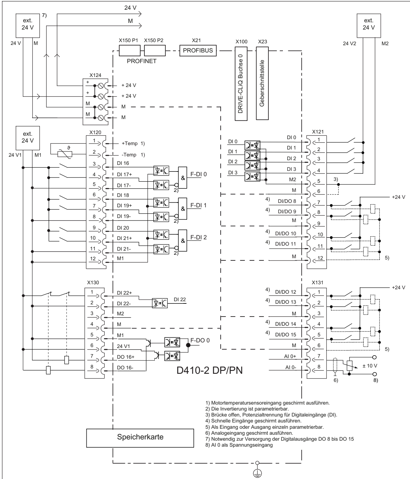
Bild 4-8 Anschlussbeispiel SIMOTION D410-2 DP/PN mit Safety Integrated Extended und Advanced Functions
