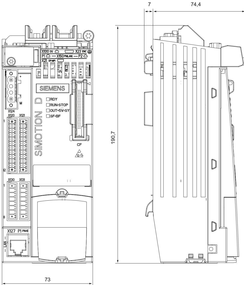
Bild 6-2 Maßbild SIMOTION D410-2 DP/PN (Angaben in mm)
