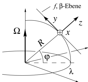
Figur 6.1: Lokales kartesisches Koordinatensystem auf rotierender Kugel und Bezeichnungen
