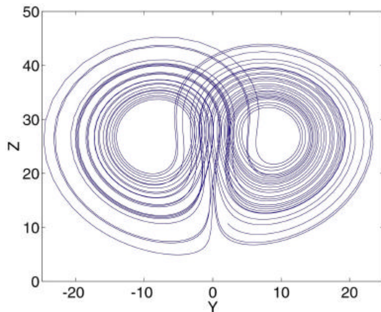
Figur 7.9b: Schnitte durch die verschiedenen Ebenen im (X, Y, Z) -Raum. (Y, Z) Ebene des Lorenz-Saltzman Modells mit den klassischen Parameterwerten.
