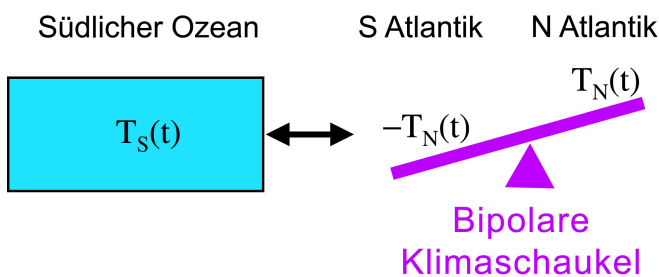
Figur 9.2: Bipolare Klimaschaukel gekoppelt mit einem südlichen Wärme reservoir. (Figur nach Stocker & Johnsen, 2003)
