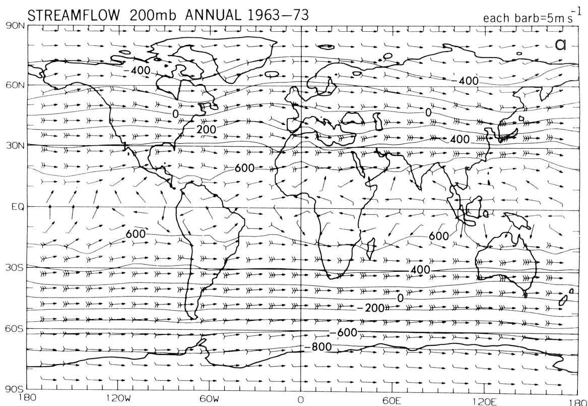
Figur 7.1: Mittlerer Wind auf ca. 12 km Höhe. (Figur aus Peixoto & Oort, 1982).
