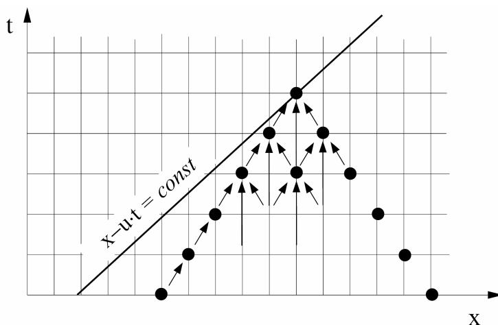
Figur 3.8: Abhängigkeitsgebiet des Schemas CTCS (3.14) und Charakteristik, die ausserhalb liegt, und somit das CFL-Kriterium verletzt.
