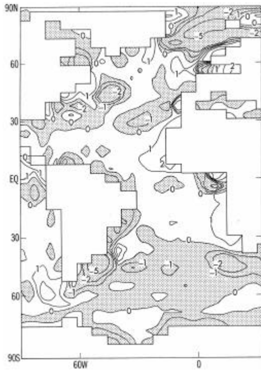
Figur 8.12: Korrektur des Wasserflusses in m 3 /Jahr. Besonders in Bereichen starker Ozeanströmungen (Golfstrom), sowie in Gebieten der Tiefenwasserbildung (Norwegisches und Weddell Meer), wie auch an Osträndern treten sehr hohe Flüsse auf. (Figur aus Manabe & Stouffer, 1988, J. Climate 9, 841.).
