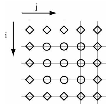
Figur 5.1: Gitter mit inneren Punkten und Randpunkten
