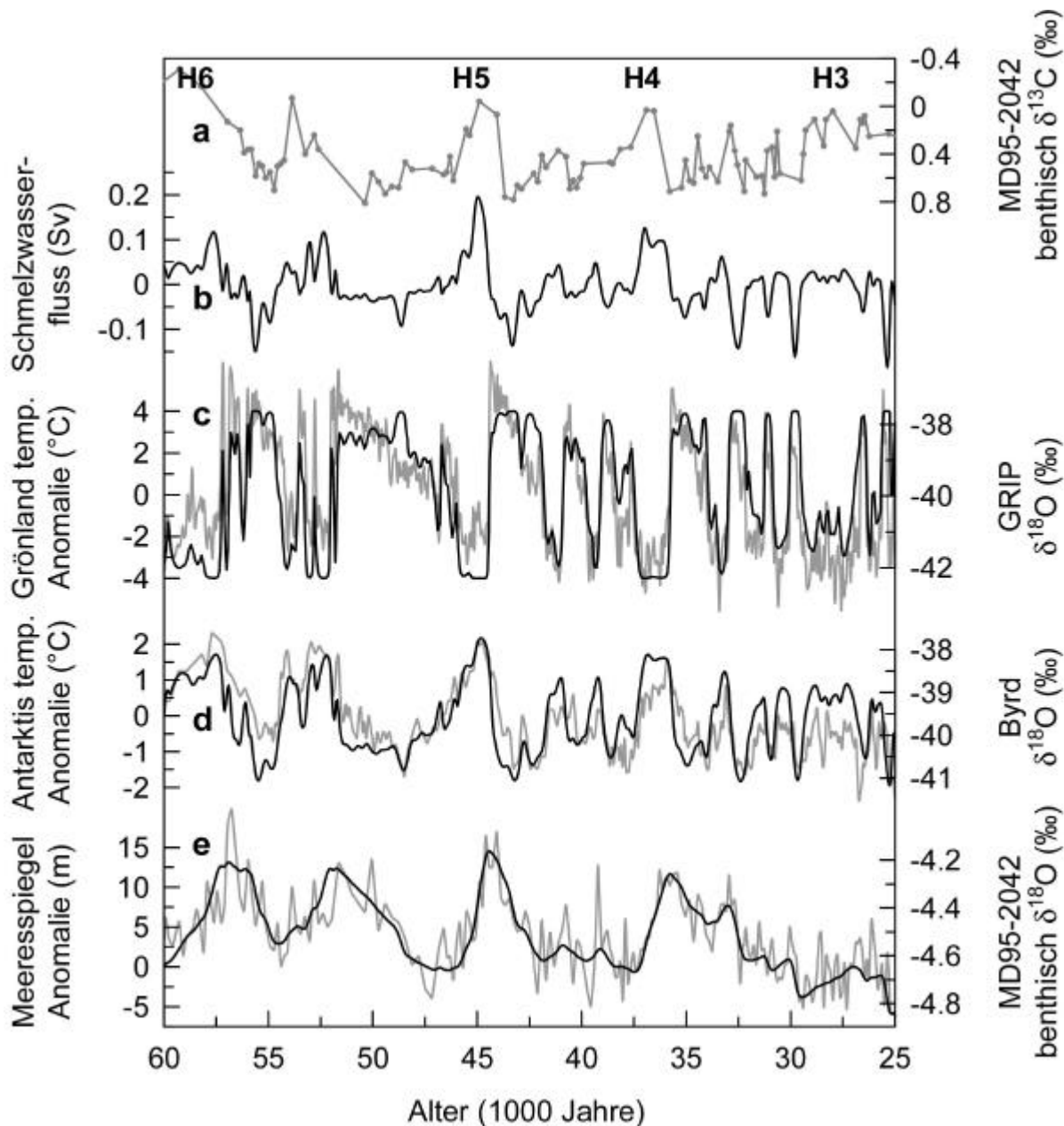
Figur 9.4: Variabilität der Grönland (c) und Antarktis (d) Temperatur aus Eisbohrkernen, und aus Proxydaten aus einemhochauflösenden Tiefseesedimentkern vor Portugal (e, Shackleton et al., 2000, Paleoceanography 15, 565). Gemessene Daten sind in Grau gegeben, nach (9.3) modellierte Daten mit Input der Grönlandtemperatur sind die schwarzen Kurven. Der Schmelzwasserfluss (b) wird durch Optimierung der Übereinstimmung der grauen und schwarzen Kurven in (c) bis (e) erhalten. Die Übereinstimmung von (a) und (b) ist ein unabhängiger Test der Gültigkeit von Gleichung (9.3). (Figur aus Knutti et al., 2004).
