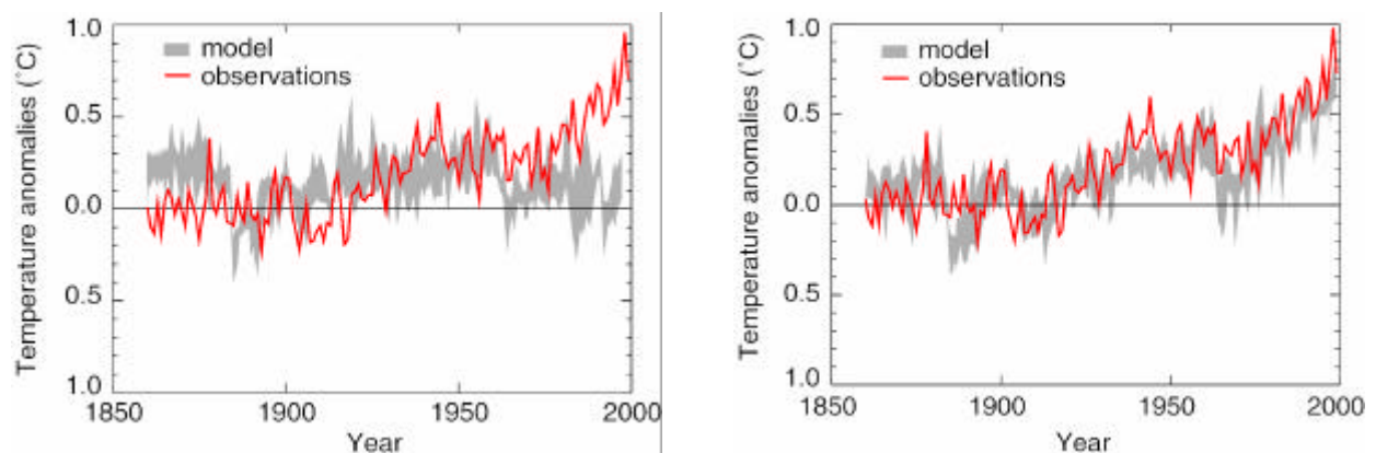
Figur 1.12: Global gemittelte Entwicklung der Temperatur seit 1850 basierend auf instrumentell gemessenen Beobachtungen (dicke Linie) und vier Ensemble Simulationen mit dem gekoppelten Klimamodell des Hadley Centres (graues Band). Links: Simulationen mit konstantem CO_2 und Aerosolen, beobachteten Vulkanausbrüchen und variable solare Strahlung. Rechts: zusätzlich vorgeschriebene atmosphärische CO_2 Konzentrationen und Sulfataerosole.
