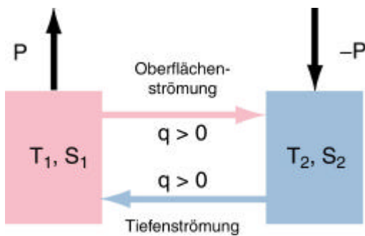
Figur 9.6: 2-Box Modell der thermohalinen Zirkulation. (Nach Stommel, 1961 und Marotzke, 2000).
