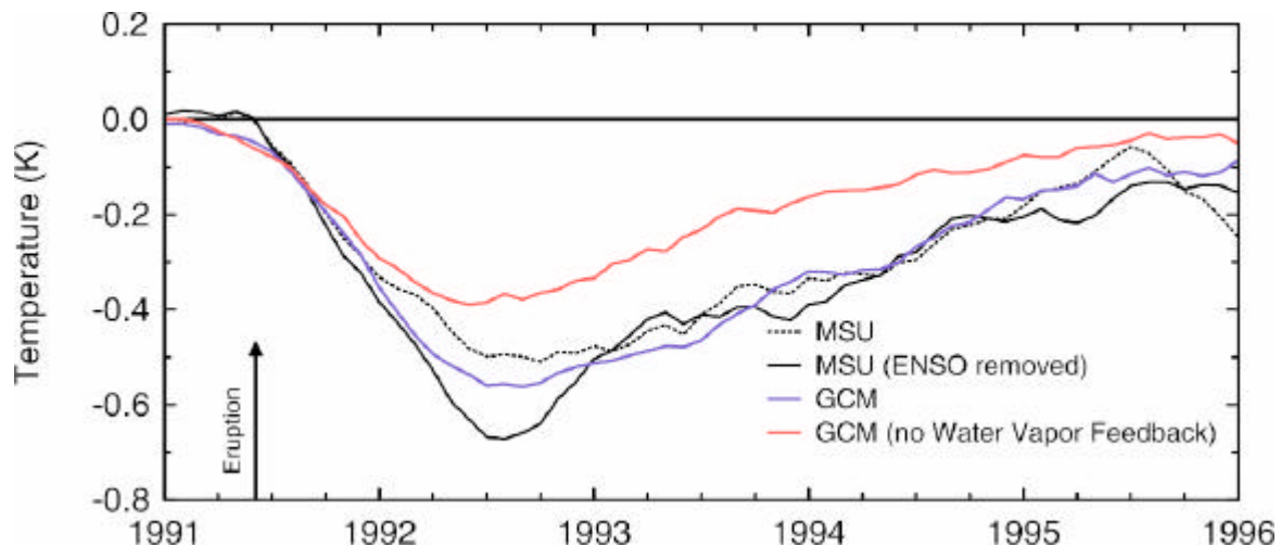
Figur 2.12: Global gemittelte Temperaturabweichung in der mittleren Troposphäre nach der Eruption von Mount Pinatubo 1991. Eine globale Abkühlung von 0.7^{\circ}\text{C} wurde anhand von Strahlungsmessungen von Satelliten (microwave sounding unit, MSU) beobachtet, nachdem ein erwärmender Effekt des 1992/93 ENSO abgezogen wurde. Ein Klimamodell, in dem der Wasserdampf-feedback abgestellt ist, zeigt eine geringere Abkühlung. (Soden et al., 2002, Science 296, 797).
