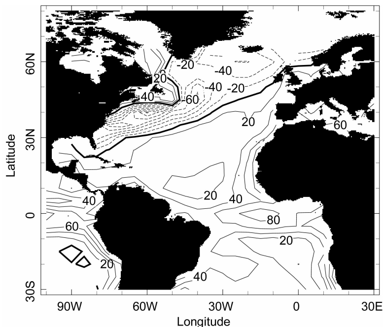
Figur 8.3: Wärmeflüsse -F(O \rightarrow A) im Atlantikbereich in \text{Wm}^2 . Die Karte wurde auf dem Internet generiert ( http://ingrid.ldeo.columbia.edu ), wo viele Datensätze zugänglich sind (Cayan Datensatz).
