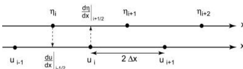
Figur 6.3b: Versetztes Gitter für die Flachwassergleichungen. Flussgrössen ( u ) und Volumengrössen ( \eta ) werden an unterschiedlichen Stellen ausgewertet (staggered grid).
