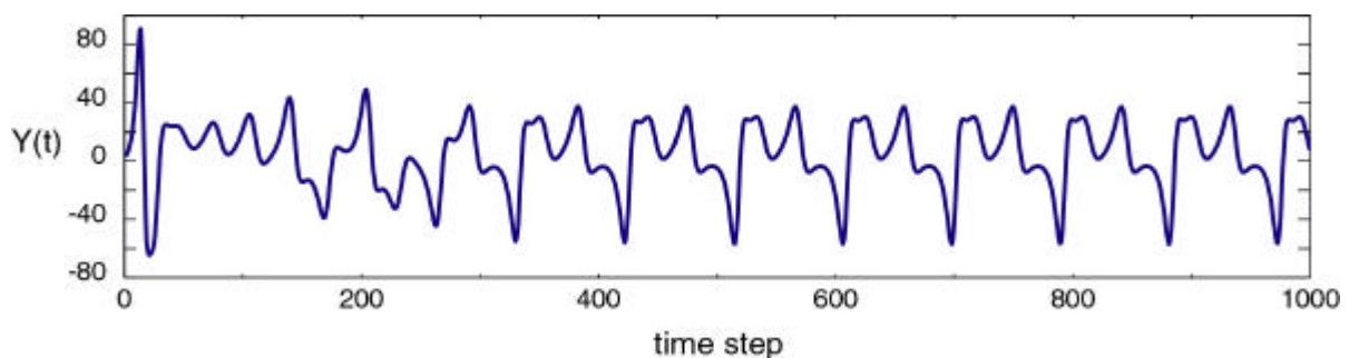
Figur 7.11: Wie Figur 7.8 aber mit r = 100 , s = 10 , b = 8/3 .
