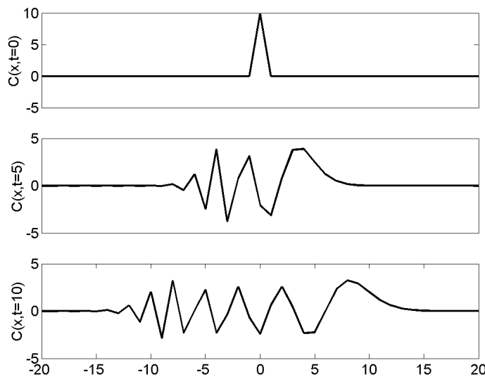
Figur 3.7: Auseinanderlaufen eines Wellenpakets und Erzeugung des numerischen Modes bei der Lösung der Advektionsgleichung mit CTCS.
