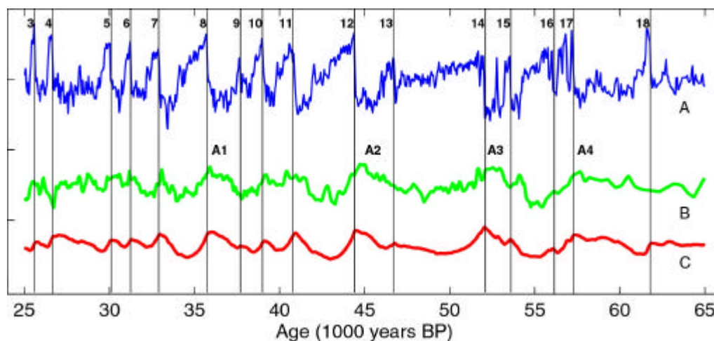
Figur 9.3: Hochpassgefilterte Zeitreihen der Temperaturen in Grönland (A) und der Antarktis (B) aus Eisbohrkernen, und (C), simulierte Temperaturen gemäss (9.2) mit Input (A). Die Stadiale in der Antarktis (A1, A2, ...) sind somit eine Manifestierung der abrupten Dansgaard/Oeschger Ereignisse im Norden. (Figur aus Stocker & Johnsen, 2003).
