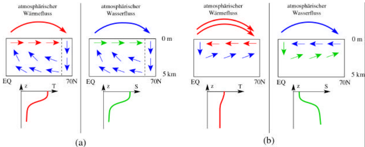
Figur 9.8: Schematische Darstellung der thermohalinen Strömung und der meridionalen Wärme- und Wasserflüsse. (a) Direkte Zirkulation: Wasser sinkt, wo es kalt ist; (b) indirekte Zirkulation: Wasser sinkt in warmen Gebieten.
