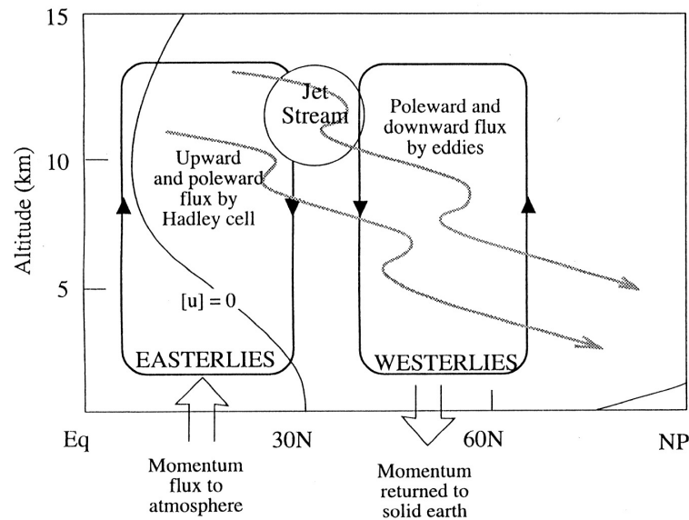
Figur 7.3: Schematische Darstellung des meridionalen Flusses von Drehimpuls von der Erdoberfläche via die Atmosphäre zurück an die Erde. (Figur aus Hartmann 1992).
