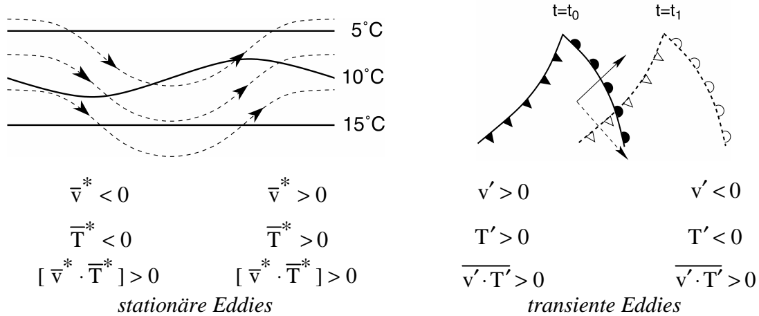
Figur 4.3: Schematische Darstellung von stationären und transienten Eddies in der Atmosphäre. In der dargestellten Situation transportieren beide Systeme Wärme nordwärts.
