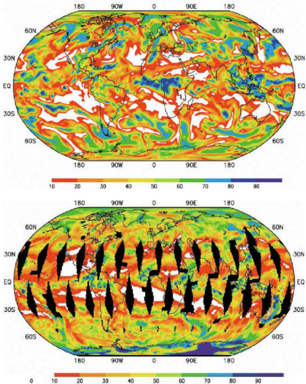
Figur 2.3: Vergleich der Leistung moderner Klimamodelle anhand des atmosphärischen Wasserdampfgehaltes auf 400 mb (ca. 7 km) angegeben als relative Feuchte (in %) an einem Tag im Mai. Links: Modellsimulation mit dem Modell des MPI Hamburg in höchster Auflösung (T106, M. Wild, ETHZ). Rechts: Mittlere relative Feuchte im Bereich 250 bis 600 mb aus Satellitendaten (SSM/T-2) berechnet, wobei Unsicherheiten ausserhalb 30°S und N grösser sind. Trockene Gebiete sind als weisse Flächen erkennbar. Figur von IPCC 2001, Kapitel 7.
