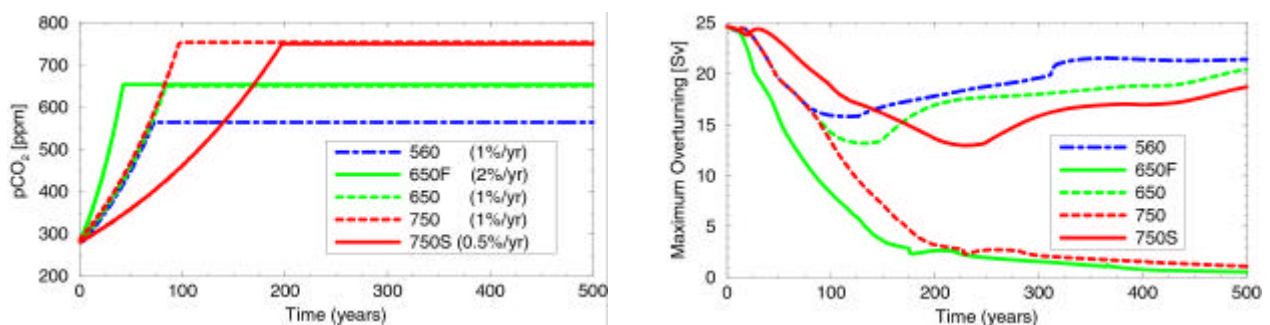
Figur 9.10: Simulationen mit dem Bern 2.5d Modell zur Entwicklung der thermohalinen Zirkulation im Atlantik bei einer Erwärmung. Die verschiedenen vereinfachten CO 2 -Szenarien (links) bestehen aus einem exponentiellen Anstieg unterschiedlicher Geschwindigkeit bis zu einem vorgegebenen Maximalwert. Die thermohaline Zirkulation (rechts) weist eine Bifurkation im Verhalten auf: für kleine Maximalwerte oder langsame Anstiegsraten wird die Schwelle eines vollständigen Abstellens nicht überschritten. (Figur von Stocker & Schmittner, 1997, Nature 388, 862)
