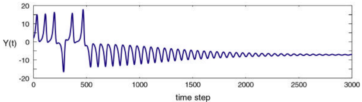
Figur 7.10: Wie Figur 7.8 aber mit r = 20 , s = 10 , b = 8/3 .
