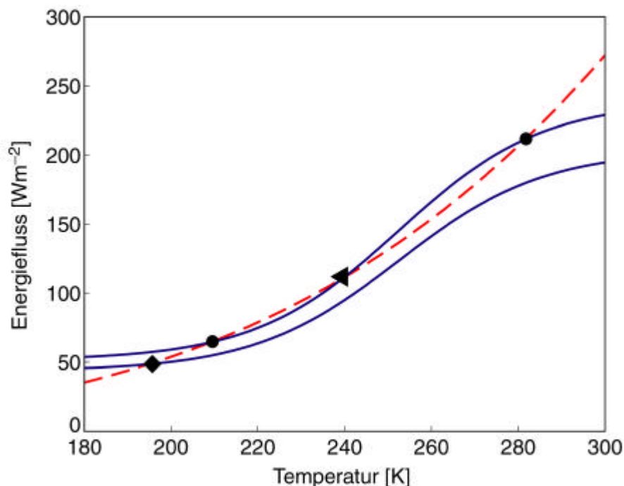
Figur 9.5: Rechte (gestrichelt) und linke Seite von (9.4) für S (obere Kurve) und 0.85 S . Die Temperaturabhängigkeit der Albedo ermöglicht mehrere Gleichgewichtslösungen: stabile (Punkte und Rhombus) und instabile (Dreieck).
