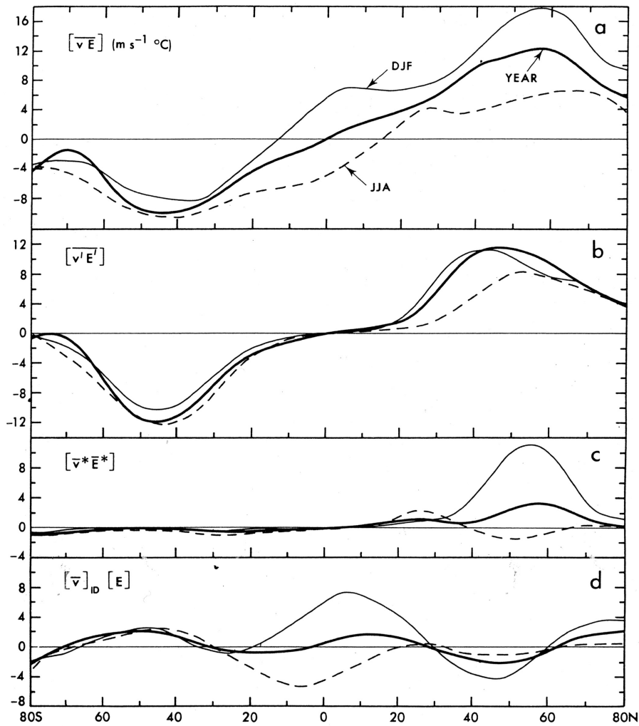
Figur 4.4: Profile der zonal und vertikal gemittelten meridionalen Transporte der gesamten Energie (4.1) in ^{\circ}\text{C m s}^{-1} . (a) total; (b) transiente Eddies; (c) stationäre Eddies; (d) mittlere meridionale Strömung, für das Jahresmittel, Winter- und Sommermonate. Um Einheiten PW zu erhalten, muss mit dem Faktor (2\pi R \cos\phi)c_p(p_0/g) multipliziert werden. (Figur aus Peixoto & Oort, 1992).
