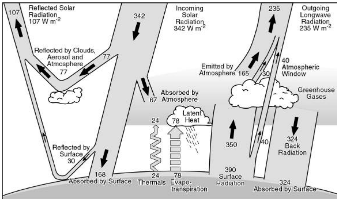
Figur 1.2: Globale Energieflüsse aus verschiedenen Quellen, die die Strahlungsbilanz der Erde beeinflussen. (Figur von IPCC, 2001).
