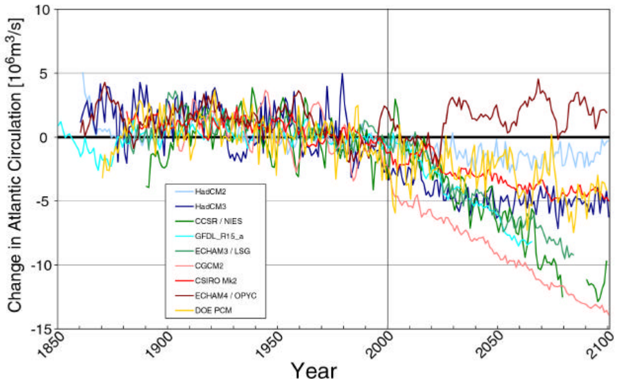
Figur 9.9: Veränderung der thermohalinen Zirkulation in 9 gekoppelten Klimamodellen für ein einfaches Erwärmungsszenario in den nächsten 100 Jahren. Viele Modelle zeigen eine Abschwächung, doch ist die Unsicherheit recht gross. (Figur aus IPCC, 2001).
