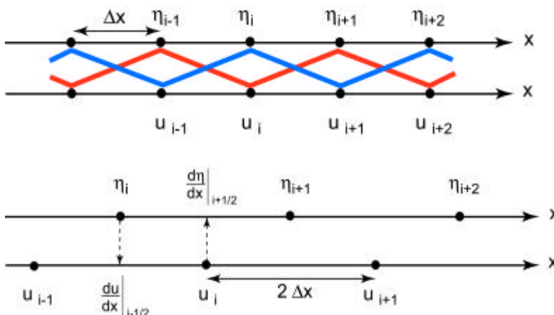
Figur 6.3a: Einfaches Gitter für die Flachwassergleichungen. Alle Funktionen werden an denselben Stellen ausgewertet. Es entstehen zwei unabhängige Untergitter, die mit den Linien verbunden sind.
