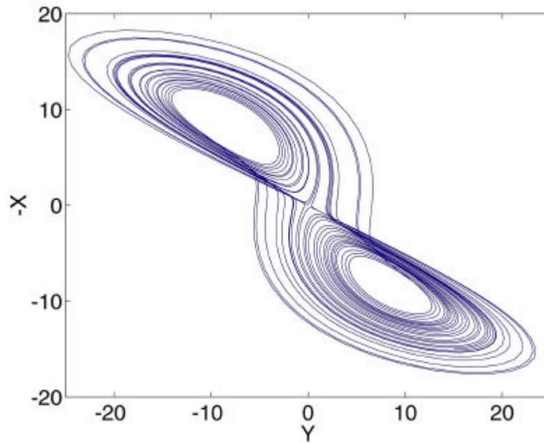
Figur 7.9c: Schnitte durch die verschiedenen Ebenen im (X,Y,Z)-Raum. (Y,-X ) Ebene des Lorenz-Saltzman Modells mit den klassischen Parameterwerten.
