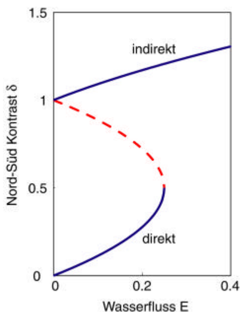
Figur 9.7: Multiple Gleichgewichte (instabil = gestrichelt) der thermohalinen Zirkulation für verschiedene Werte des Wasserflusses im Stommel Box Modell.
