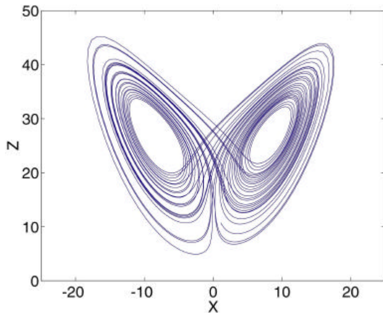
Figur 7.9a: Schnitte durch die verschiedenen Ebenen im (X, Y, Z) -Raum. (X, Z) Ebene des Lorenz-Saltzman Modells mit den klassischen Parameterwerten.
