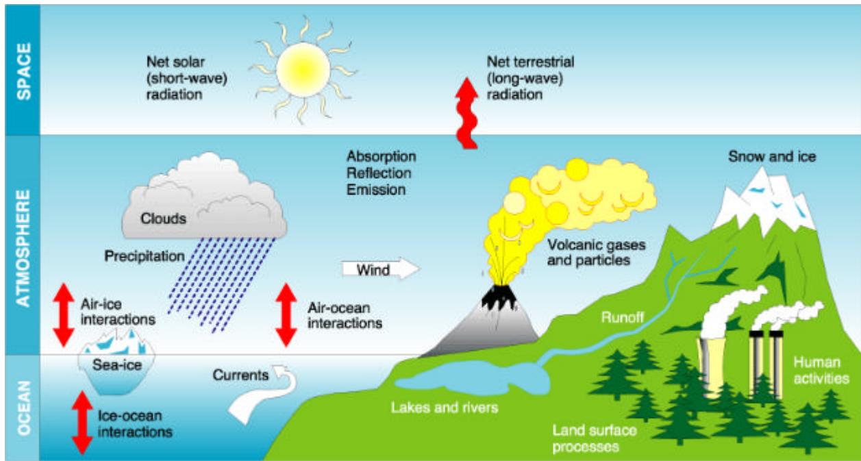
Figur 1.1: Die wichtigsten Komponenten des Klimasystems auf globaler Skala (Figur von IPCC, 2001).
