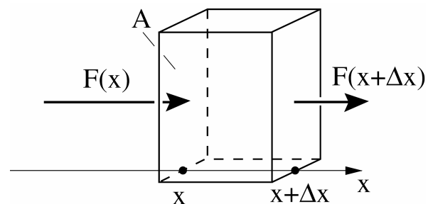
Figur 3.3: Ortsabhängiger Fluss in einer Dimension
