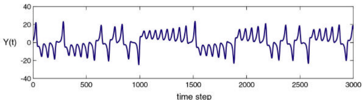
Figur 7.8: Erste 3000 Zeitschritte der Zeitreihe Y(t) des Lorenz-Saltzman Modells mit den klassischen Parameterwerten r = 28 , s = 10 , b = 8/3 und \tau = 0.012 , integriert mit dem Runge-Kutta Verfahren.
