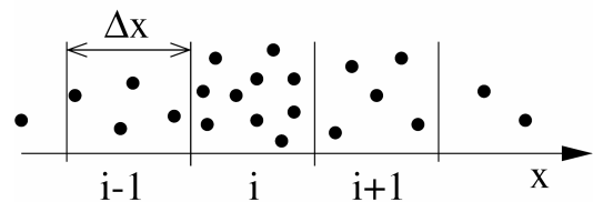
Figur 3.2: Modell der 1-dimensionalen Diffusion
