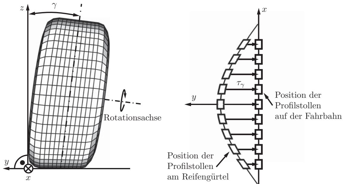
Bild 2.3: Links: Abgebildet ist ein frei rollendes Rad, welches unter einem Sturzwinkel \gamma abrollt. Der Sturzwinkel ist durch den Winkel zwischen der Reifensymmetrieachse und der Fahrtrichtung definiert.
