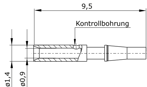
Hauptabmessungen Kontaktbuchse
