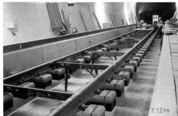
Feste Fahrbahn im Einbau im Lötschberg-Basistunnel (Bild: Rhombergbau).
