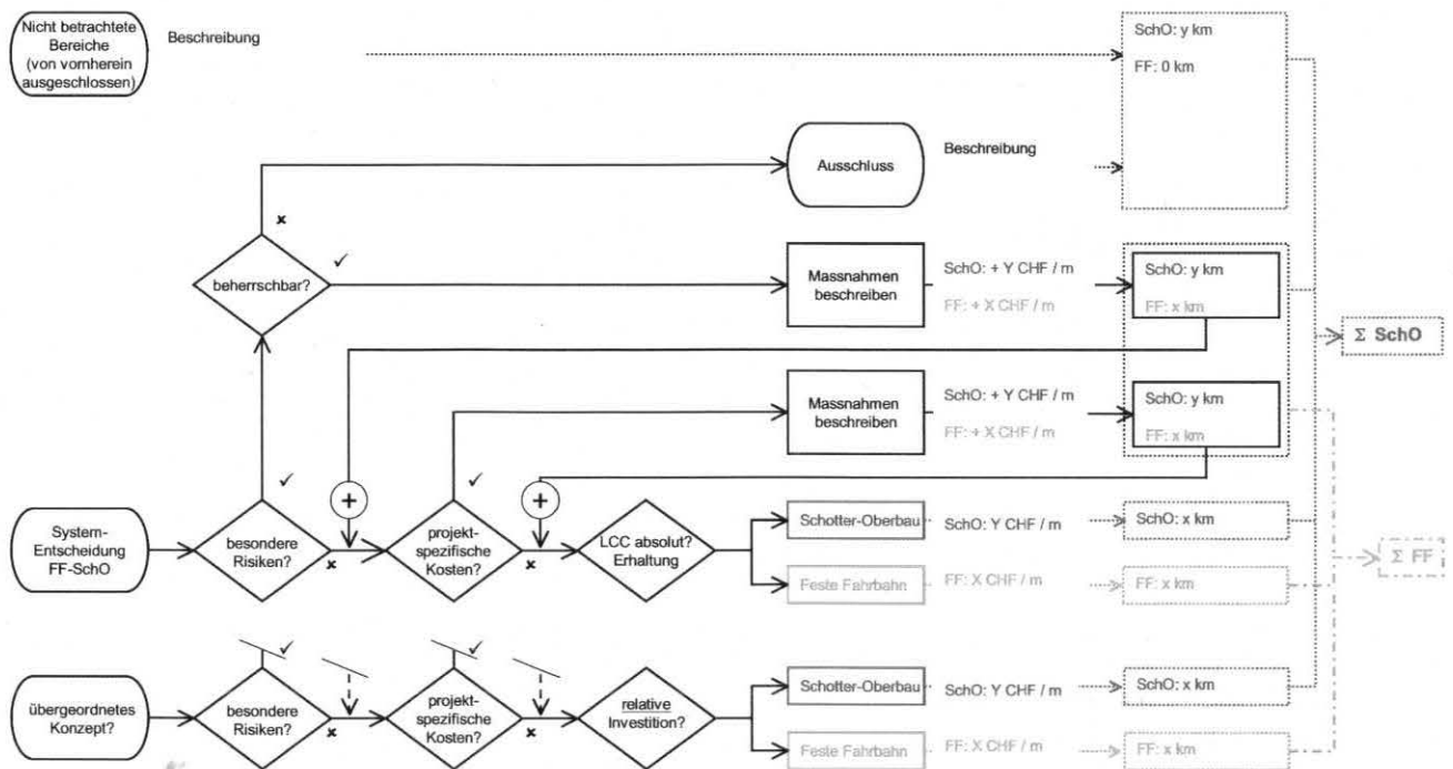
1 Entscheidungsbaum Feste Fahrbahn versus Schotteroberbau der SBB-Fahrbahnstrategie (Bild: Rolf Steinegger / SBB)
