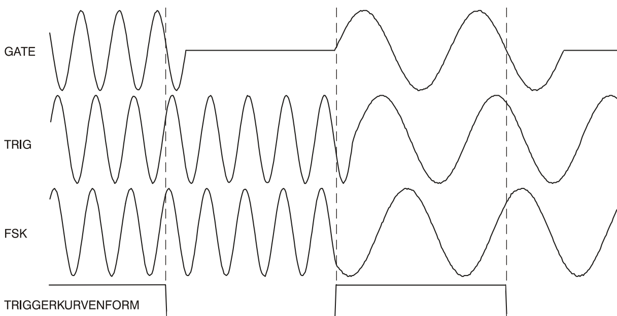
Tonkurvenformtypen
