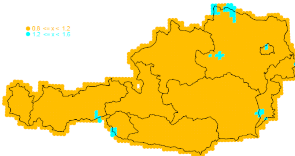
Abbildung 21. Quotient des Bemessungsniederschlags 2020 zu den Werten 2009. D: 15 Minuten, T: 10
