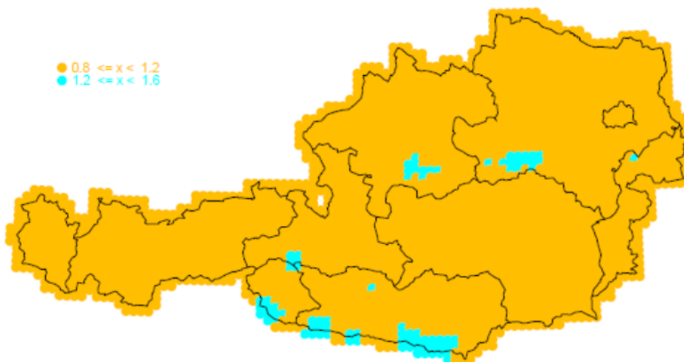
Abbildung 17. Quotient der interpolierten ÖKOSTRA-Auswertungen 2020 zu 2009. D: 12 Stunden, T: 1
