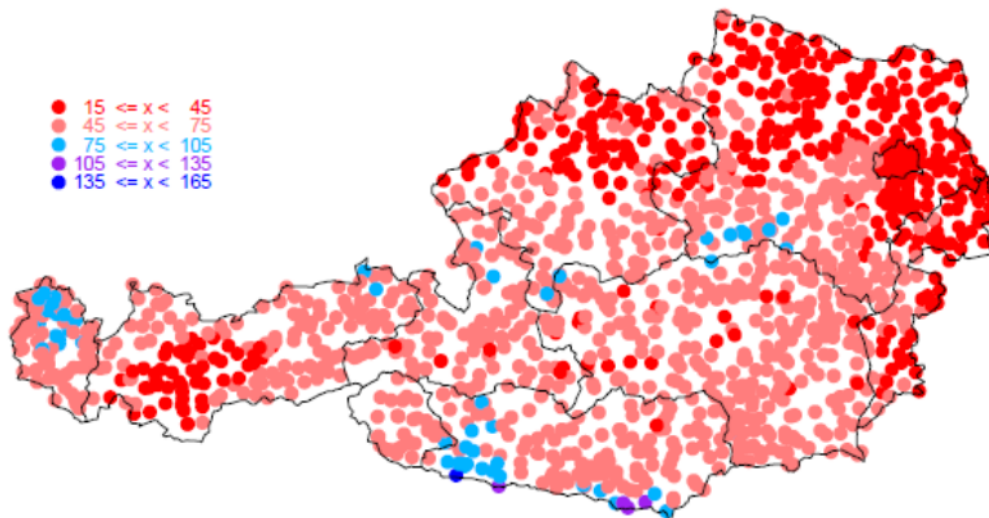
Abbildung 7. Messstellenwerte [mm] der ÖKOSTRA- Auswertung 2020. D: 1 Tag, T: 1
