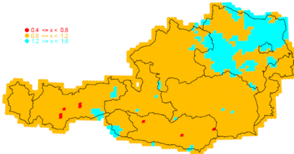
Abbildung 15. Quotient der interpolierten ÖKOSTRA-Auswertungen 2020 zu 2009. D: 60 Minuten, T: 1
