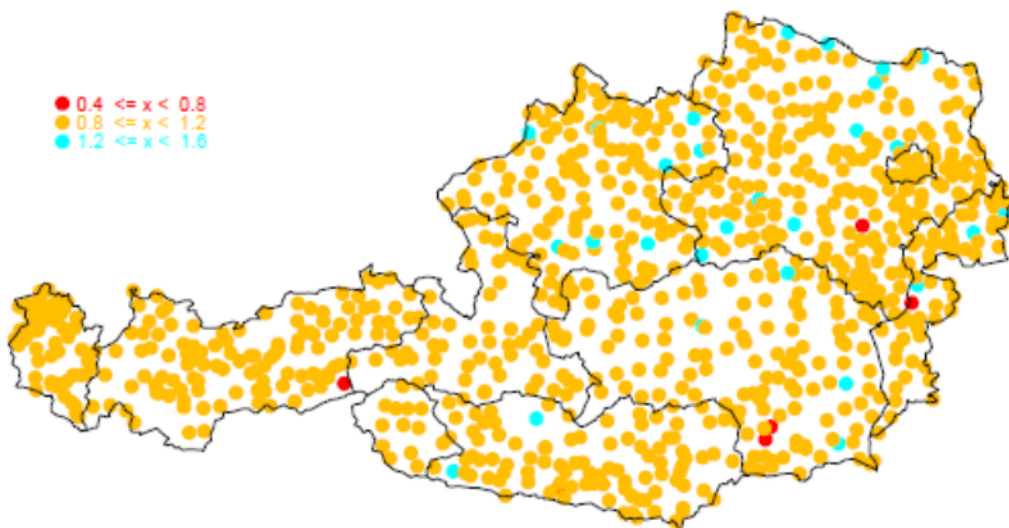
Abbildung 11. Quotient der ÖKOSTRA- Auswertung 2020 zu 2009. D: 1 Tag, T: 100
