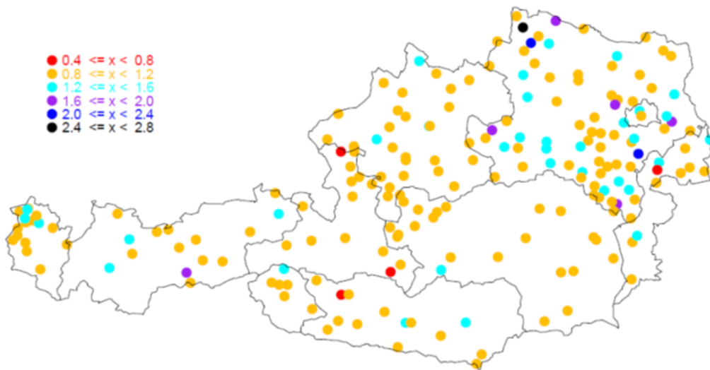
Abbildung 6. Quotient der ÖKOSTRA- Auswertung 2020 zu 2009. D: 15 Minuten, T: 100
