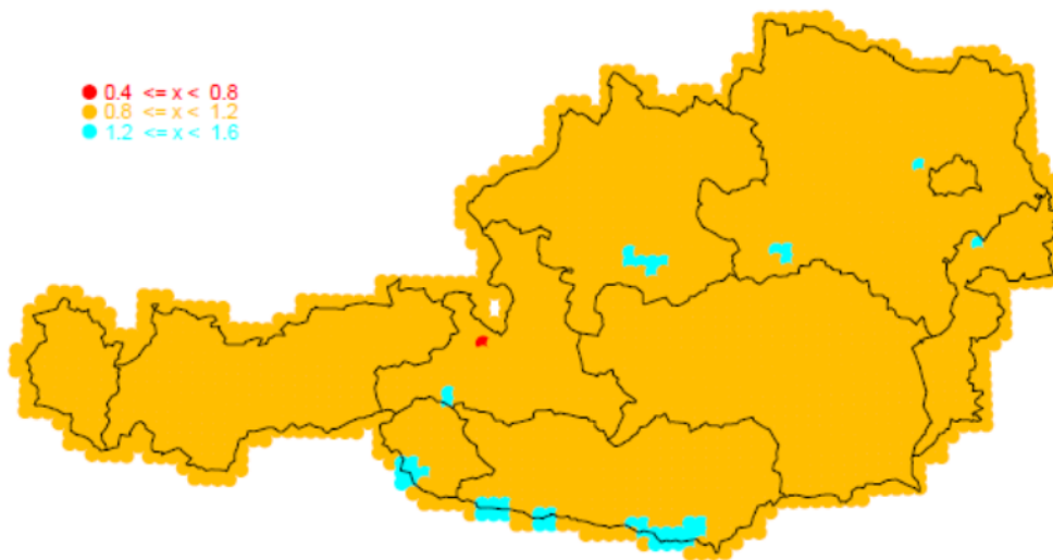
Abbildung 16. Quotient der interpolierten ÖKOSTRA-Auswertungen 2020 zu 2009. D: 6 Stunden, T: 1
