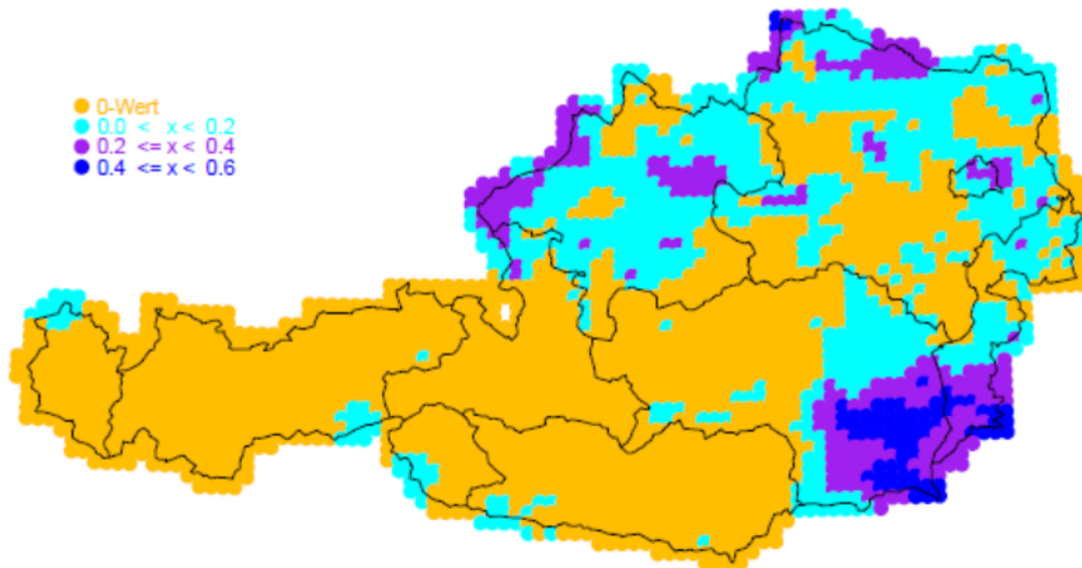
Abbildung 19. Normierte Abweichung der MaxModN-Werte 2020 zu den Werten von 2009. D: 15 Minuten, T: 1
