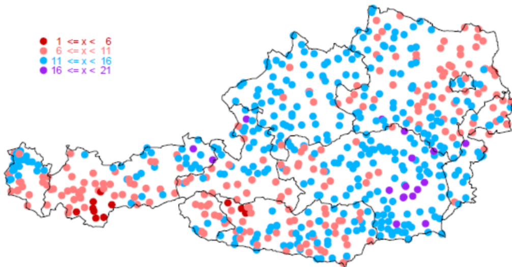
Abbildung 2. Messstellenwerte [mm] der ÖKOSTRA- Auswertung 2020. D: 15 Minuten, T: 1
