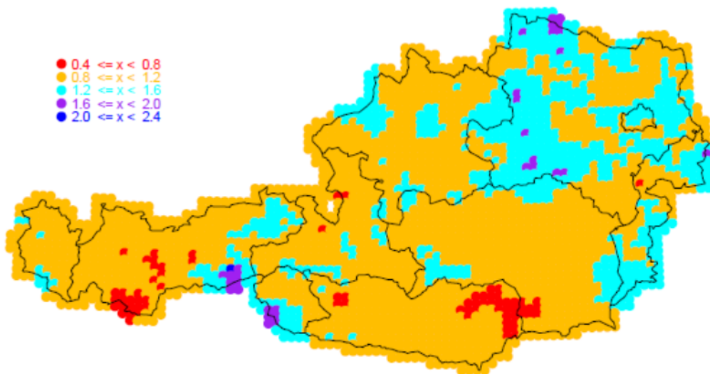
Abbildung 14. Quotient der interpolierten ÖKOSTRA-Auswertungen 2020 zu 2009. D: 15 Minuten, T: 100
