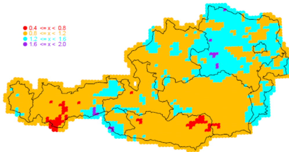
Abbildung 13. Quotient der interpolierten ÖKOSTRA-Auswertungen 2020 zu 2009. D: 15 Minuten, T: 10
