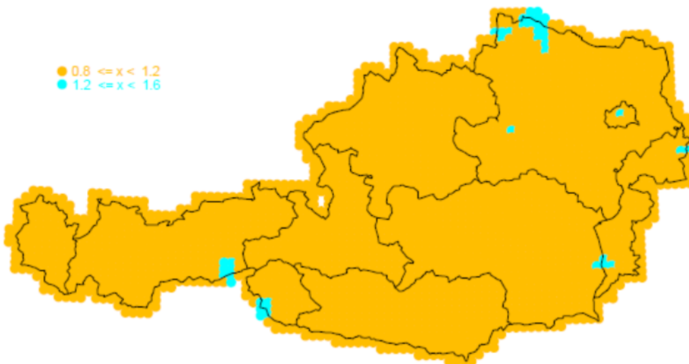
Abbildung 22. Quotient des Bemessungsniederschlags 2020 zu den Werten 2009. D: 15 Minuten, T: 100
