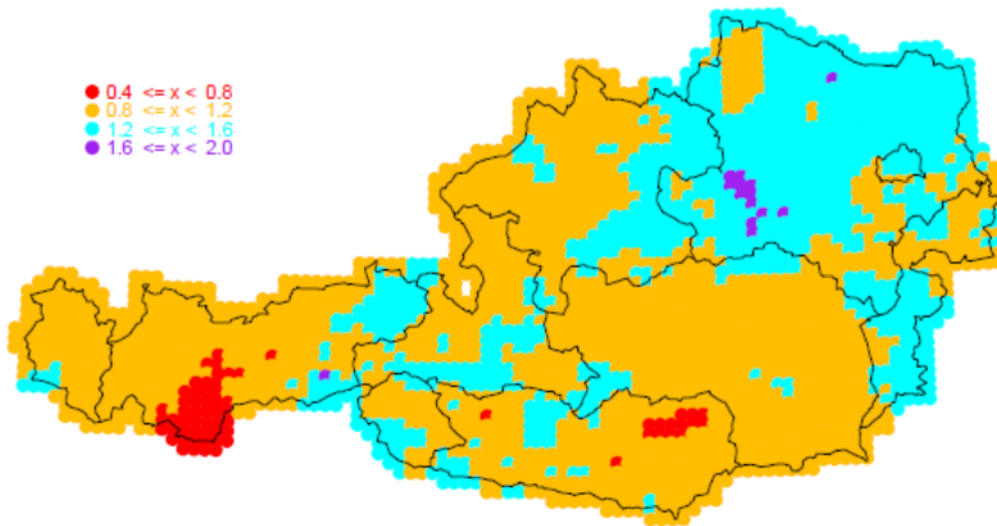
Abbildung 12. Quotient der interpolierten ÖKOSTRA-Auswertungen 2020 zu 2009. D: 15 Minuten, T: 1
