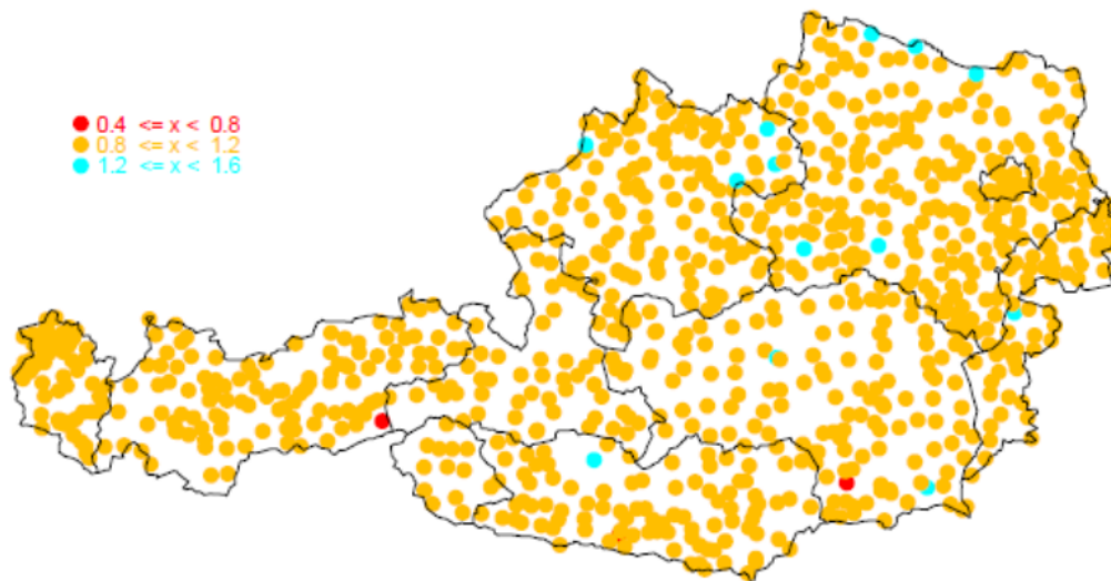
Abbildung 10. Quotient der ÖKOSTRA- Auswertung 2020 zu 2009. D: 1 Tag, T: 10
