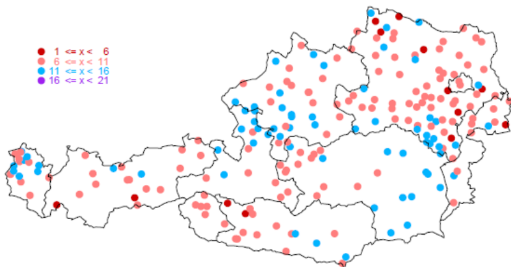
Abbildung 3. Messstellenwerte [mm] der ÖKOSTRA- Auswertung 2009. D: 15 Minuten, T: 1
