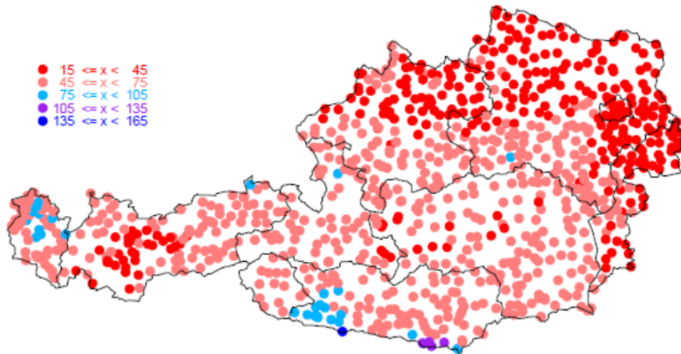
Abbildung 8. Messstellenwerte [mm] der ÖKOSTRA- Auswertung 2009. D 1 Tag, T: 1
