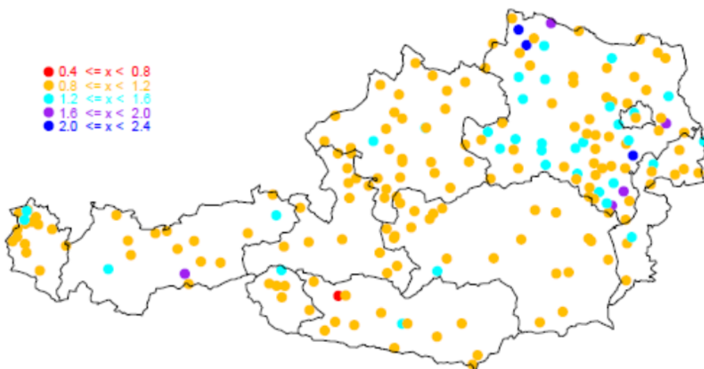
Abbildung 5. Quotient der ÖKOSTRA- Auswertung 2020 zu 2009. D: 15 Minuten, T: 10
