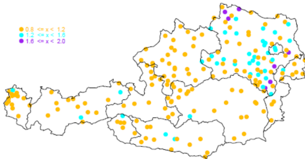
Abbildung 4. Quotient der ÖKOSTRA- Auswertung 2020 zu 2009. D: 15 Minuten, T: 1
