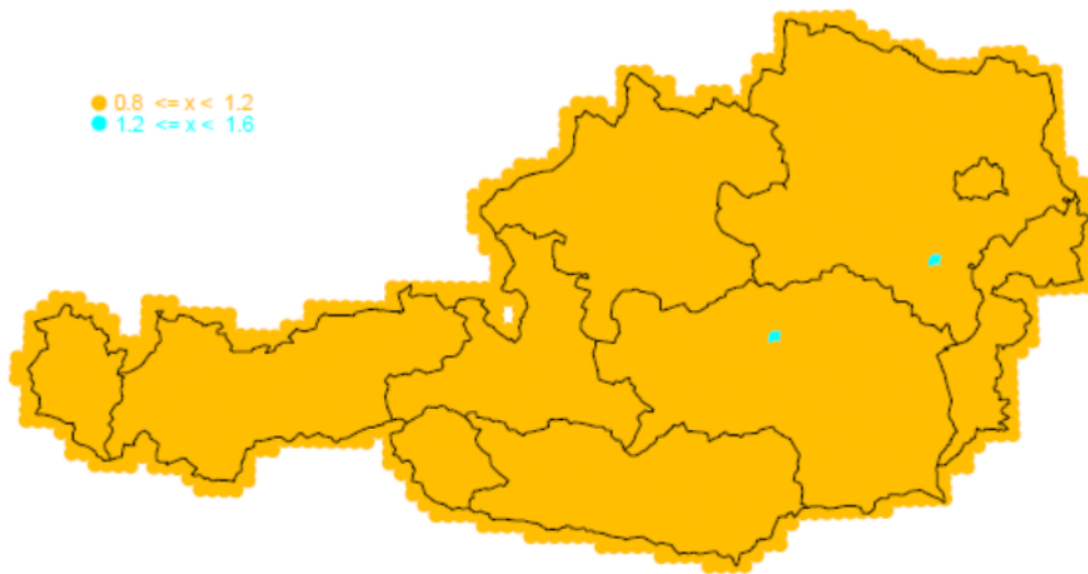
Abbildung 18. Quotient der interpolierten ÖKOSTRA-Auswertungen 2020 zu 2009. D: 1 Tag, T: 1
