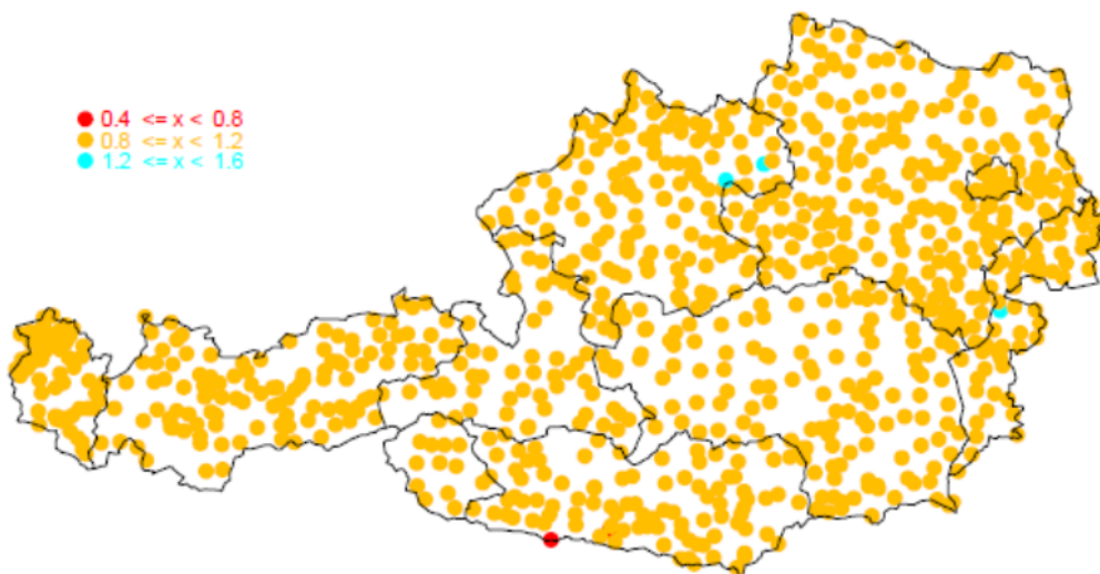
Abbildung 9. Quotient der ÖKOSTRA- Auswertung 2020 zu 2009. D: 1 Tag, T: 1
