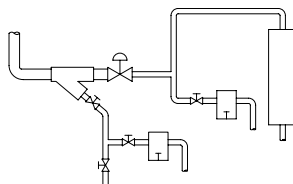
Abbildung CG-2727-3. Ungeachtet der Auslängelänge muss dem Regelventil unter der Dampfzufuhrleitung ein Kondensatsammelstutzen und ein Ableiter vorgeschaltet werden. Wenn sich die Rohrschlinge über dem Regelventil befindet, sollte dem Regelventil auch ein Ableiter nachgeschaltet werden.
