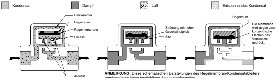
Abbildung CG-1919-1. Funktion eines Regelmembran-Kondensatableiters
