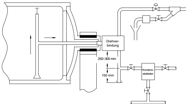
Abbildung CG-4646-1. Trockner mit außen anliegendem Produkt
