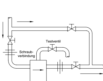
Abbildung CG-55-3. Typische Glockenkondensatableiter-Bypass-Installation
