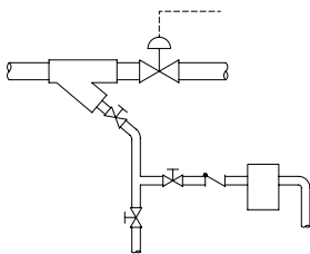
Abbildung CG-2626-1. Schmutzfänger des Ableiters vor Druckminderventil geschaltet
