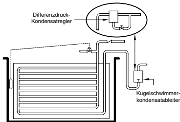
Abbildung CG-3737-1. Thermostatisch geregelter Plattenwärmeüberträger, Heberableitung
