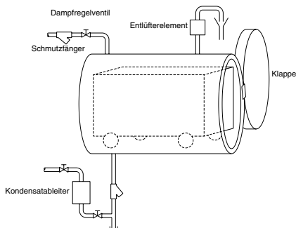
Abbildung CG-4545-1. Direkte Dampfinjektion in Produktkammer
