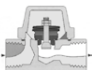
Abbildung CG-1919-2. Funktion eines Bimetallkondensatableiters
