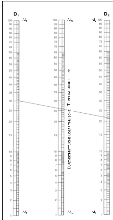
Diagramm CG-4141-1. Durchschnittliche Temperaturdifferenz für Wärmetauscherarmaturen
