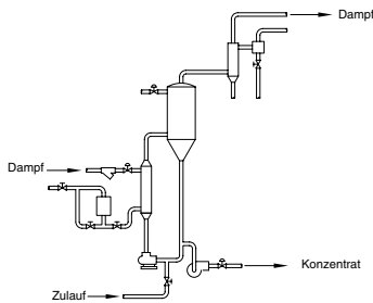
Abbildung CG-3939-1. Einfacheffekt-Verdampfungsanlage
