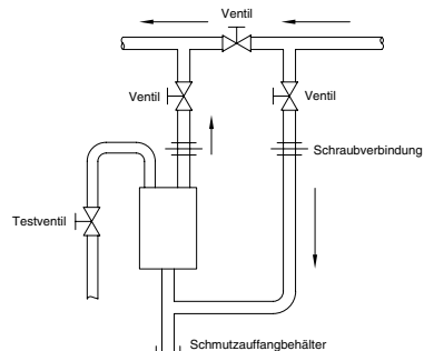
Abbildung CG-55-4. Typische Glockenkondensatableiter-Bypass-Installation, Einlass unten – Auslass oben
