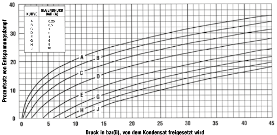
Diagramm CG-1111-1. Bei der Freisetzung von Kondensat unter geringerem Druck entstehender Entspannungsdampf in Prozent.
