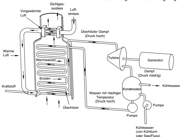
Abbildung CG-2828-1. Dampferzeuger
