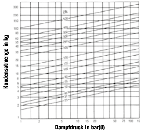
Diagramm CG-2525-1. Kondensatmenge für 20 m Rohr, das von 0°C auf Sattdampf Temperatur erwärmt wird
