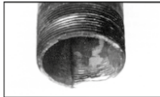
Abbildung CG-1515-2. CO 2 in Verbindung mit Kondensat, das unter Dampftemperatur abgekühlt ist, bildet Kohlensäure, die Rohre und Wärmeüberträger angreift. Bei dem dargestellten Rohrstück wurde der Werkstoff zersetzt.
