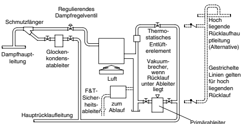
Abbildung CG-33-2. Ableitung und Entlüftung einer Luft-Heizschlange
