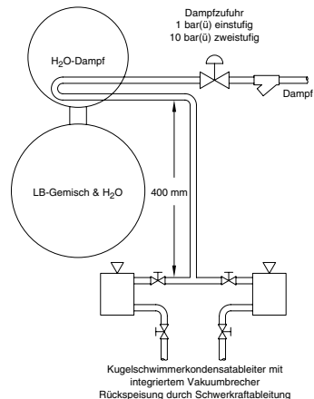
Abbildung CG-5050-1. Allgemein bewährte Verrohrung für DampfabSORBER mit Ersatzableiteranlage
