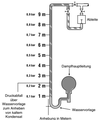
Abbildung CG-2323-2. Kondensat von der Schwerkraftabfuhrstelle wird durch ein Flüssigkeitsheber zum Ableiter gehoben. Jede Anhebung um 1 m senkt die Druckdifferenz um 0,1 bar. Am tiefsten Punkt ist eine Wasservorlage vorhanden und das eingebaute Rückschlagventil des Ableiters verhindert
