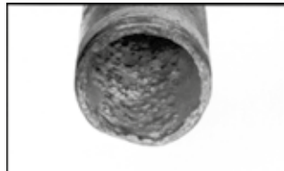
Abbildung CG-1515-3. Sauerstoff im System beschleunigt die Korrosion (Oxidation) von Rohren und führt hier gezeigt zu Rostnarben.
