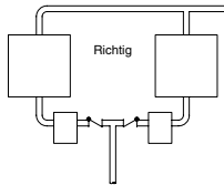
Abbildung CG-2222-2. Wenn jede Einheit über einen eigenen Ableiter verfügt, kann Medium nicht fehlerleitet werden. Auf diese Weise gewährleisten Sie einen höheren Wirkungsgrad.
