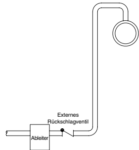
einen Rückfluss. Abbildung CG-2323-3. Wenn sich das Ableiterventil öffnet, hebt der Dampfdruck das Kondensat an. Jede Anhebung um 1 m senkt die Druckdifferenz um 0,1 bar.
