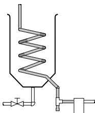
Abbildung CG-2222-3. Spiralband-Wärmeüberträger, Schwerkraftabführung zu Ableiter mit konstantem Druck. 300 kg/h Kondensat von einer einzelnen Kupferferroschlange mit 3 bar(ü). Schwerkraftabführung zu Ableiter. Außerst wenig Raum für Dampfvolumen. Sicherheitsfaktor 2:1.
