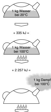
Abbildung CG-1212-1. Diese Zeichnungen zeigen, wie viel Wärme erforderlich ist, um bei atmosphärischem Druck ein Kilogramm Dampf zu erzeugen. Für je 1°C Temperaturanstieg bis zum Siedepunkt sind 4,186 kJ erforderlich, während um einiges mehr Kilojoule erforderlich sind, um Wasser bei 100°C in Dampf bei 100°C zu konvertieren.
