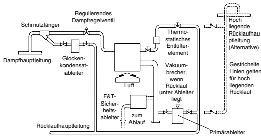
Abbildung CG-33-2. Ableitung und Entlüftung einer Luft-Heizschlange
