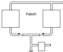
Abbildung CG-2222-1. Wenn zwei Dampfverbraucher mit einem Ableiter entleert werden (Sammelableitung), kann dies zu einer Fehlleitung des Mediums führen.
