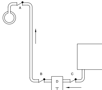
Abbildung CG-55-4. Typische Glockenkondensatableiter-Bypass-Installation, Einlass unten – Auslass oben
