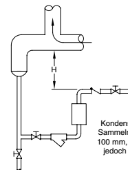
Abbildung CG-2626-3. Kondensatsammelstutzen des Ableiters an Steigrohr. Abstand „H“ in Metern geteilt durch 10 = statischer Druck (bar), mit dem Wasser durch den Ableiter gedrückt wird.
