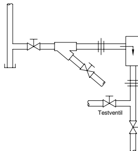
Abbildung CG-57-3. Typische Installation eines thermostatischen Kondensatableiters
