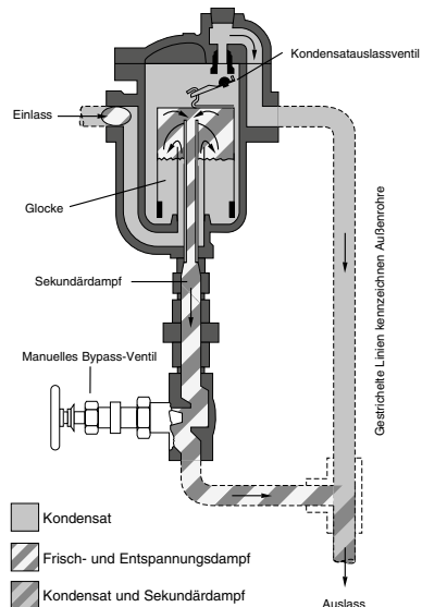
Abbildung CG-2121-2. Funktion eines Kondensatreglers
