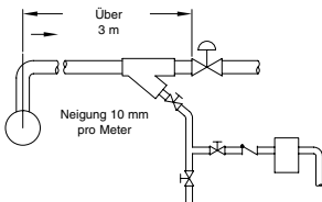
Abbildung CG-2727-2. Verrohrung für einen Auslauf über 3 m Länge. Dem Regelventil muss ein Kondensatsammelstutzen und ein Ableiter vorgeschaltet werden. Ein Schmutzfänger vor dem Regelventil kann als Kondensatsammelstutzen dienen, wenn der Abschlammanschluss zu einem Glockenkondensatableiter führt. Dies minimiert zudem den Reinigungsaufwand für den Schmutzfänger. Der Ableiter sollte mit einem innenliegenden Rückschlagventil oder einer vorgeschalteten Rückschlagklappe ausgerüstet sein.
