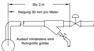
Abbildung CG-2727-1. Verrohrung für einen Auslauf unter 3 m Länge. Ein Ableiter ist nur erforderlich, wenn die Neigung zur Zulaufsammelleitung weniger als 50 mm pro Meter beträgt.
