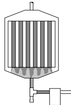
Abbildung CG-2222-4. Mehrere Rohre, Schwerkraftabführung zu Ableiter mit geregelterm Druck. 300 kg/h Kondensat von Lufterhitzer mit 5 bar(ü). Mehrere Rohre bergen eine gewisse Gefahr durch die Fehlleitung von Medium. Sicherheitsfaktor 3:1 bei 2,5 bar(ü).
