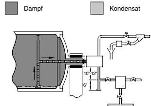
Abbildung CG-2222-5. Großer Zylinder, Heberableitung. 300 kg/h von einem Zylindertrockner mit 1.200 mm Durchmesser und 2.500 mm Länge mit einem Volumen von 2,8 m 3 bei 2 bar(ü). Der Sicherheitsfaktor ist für Differenzdruck-Kondensatregler 3:1 und für Glockenkondensatableiter 8:1.
