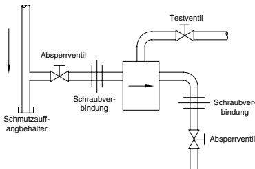
Abbildung CG-5254-1. Typische Installation eines Glockenkondensatableiters
