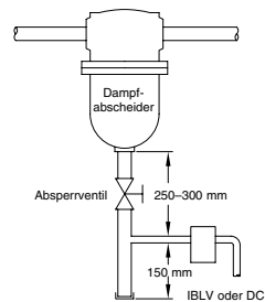
Abbildung CG-2727-4. Dem Abscheider nachgeschalteter Ableiter. Zur Gewährleistung eines positiven und schnellen Kondensatflusses zum Ableiter ist ein Kondensatsammelstutzen und ein Schmutzauffangbehälter in voller Größe erforderlich.
