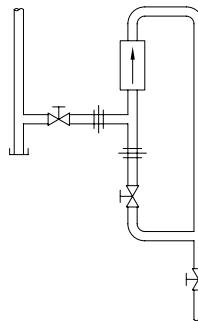
Abbildung CG-57-2. Typische Installation eines Regelmembran-Kondensatableiters
