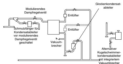
Abbildung CG-3535-1. Prozesslufferhitzer
