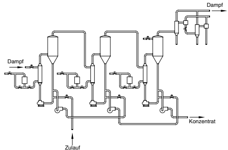
Abbildung CG-3939-2. Triple-Effekt-Verdampfungsanlage
