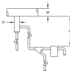
Abbildung CG-2626-2. Kondensatsammelstutzen des Ableiters an Hauptleitung
