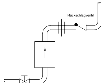
Abbildung CG-5254-2. Typische Installation eines Glockenkondensatableiters mit Einlass unten – Auslass oben
