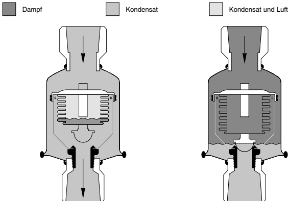
Abbildung CG-2020-1. Funktion eines Kondensatableiters
