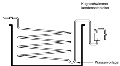
Abbildung CG-3737-2. Spiralband-Wärmeüberträger, Heberableitung
