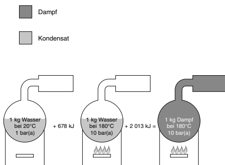
Abbildung CG-1212-2. Diese Zeichnungen zeigen, wie viel Wärme erforderlich ist, um ein Kilogramm Dampf bei einem Druck von 10 bar(a) zu erzeugen. Beachten Sie die zusätzliche Wärme und höhere Temperatur, die gegenüber der Erwärmung bei Atmosphärendruck erforderlich sind, um Wasser bei 10 bar(a) zum Kochen zu bringen. Im Gegensatz dazu wird jedoch weniger Wärme benötigt, um Wasser bei der höheren Temperatur zu verdampfen.
