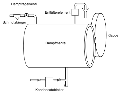
Abbildung CG-4545-2. Produkt in Kammer – Dampf in Doppelwand
