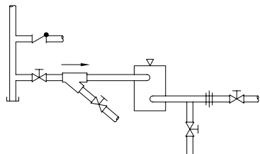
Abbildung CG-56-3. Typische Installation eines Kugelschwimmerkondensatableiters
