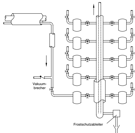
Typische Begleitheizungsinstallation
