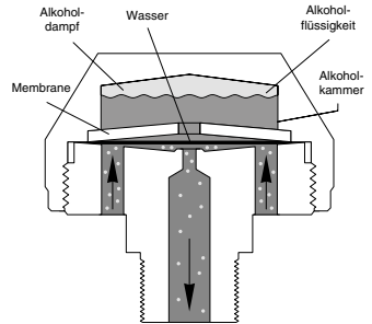
Abbildung CG-2020-2. Funktion eines thermostatischen Kapselableiters
