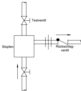
Abbildung CG-55-3. Typische Glockenkondensatableiter-Bypass-Installation
