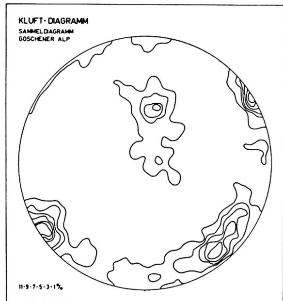
Fig. 5: Verteilung der Klüfte im Zentralgranit der Göschener Alp. – Darstellung der Kluftlagen als Diagramm. Die Prozentwerte bezeichnen die Besetzungsdichten der verschiedenen Flächen.
