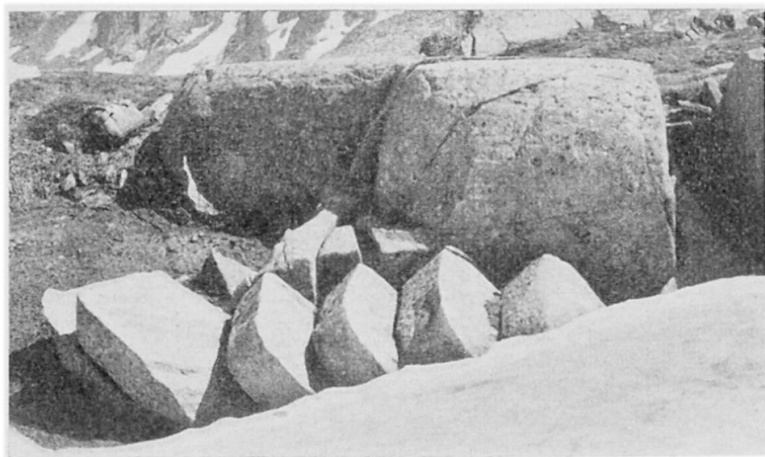
Abb. 1: Längs einer Klufte zerfallener Rundhöcker W Grimselpaß. Die schrägliegenden Steinplatten standen ursprünglich mehr rechts, außerhalb des Bildausschnittes. Als Größenvergleich mag der Rucksack (hinten links) dienen.
