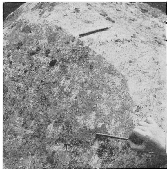
Abb. 19: Abhebekante der Schiffe jüngerer Richtung (Bleistift; von rechts nach links) von den Schliffen der ältern Richtung (Hand mit Bleistift; gegen den Beschauer).
