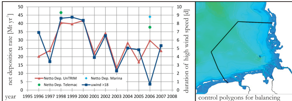
Abbildung 18: Über den Rand der Deutschen Bucht integrierte Netto-Deposition aus UnTRIM (rot), TELEMAC (grün) und MARINA (hellblau) und Dauer hoher Windgeschwindigkeiten ( > 18 \text{ m/s} ) bei Helgoland. In der rechten Abbildung sind die Kontrollabschnitte für die Bilanzierung markiert.
