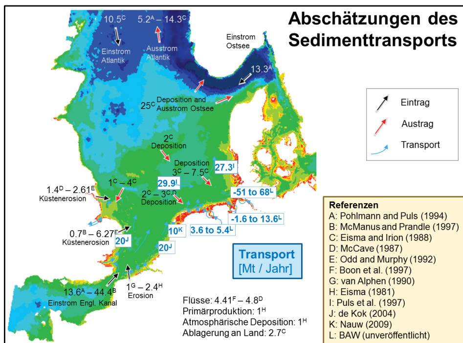
Abbildung 15: Schätzung der Sedimenttransportbilanzen in der Literatur.
