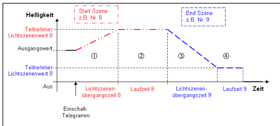
Abb. 8 Graphische Darstellung des Dynamik-Betrieb
