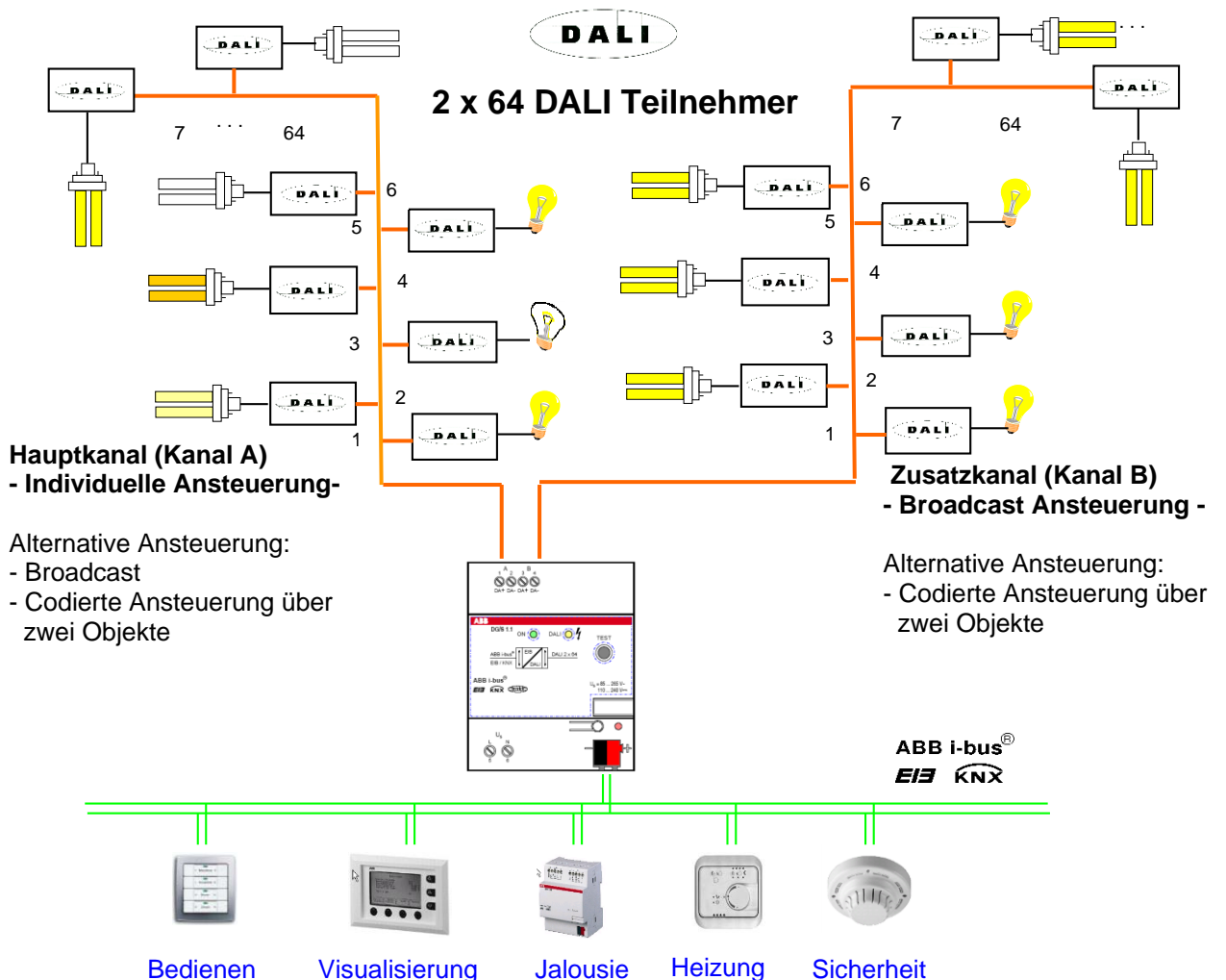
Abb. 2 DALI-Gateway DG/S 1.1 Prinzipschaltbild
