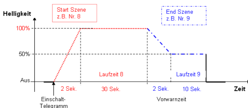
Abb. 26 Treppenlichtverlauf
