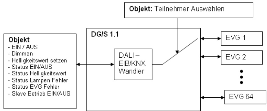
Abb. 23 Prinzipschaltbild – Teilnehmer Auswahl
