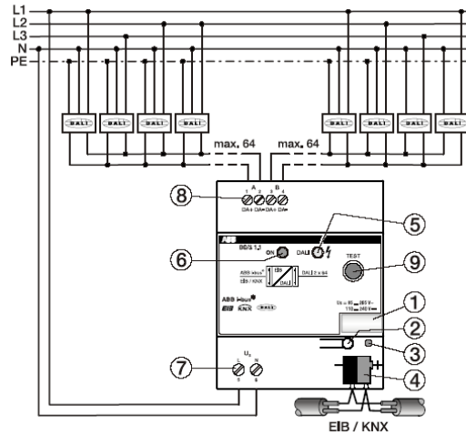
Abb. 4: Anschlussbild des 1fach DALI-Gateway DG/S 1.1
