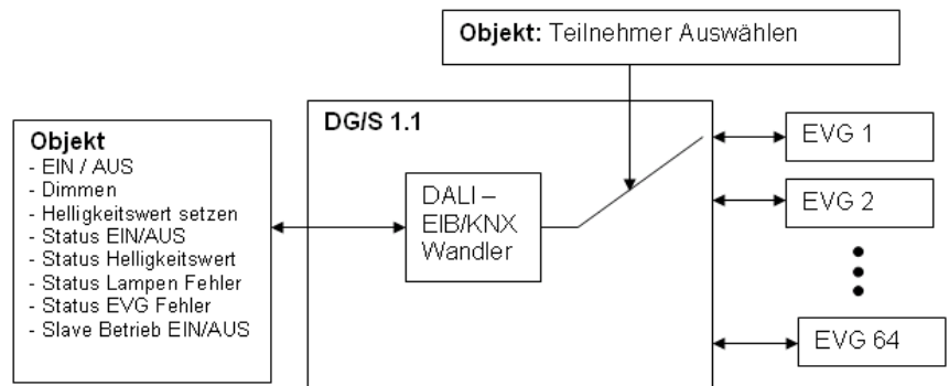
Abb. 15 Prinzipschaltbild – Teilnehmer Auswahl
