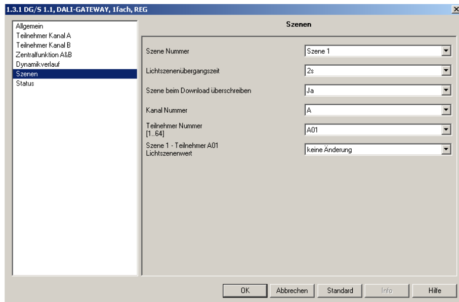
Abb. 13: Parameterfenster "Szenen"
