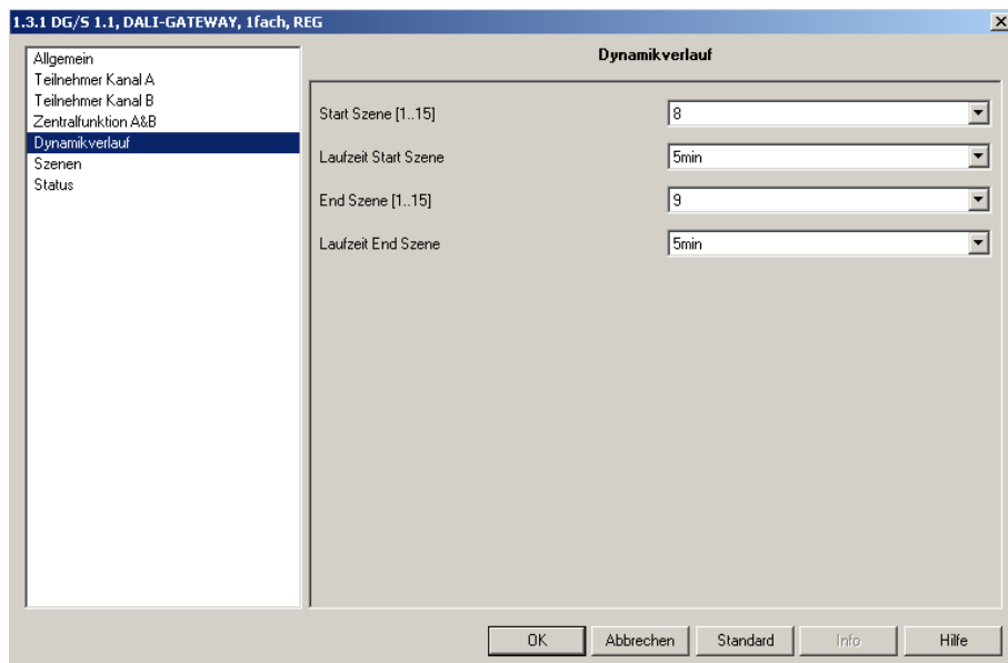
Abb. 11: Parameterfenster "Dynamikverlauf"
