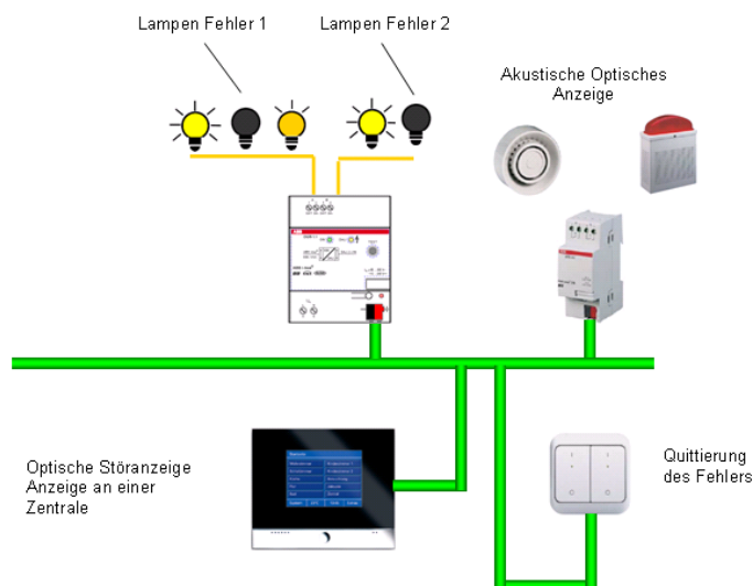
Abb. 35 Systemdarstellung Störmeldung
