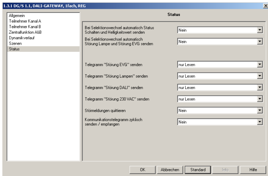
Abb. 14: Parameterfenster "Status"
