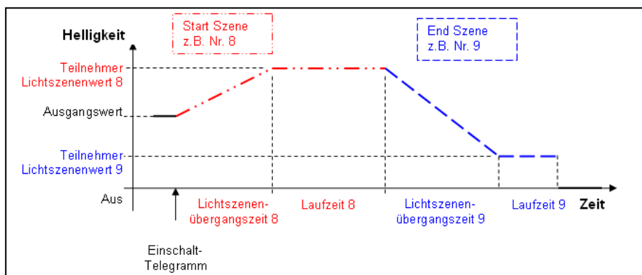
Abb. 12 Graphische Darstellung des Dynamik-Betrieb
