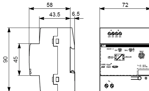
Abb. 5: Maßbild DG/S 1.1
