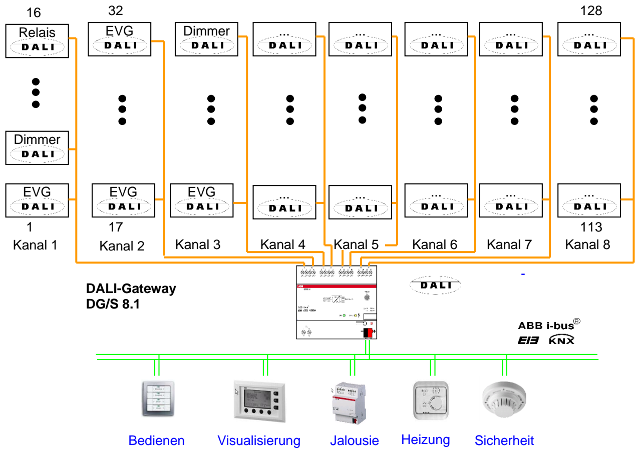
Abb. 3 DALI-Gateway DG/S 8.1 Prinzipschaltbild
