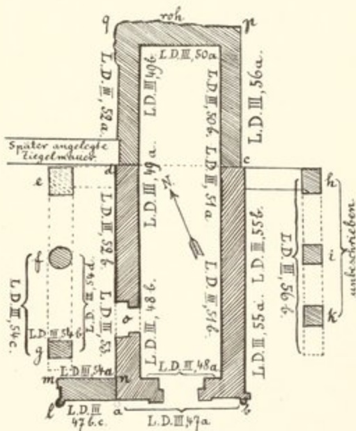
Grundriss des Tempels von Semneh (nach Lepsius).
