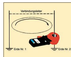
Prinzip der Basis-Schleife: sie besteht aus zwei lokalen Erdungen, die mit einem Leiter verbunden werden.
