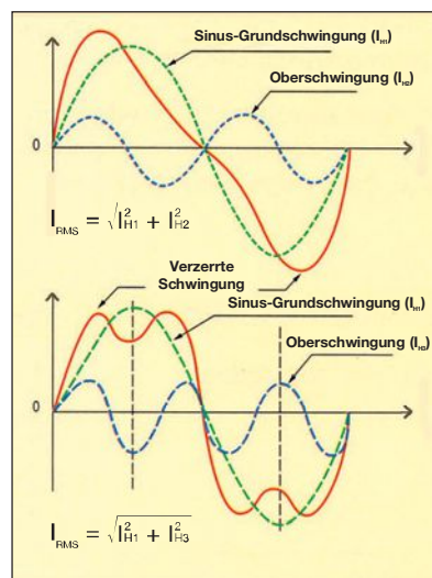
Abb. 2 - Zerlegung einer verzerrten Schwingung in Grundschwingung und Oberschwingung 2. bzw. 3. Ordnung
