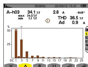
Vberschwingungsanalyse
