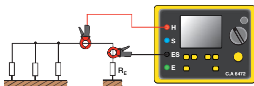
Prinzipschema eines ausgedehnten Erdungsnetzes. In der Praxis besteht eine Erdung meist aus mehreren Basis-Schleifen, die ein ausgedehntes Erdungsnetz bilden.
