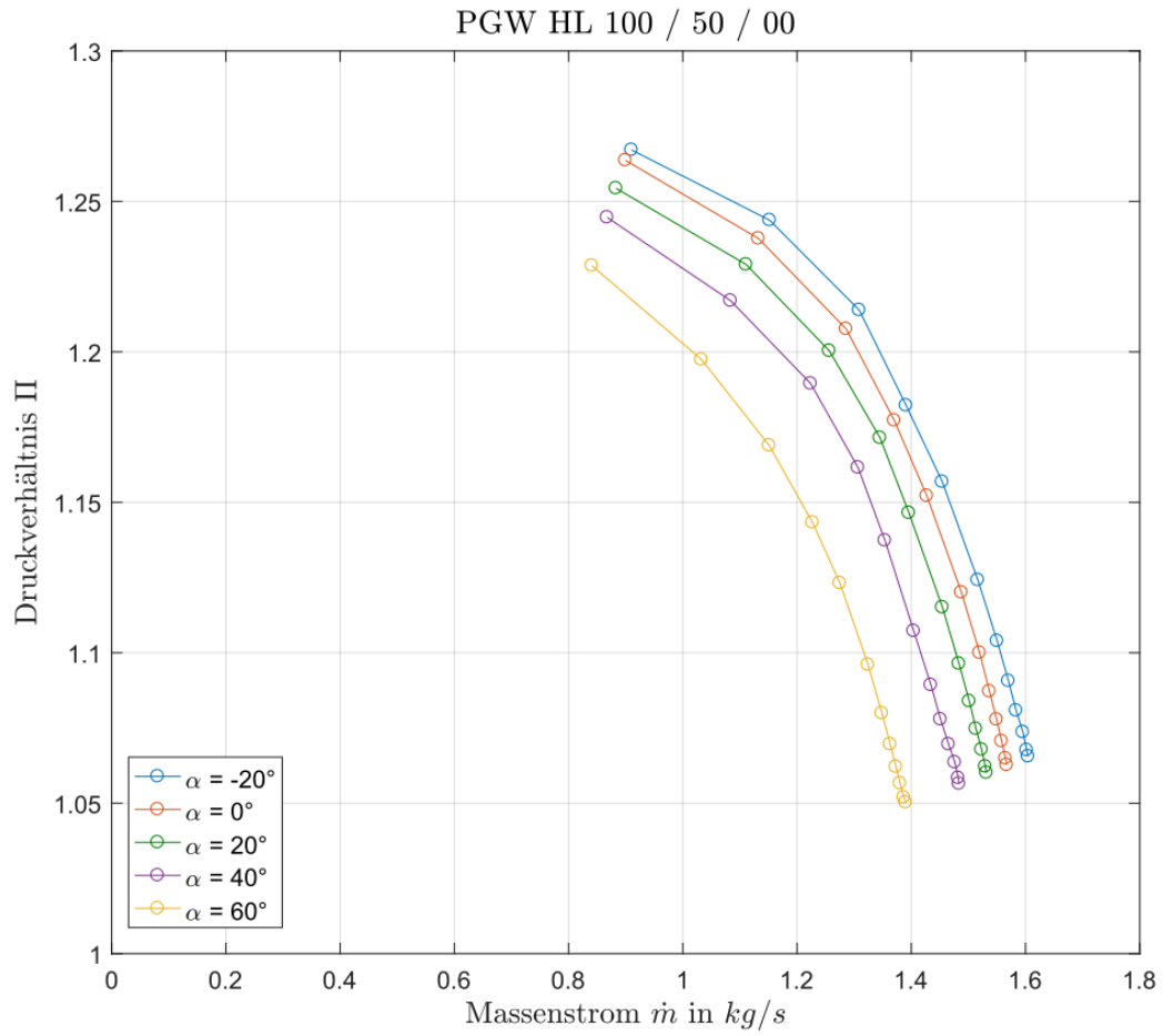
Abbildung 5.9: Kennfeld des Verdichters PGW HL 100 / 50 / 00 mit Vordrallregelung
