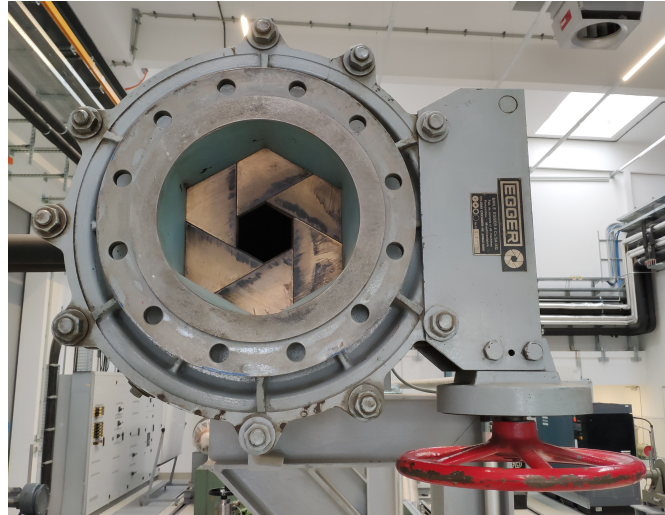
Abbildung 3.2: Drosselschieber in leicht geöffneter Position
