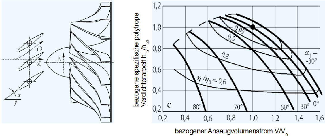
Abbildung 2.9: links: Funktionsskizze eines Vordrallreglers [9]; rechts: Kennfeld eines Verdichters mit Vordrallregelung [9]
