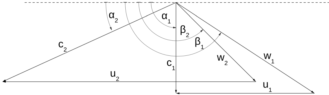
Abbildung 2.3: gemeinsame Darstellung der Geschwindigkeitsdreiecke des Verdichterlaufrades
