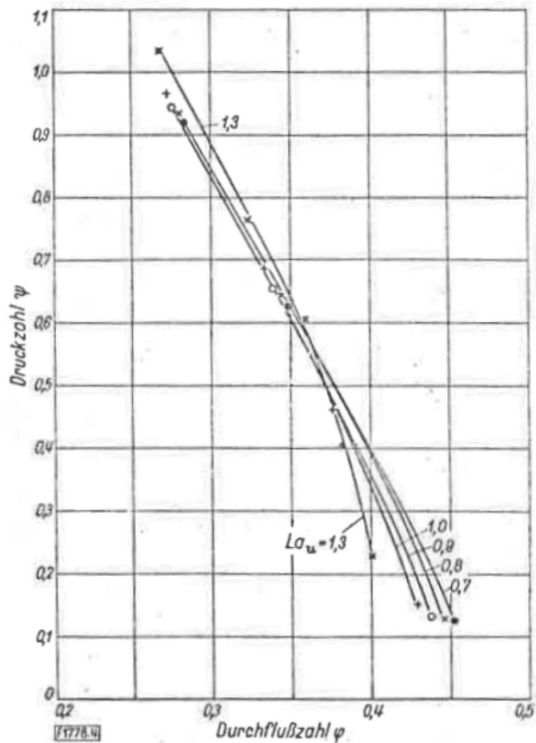
Abbildung 2.11: Kennlinien für eine verlustlose Axialverdichterstufe bei Lavalzahlen La_u = [0.7, 0.8, 0.9, 1.0, 1.3] aus [11]
