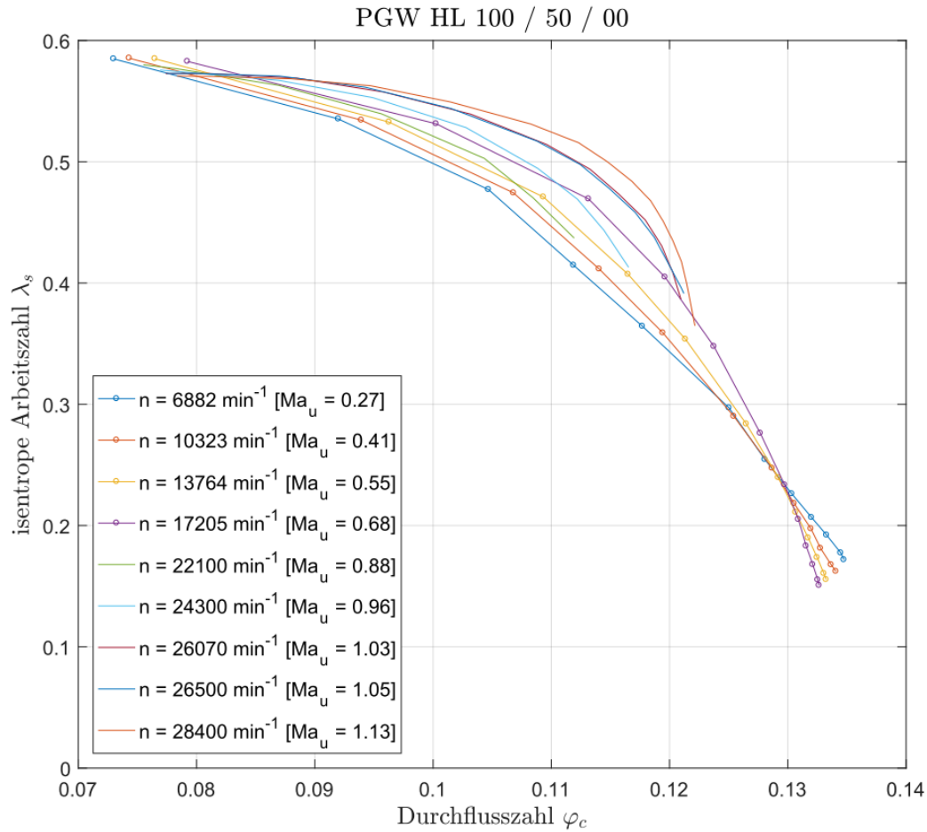
Abbildung 5.19: Verläufe der isentropen Arbeitszahl \lambda_s des Herstellerkennfeldes und des aufgenommenen Kennfeldes des Verdichters PGW HL 100 / 50 / 00
