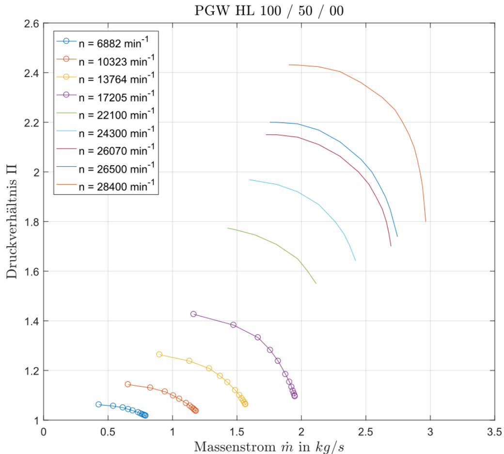
Abbildung 5.14: Gemeinsame Darstellung des aufgenommenen Kennfeldes und des Herstellerkennfeldes des Verdichters PGW HL 100 / 50 / 00
