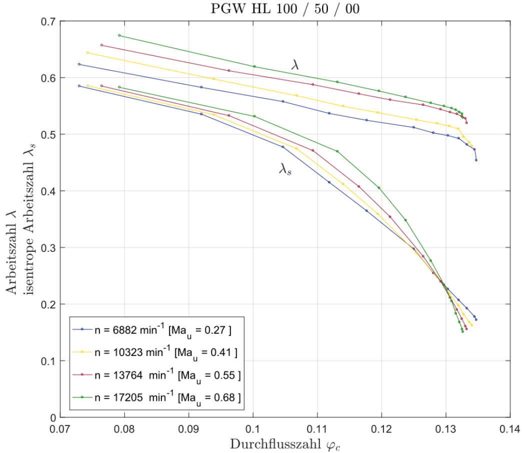
Abbildung 5.6: Dimensionslose Darstellung der Kennlinien des Verdichters PGW HL 100 / 50 / 00 mit Drehzahlregelung
