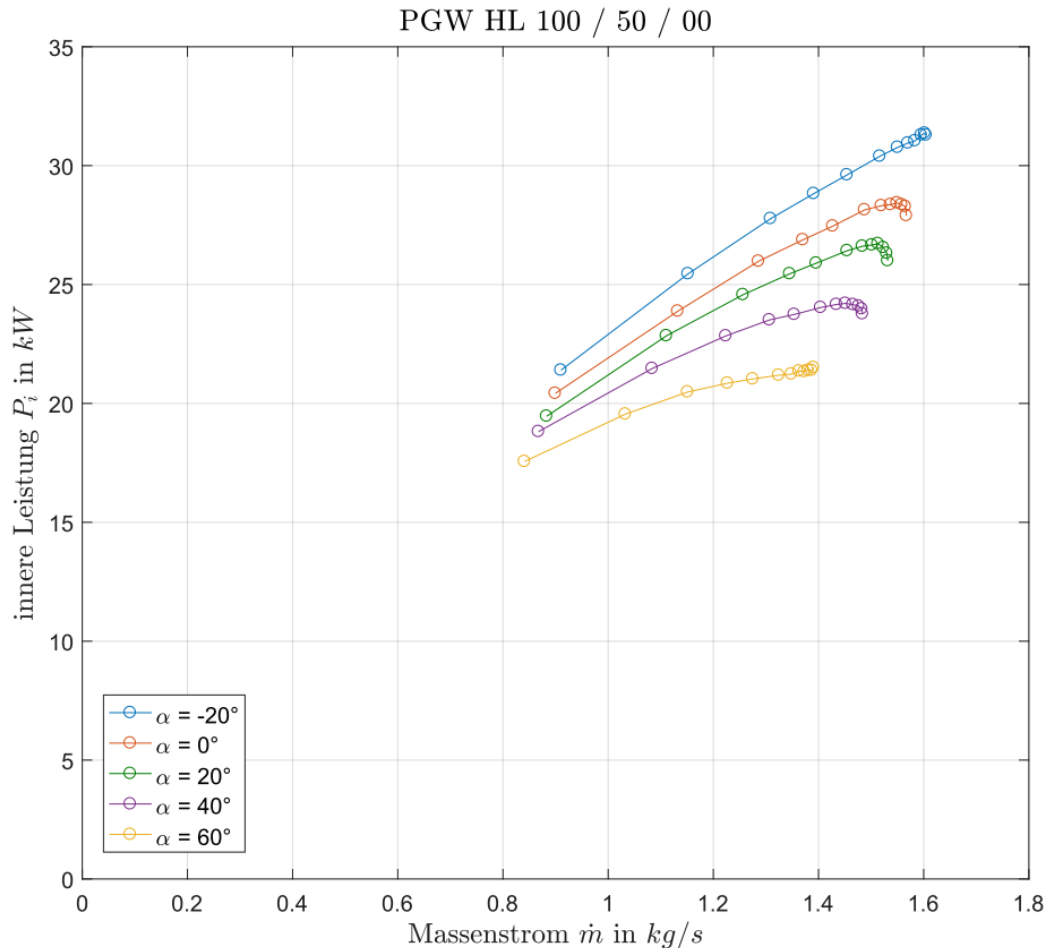
Abbildung 5.11: Innere Leistung des Verdichters PGW HL 100 / 50 / 00, Vordrallregelung
