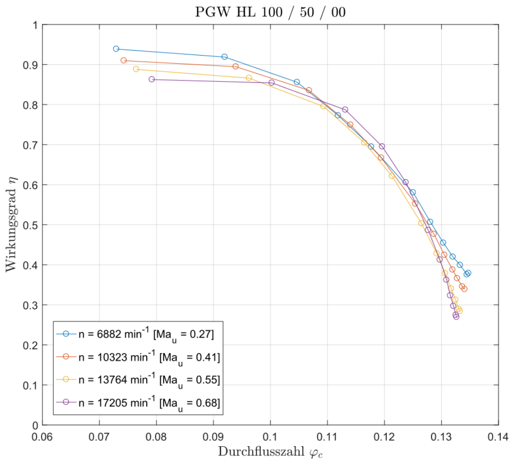
Abbildung 5.7: Dimensionslose Darstellung der Wirkungsgradverläufe des Verdichters PGW HL 100 / 50 / 00 mit Drehzahlregelung
