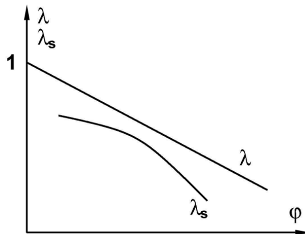
Abbildung 2.10: \lambda , \varphi - und \lambda_s , \varphi -Charakteristik einer Verdichterstufe [5]
