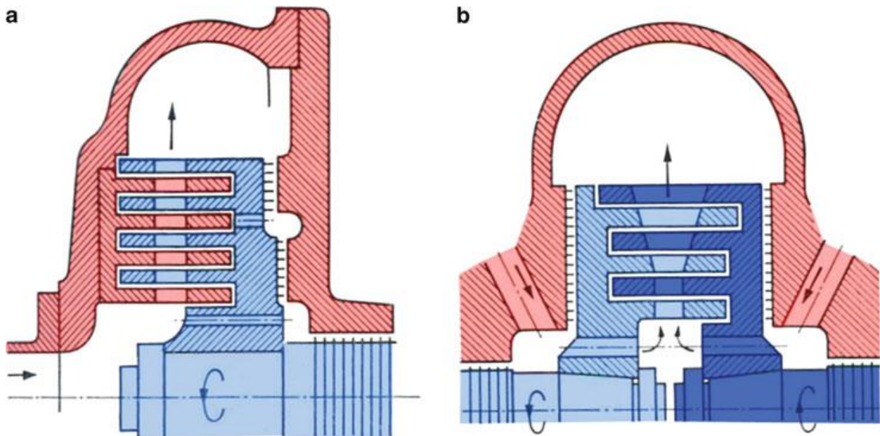
Abbildung 23: a) einläufige Radialturbine; b) gegenläufige Ljungström-Turbine [2]
