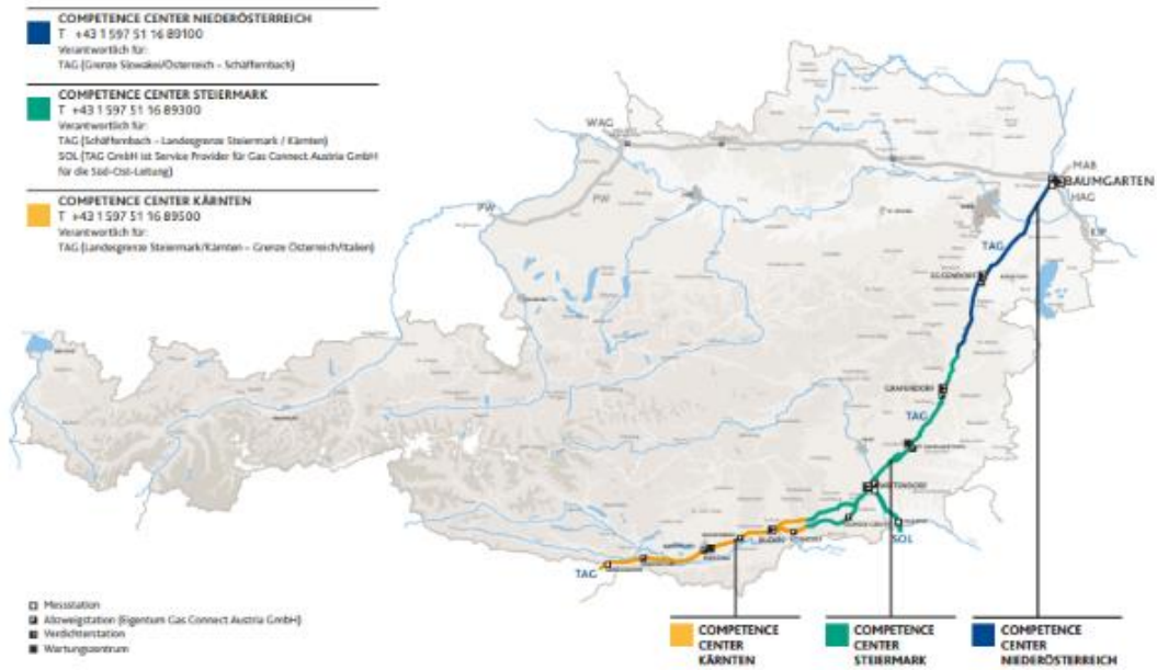
Abbildung 42: TAG Pipelinenetz [12]
