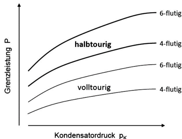
Abbildung 34: Halb- und volltourige Ausführung der Dampfmaschinen für Kernkraftwerke [2]
