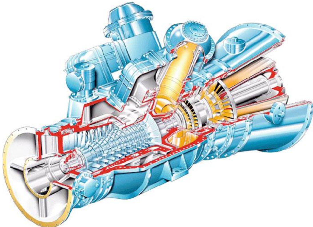
Abbildung 7: Zweiwellige stationäre Gasturbine in Schwerbauweise [1]
