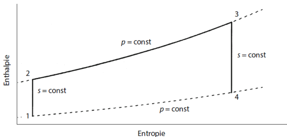
Abbildung 5: (Teil-) Idealer Joule-Prozess [1]
