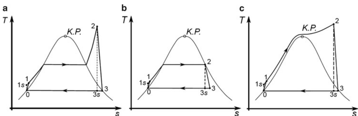
Abbildung 16: T,s-Diagramm des einfachen Clausius-Rankine-Prozesses a) Unterkritischer Dampfprozess b) Sattdampfprozess c) Überkritischer Dampfprozess [2]
