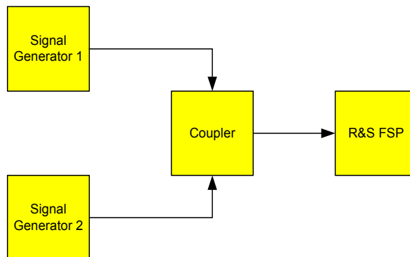
Bild 2.4 Messaufbau zur Generierung von zwei Signalen
