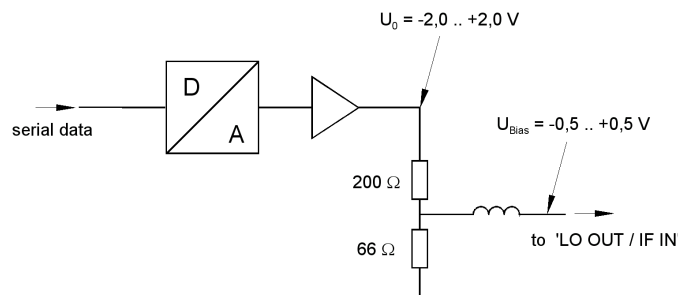
Bild 4.40 Bias-Schaltung des R&S FSP
