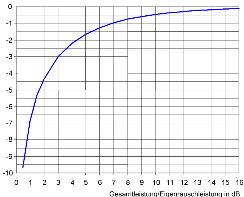
Bild 2.16 Korrekturfaktor für die gemessene Rauschleistung abhängig von Abstand zu Eigenrauschleistung des R&S FSP
