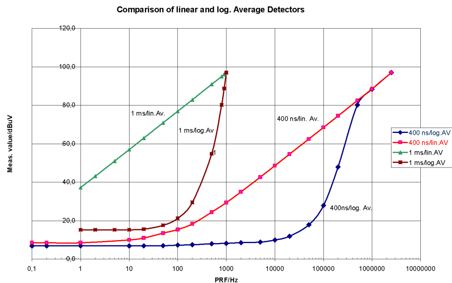
Bild 4.2 Ansprechverhalten des linearen und des logarithmischen Mittelwert-Detektors als Funktion der Puls wiederholfrequenz (PRF) für pulsmodierte Signale mit Impulsdauern von 400 ns und 1 ms. Die Auflösungsbandbreite ist 1 MHz.
