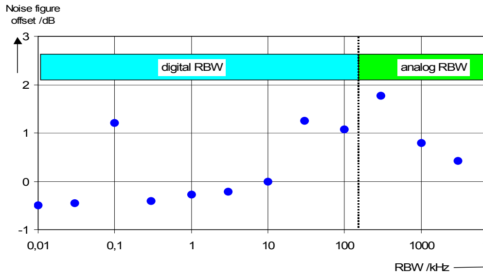
Bild 2.10 Änderung des Rauschmaßes des R&S FSP bei den verschiedenen Bandbreiten. Als Bezugsbandbreite ist 10 kHz gewählt.
