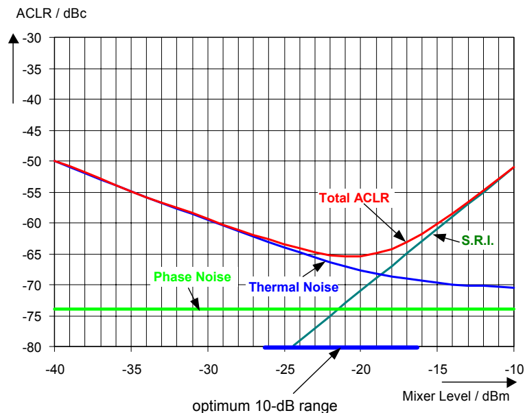
Bild 2.38 Dynamik des R&S FSP bei Nachbarkanalleistungsmessung an W-CDMA-Uplink-Signalen abhängig vom Mischerpegel.
