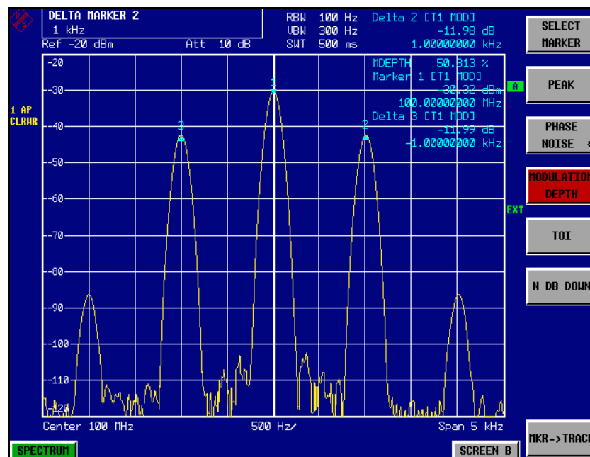
Bild 2.23 Messung des AM-Modulationsgrades. Der Modulationsgrad kann hier mit MDEPTH = 49.436\% abgelesen werden. Die Frequenz des NF-Signals kann der Frequenzanzeige der Delta-Marker entnommen werden
