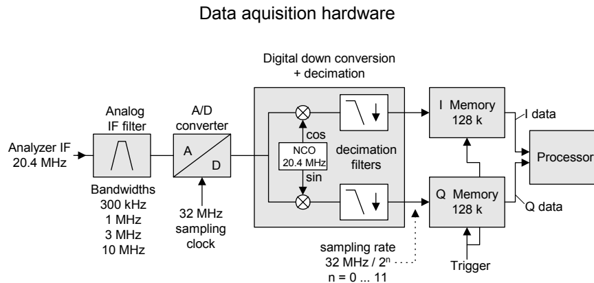
Bild 6.25 Blockschaltbild mit der Signalverarbeitung des R&S FSP
