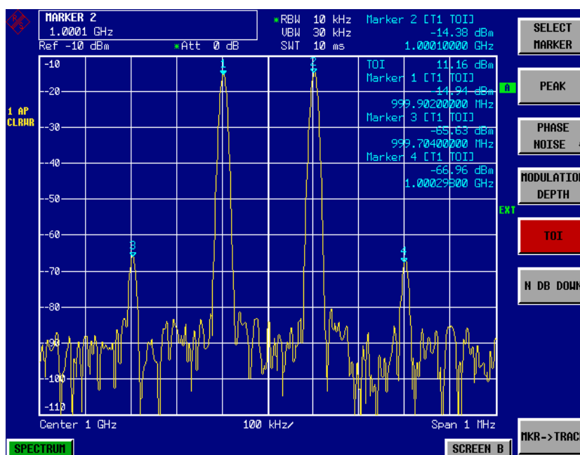
Bild 2.5 Ergebnis der Messung des Eigen-Intermodulationsabstandes des R&S FSP. Der Interceptpunkt dritter Ordnung (TOI) wird am rechten oberen Rand des Grids ausgegeben
