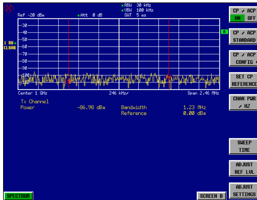
Bild 2.17 Messung der R&S FSP-Eigenrauschleistung in 1,23 MHz Kanalbandbreite.
