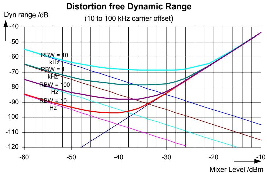
Bild 2.8 Intermodulationsfreier Bereich des R&S FSU3 abhängig vom Pegel am Eingangsmischer und der eingestellten Auflösebandbreite (Nutzsignalabstand = 10 bis 100 kHz, DANL = -157 dBm/Hz, T.O.I = 25 dBm; typ. Werte bei 2 GHz)
