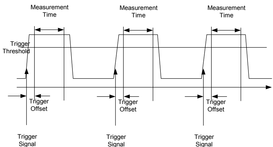
Bild 7.7 Signalverlauf und Zeitverhältnisse des zu messenden Signals
