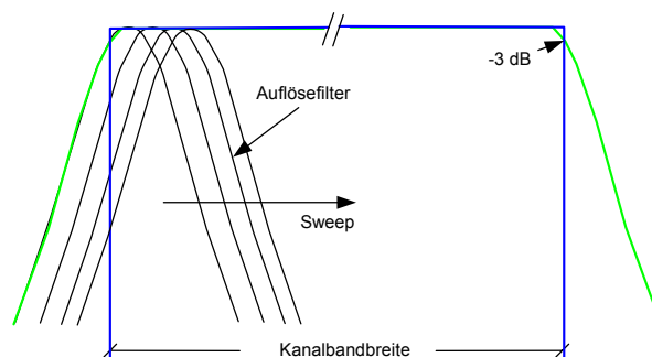
Bild 2.18 Approximation des Kanalfilters durch Sweepon mit kleiner Auflöseseite
