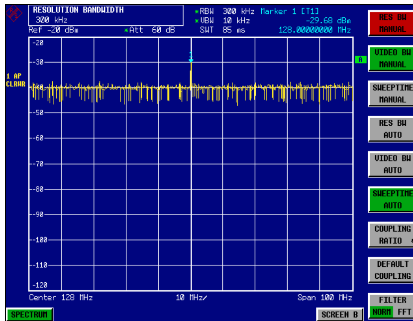
Bild 2.14 Anzeige des Referenzsignals bei kleinerer Auflösungsbandbreite.
