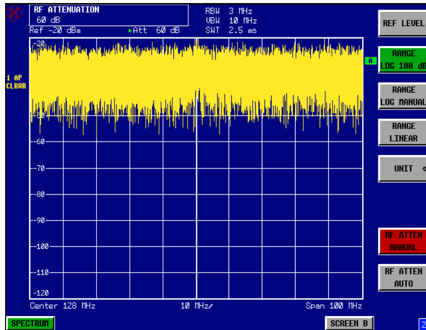
Bild 2.11 Darstellung eines Sinussignals mit kleinem Rauschabstand. Das Signal wird mit dem Auto-Peak-Detektor gemessen fast vollständig durch das Eigenrauschen des R&S FSP überdeckt.
