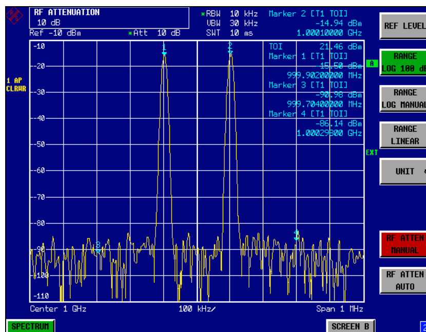
Bild 2.6 Durch Erhöhung der HF-Dämpfung verschwinden die R&S FSP-Eigenstörprodukte im Rauschen.
