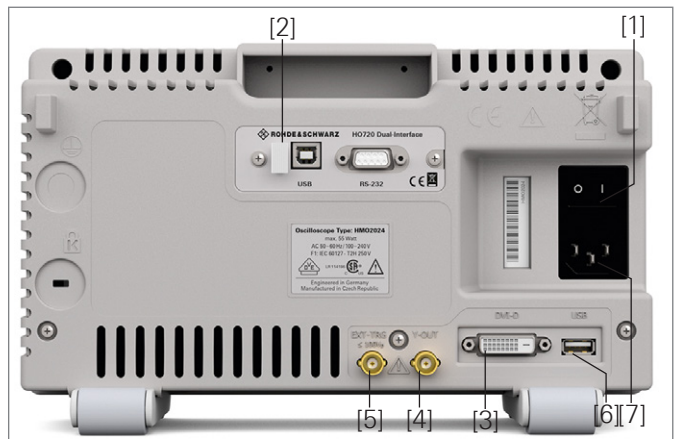
Abb. 2.14: Geräterückseite R&S®HMO2024
