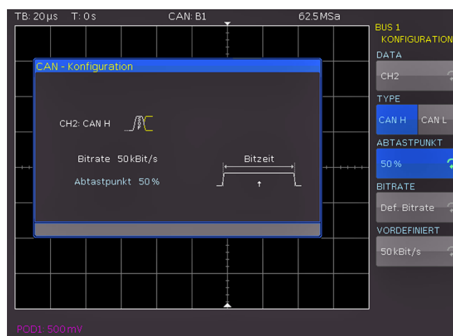
Abb. 12.18: Einstellung des Abtastzeitpunktes bei der CAN Konfiguration
