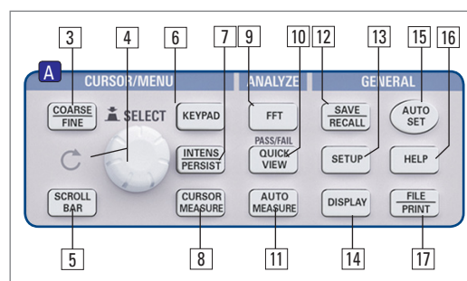
Abb. 2.2: Bedienfeldabschnitt A
