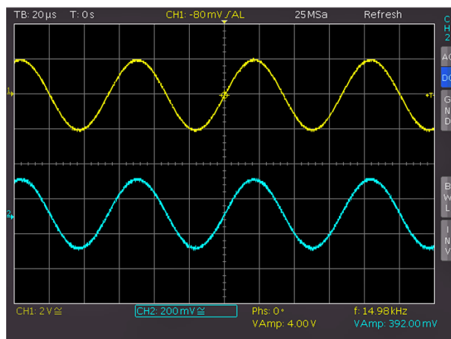
Abb. 2.15: Signal Y-Ausgang
