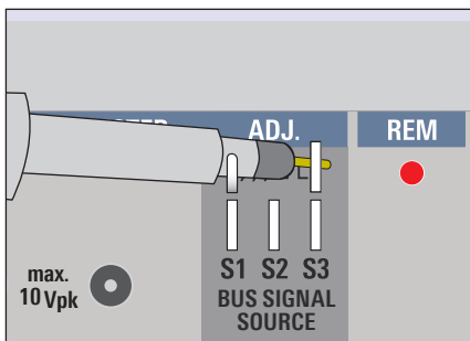
Abb. 4.3: Korrekter Tastkopfanschluss am Probe Adjust Ausgang
