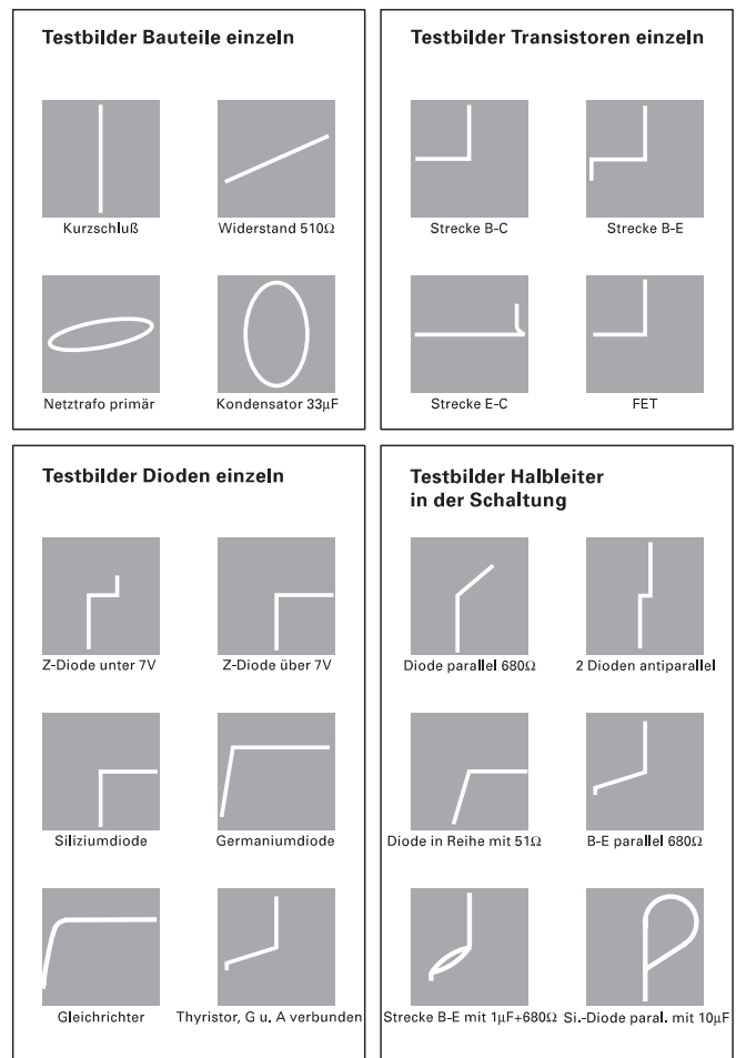
Abb. 9.11: Komponententester Testbilder
