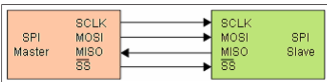
Abb. 12.9: Einfache Konfiguration eines SPI BUS
