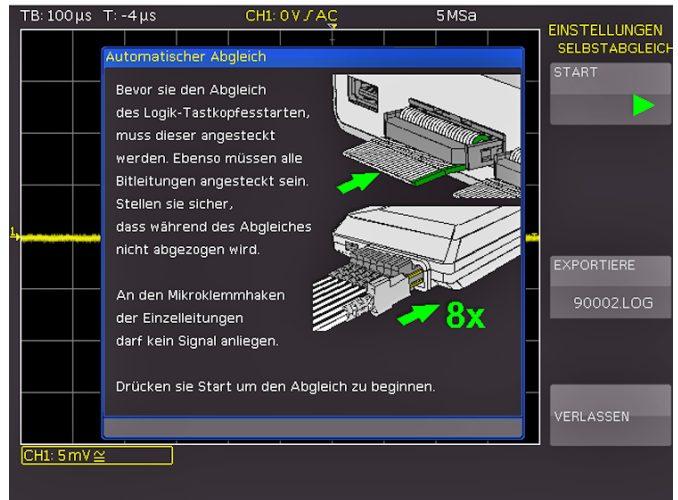
Abb. 2.13: Selbstabgleich Logiktastkopf
