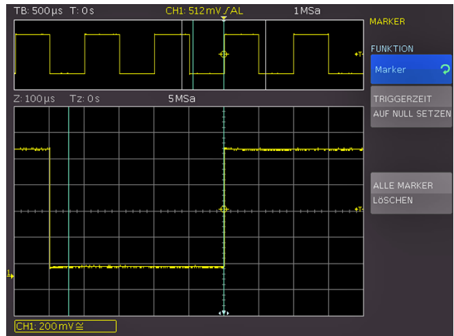
Abb. 5.6: Marker im Zoom Modus
