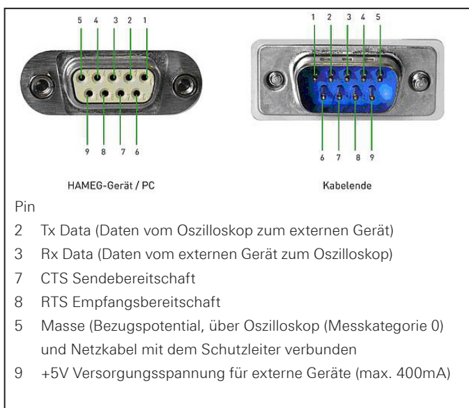
Abb. 13.1: Pinbelegung der RS-232 Schnittstelle
