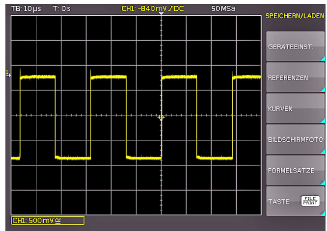
Abb. 3.12: Speichern und Laden Menü
