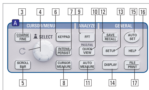
Abb. 3.1: Bedienfeldabschnitt A
