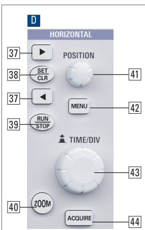
Abb. 3.5: Teil D des Bedienfeldes mit Zoomtaste
