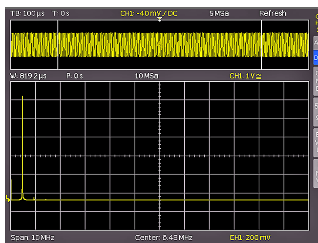
Abb. 9.7: FFT Darstellung
