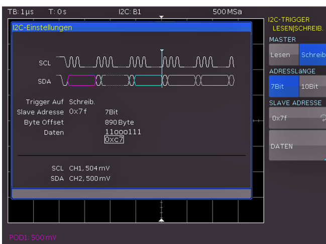
Abb. 12.7: I2C LESEN/SCHREIB Triggermenü
