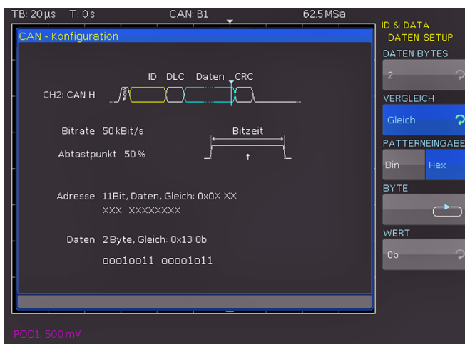
Abb. 12.19: CAN Daten Triggernmenü
