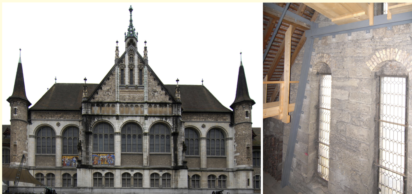
Bild 6. Erdbebenertüchtigung des Landesmuseums in Zürich: Ansicht an die Längsgiebelwand der Ruhmeshalle (links), Stahlrahmen auf der Innenseite der Längsgiebelwand zur Sicherung quer zur Wandebene (rechts).
