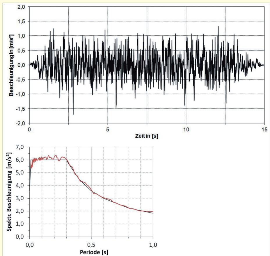
Bild 10. Spektrenkonformer Beschleunigungszeitverlauf (oben) und Gegenüberstellung des Zielspektrums mit den gemittelten Antwortspektren aus sieben Zeitverläufen;
