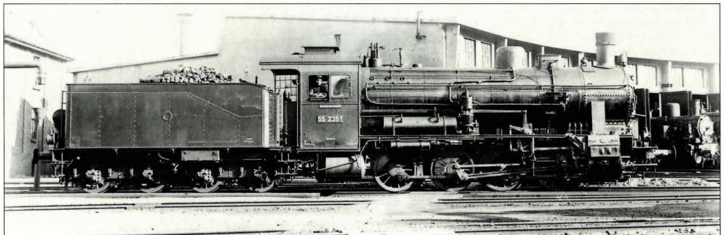
Bild 14: Die 55 2351, eine der G 9-Lokomotiven mit Lentz-Ventilsteuerung. Auf dem rechten Laufblech Knorr-Luftpumpe und Hauptluftbehälter. Foto: Sammlung Weisbrod
