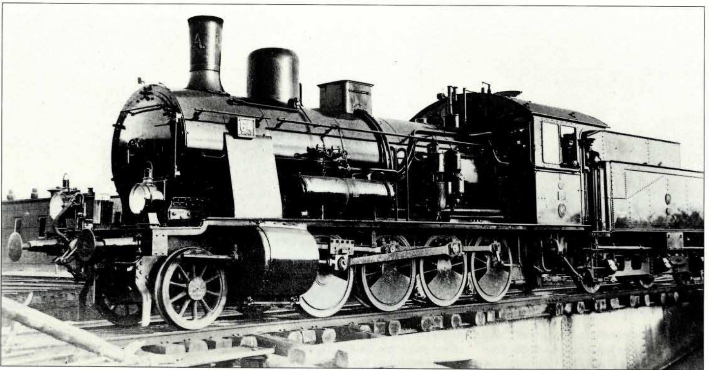
Bild 9: Die G 7 2 aus der Nachbauserie von 1917 (64 WARSCHAU), die als 4464 KÖNIGSBERG von der DRG die Betriebsnummer 56 003 erhielt. Die innenliegende Allan-Steuerung gestattet den freien Blick auf das Triebwerk. Foto: Sammlung Weisbrod
