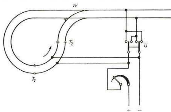
Bild 10 Schaltung 1 Einfache Kehrschleifenschaltung für eine Fahrrichtung
