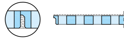
FF: je eine Stirn- und Längskante FF / SK
