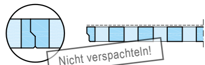
linear: umlaufender Stufenfalz
