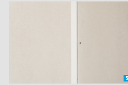
5 Gipsplatten mit ca. 5 mm Abstand montieren
