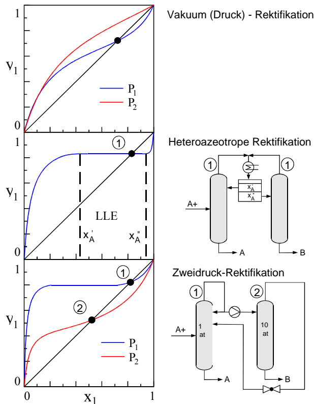
Abb. 9: Trennung der Systeme Ethanol/H 2 O (Vakuumrektifikation), H 2 O/Butanol-1 (Heteroazeotrope Rektifikation) und THF/H 2 O durch Zweidruckrektifikation
