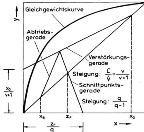
Abb. 6: Gleichgewichtsdiagramm mit Verstärkungs-, Abtriebs- und Schnittpunktgeraden
