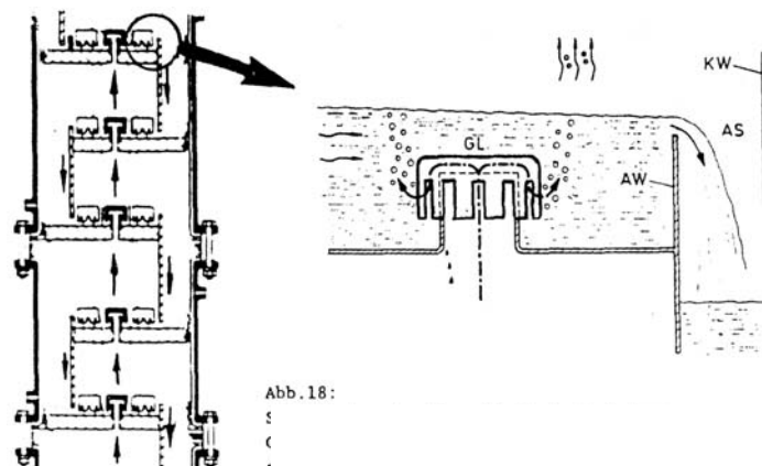
Abb. 14: Stoffströme in einer Glockenbodenkolonne
