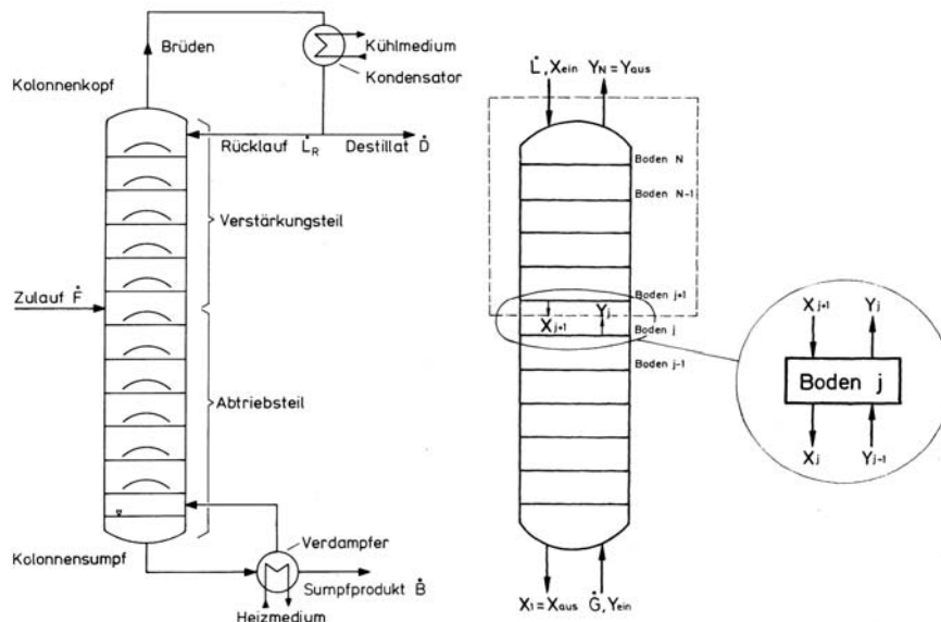
Abb. 3: Schematische Darstellung einer kontinuierlich arbeitenden Kolonne mit Verstärkersäule, Feedboden, Abtriebssäule, Rückflussteiler am Kopf der Kolonne und Verdampfer im Kolonnensumpf
