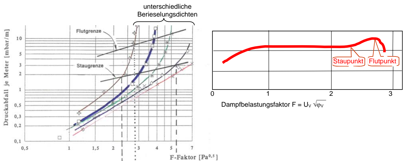
Abb. 16: spezifischer Druckverlust und Anzahl der theoretischen Trennstufen/m (NTU/m) als Funktion des F-Faktors (F = Dampfgeschwindigkeit im freien Querschnitt * \sqrt{\text{Dampfdichte}} )
