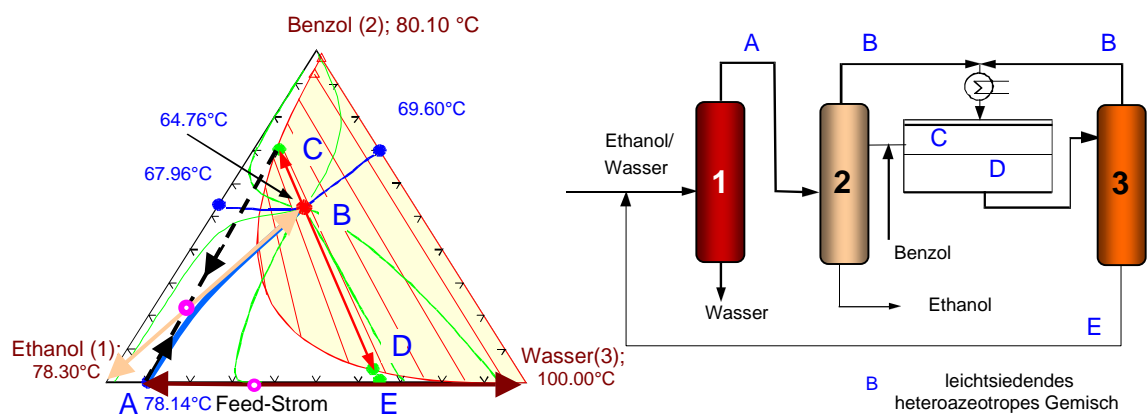
Abb. 11: Kolonnenkonfiguration und Phasengleichgewicht des ternären Systems Ethanol–Wasser–Benzol
