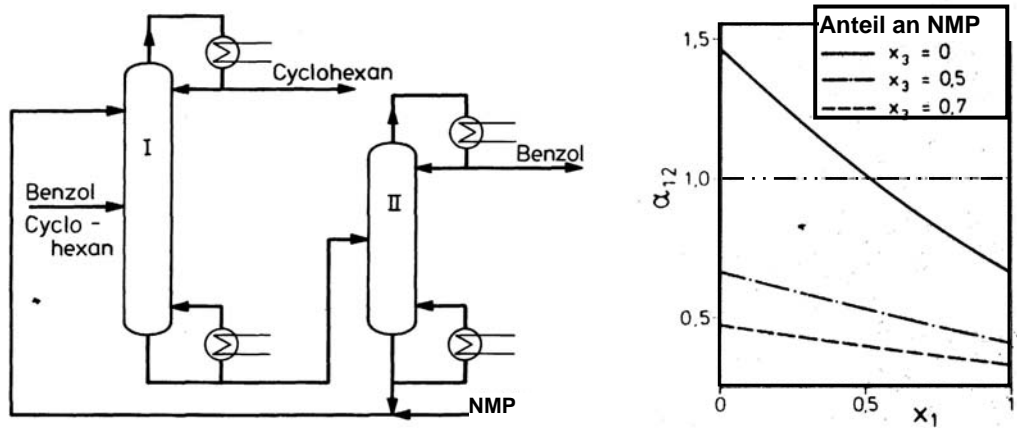
Abb. 10: Kolonnenkonfiguration der extraktiven Rektifikation am Beispiel des Systems Benzol–Cyclohexan–NMP sowie der Einfluss von Anilin auf das Dampf–Flüssig–Gleichgewicht des Systems Benzol–Cyclohexan (1 – Benzol; 2 – Cyclohexan; 3 – Anilin)
