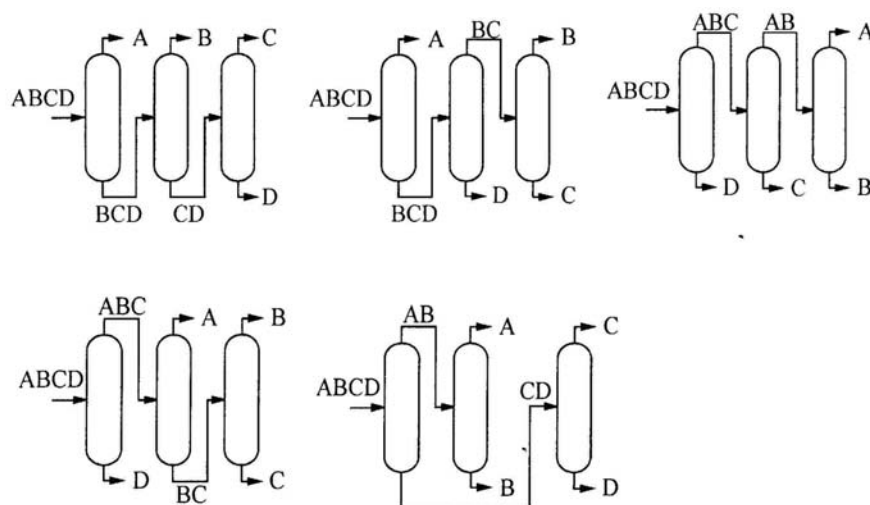
Abb. 12 Rektifikationssequenzen für die Auftrennung von Vier-Komponentengemischen
