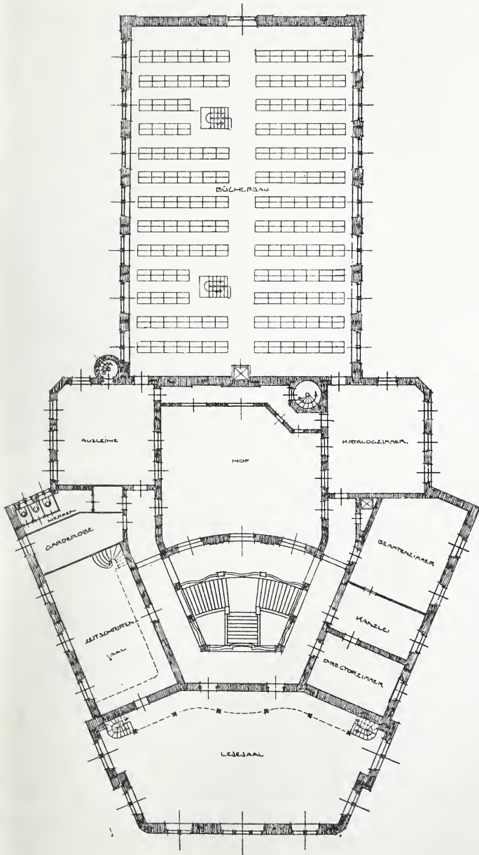
Universitätsbibliothek Gießen. Obergeschoß. Maßstab 1 : 400 = 2 1/2 mm : 1 m.
