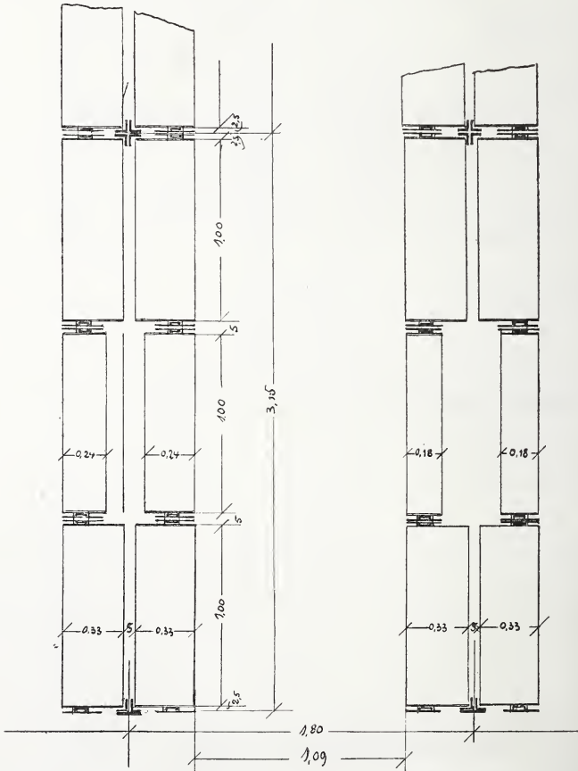
Danziger Büchergestell Steeg. Fig. 4. Grundriß eines Binderfeldes.
