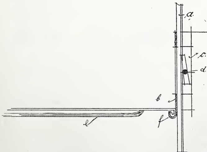
Fig. 3. Vorderansicht des Schildes mit Boden.
