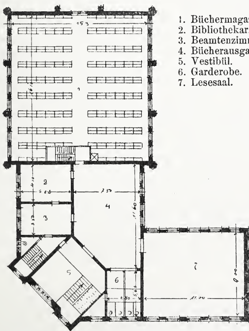
Stadtbibliothek Danzig. Grundriß II: Obergeschoss. Maßstab 1 : 400 = 2\frac{1}{2} mm : 1 m.
