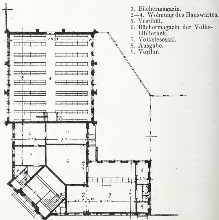
Stadtbibliothek Danzig. Grundrifs I: Erdgeschoss.
