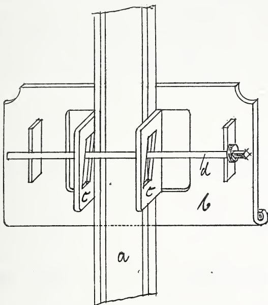
Danziger Büchergestell Steeg. Fig. 2. Seitenansicht des Schildes.
