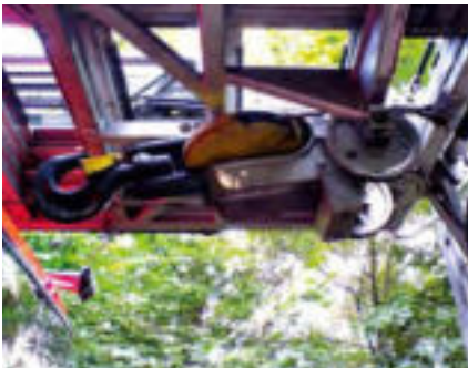
Die Kraneinrichtung des Hubrettungsfahrzeuges – die lose Rolle und die beiden festen Rollen wirken zusammen als Flaschenzug.
