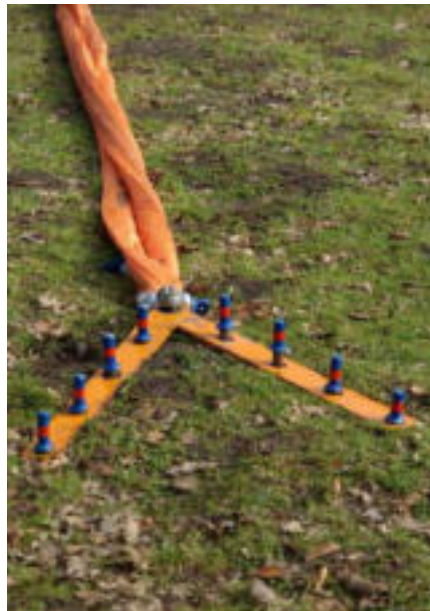
Erdanker als Festpunkt
