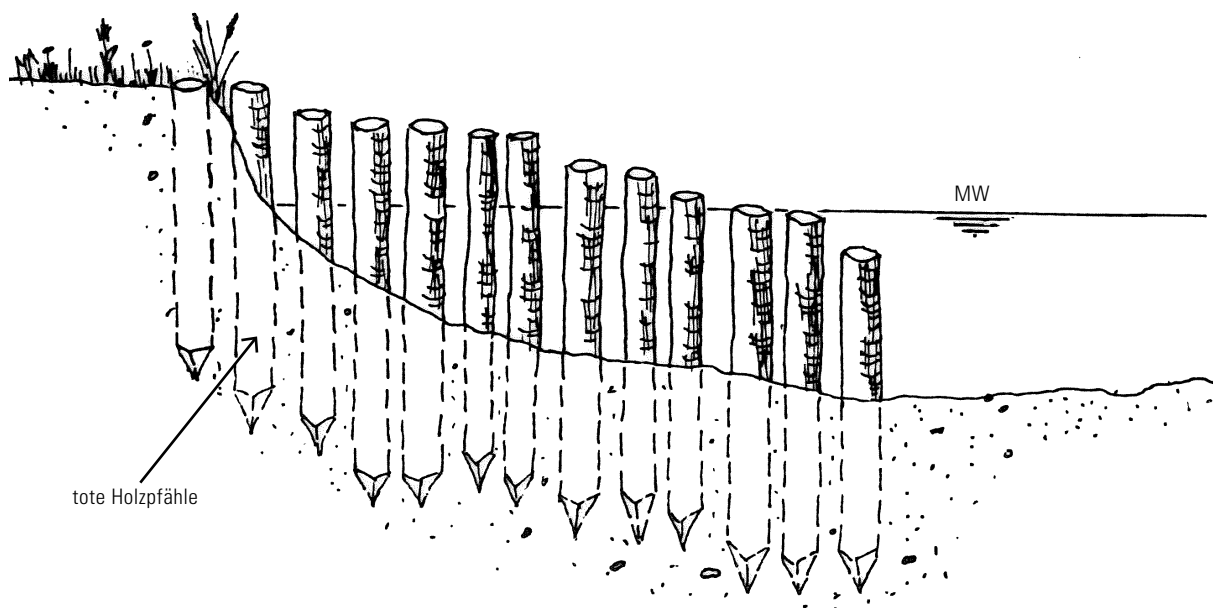
Nicht austriebsfähige Pfahlbuhne
