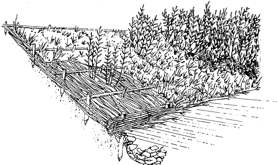
Spreitlage mit Querstangen- und Steinfußsicherung mit fortschreitender Vegetationsentwicklung
