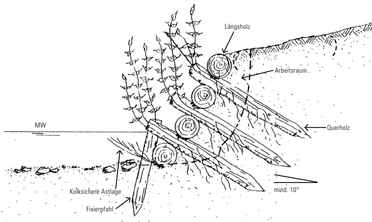
Einwandige Krainerwand mit zusätzlichem Befestigungspfahl und Astlage unter dem ersten Längsholz (Kolk-schutz bei feinen Böden)
