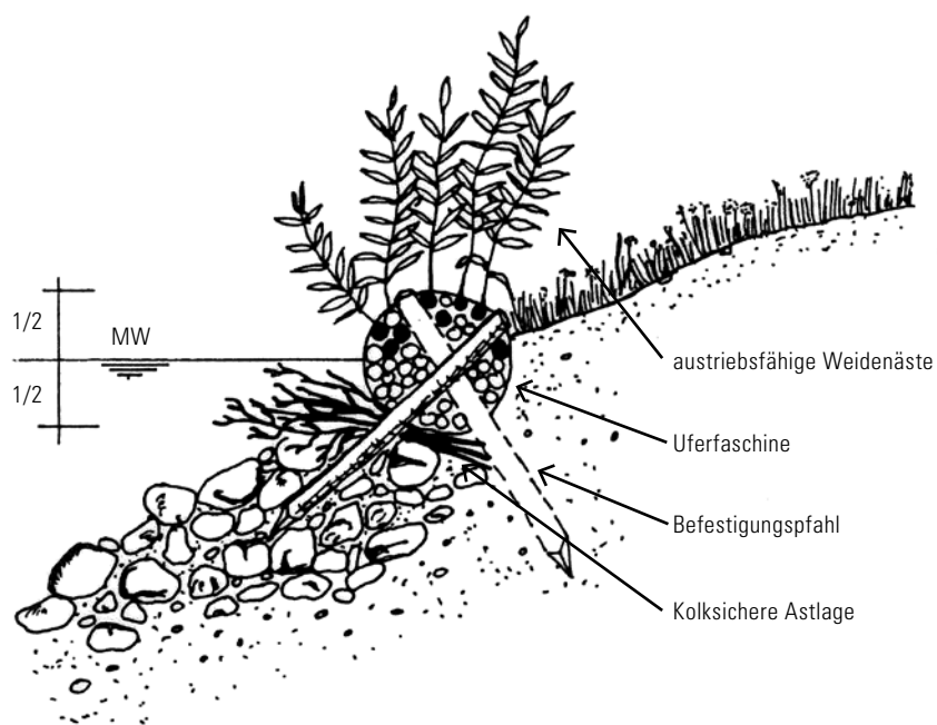
Eingebaut lebende Faschine mit Austrieb auf zusätzlicher Astlage
