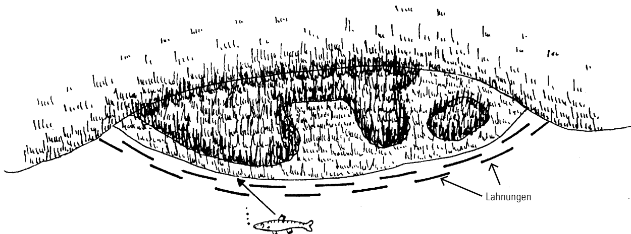
Anordnung von Lahnungen vor einem Schilfbestand
