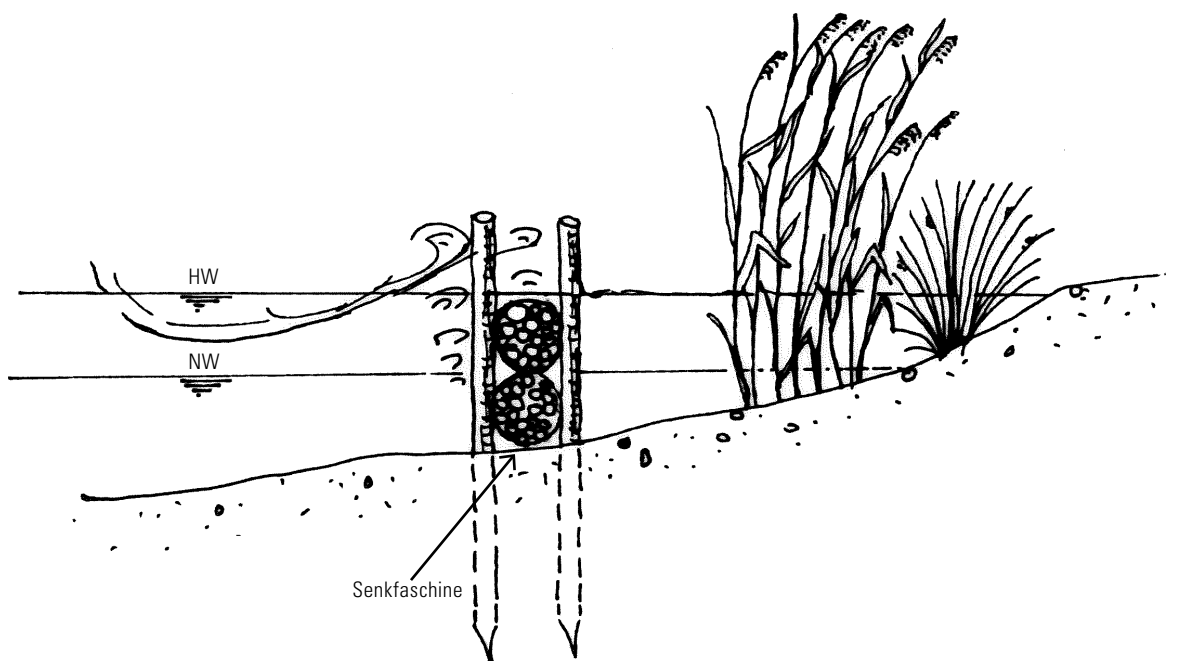
Lahnung aus zwei Senkfaschinen ohne Querfaschinen zwischen den Pfahlreihen
