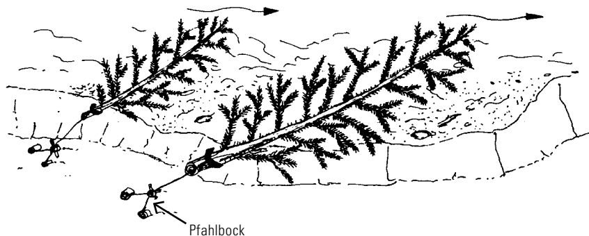
Raubäume vom Ufer abgehängt
