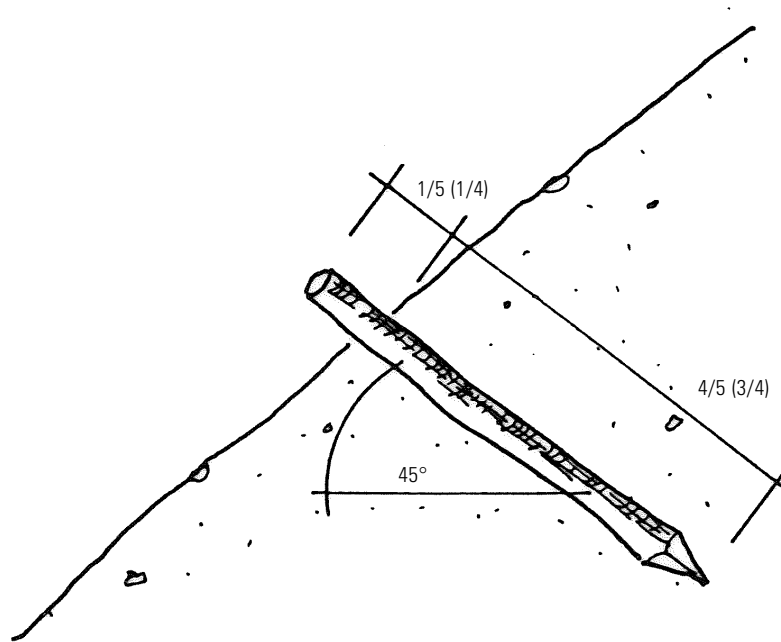
Steckholz fachgerecht eingebaut
