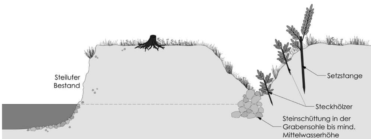
Schlafende Ufersicherung mit Weidensteckhölzern und -setzstangen
