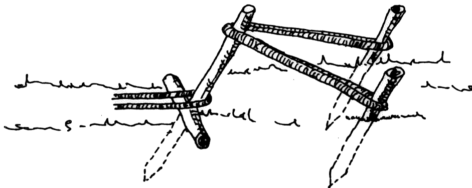
Pfahlbock zum Befestigen von Raubäumen am Ufer
