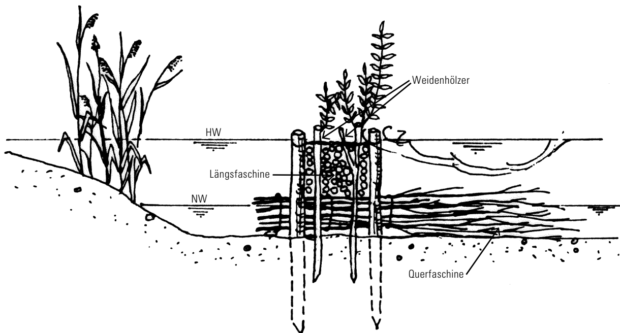
Einfache Lahnung mit lebenden Weidenhölzern
