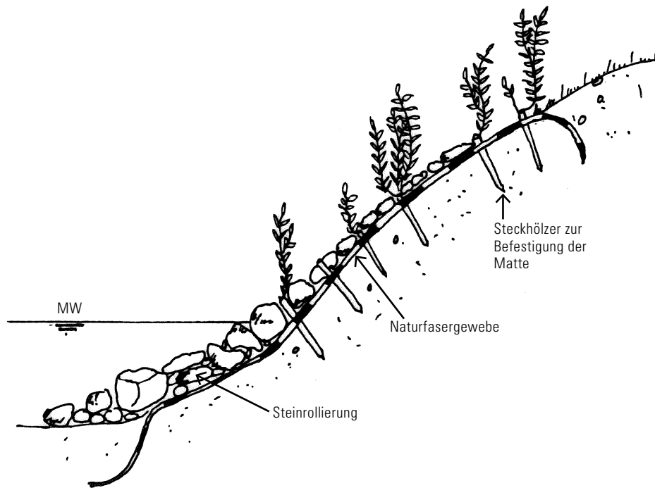
Böschungsschutzmatte mit Weidensteckhölzern und Rollierung
