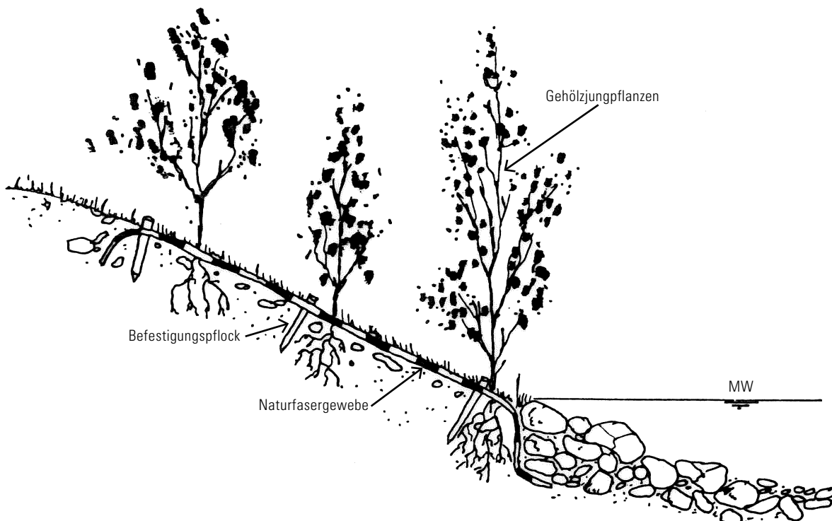
Böschungsschutzmatte mit Gehölzjungpflanzungen
