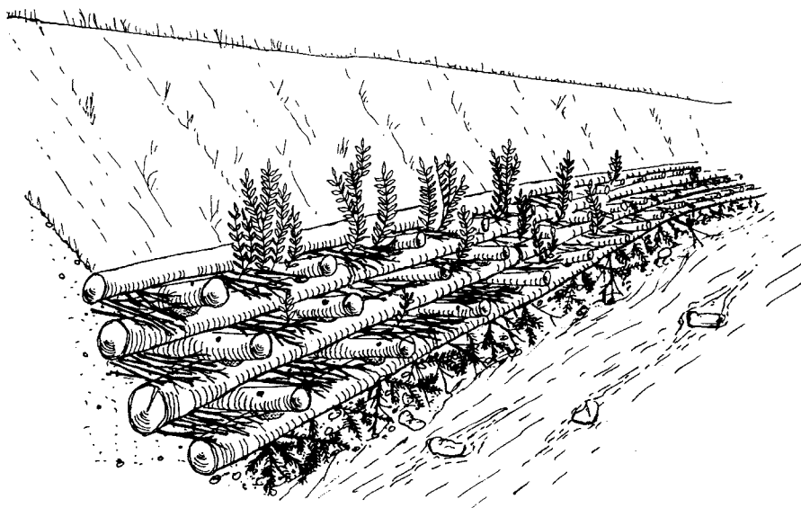
Krainerwand mit beginnender Vegetationsentwicklung
