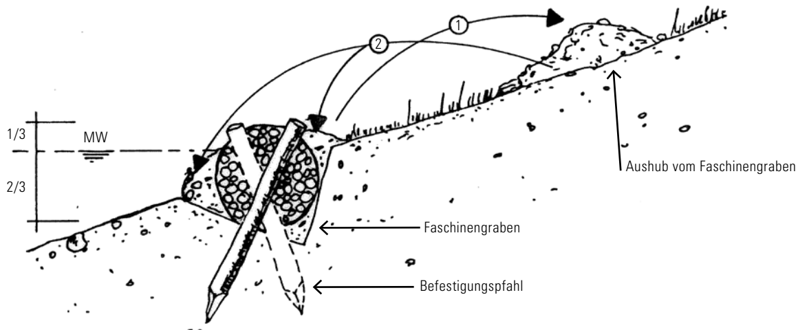
Bauablauf beim Einbau einer Faschine
