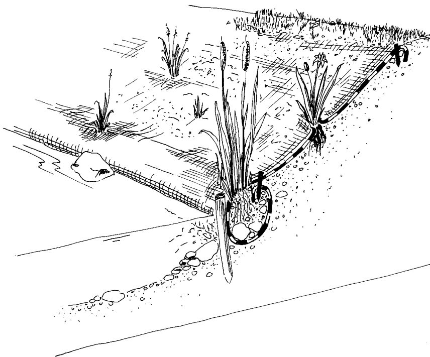
Röhrichtwalze mit Böschungsschutz kombiniert
