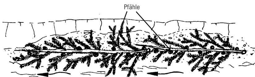
Raubaumkette mit Pfahlreihen
