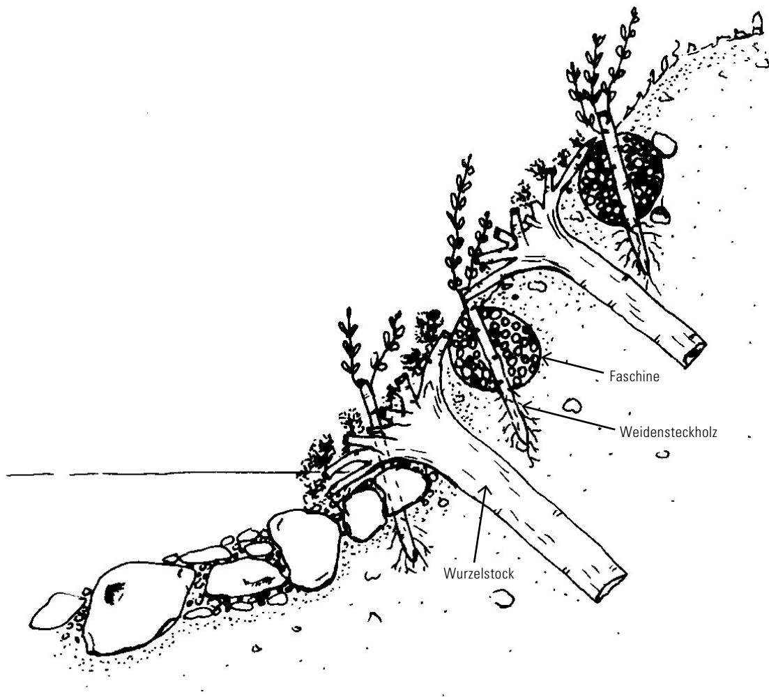
Wurzelstöcke zur Ufer-/Böschungssicherung in Kombination mit Faschinen und kräftigen Weidensteckhölzern
