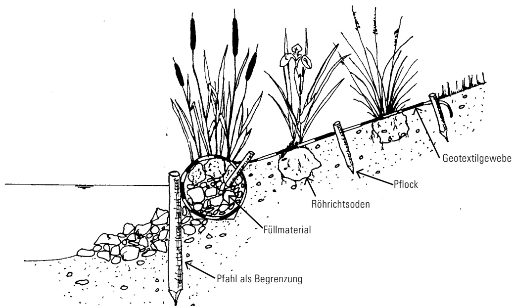
Vegetationswalze mit nachfolgender, geotextilgesicherter Ballenpflanzung
