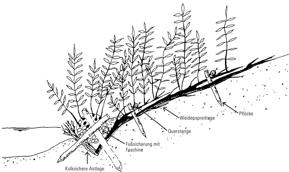
Spreitlage mit Faschine als Fußsicherung mit beginnender Vegetationsentwicklung
