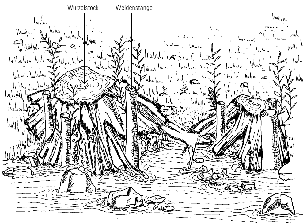
Am Ufer eingebaute Wurzelstöcke mit Weidenstangen
