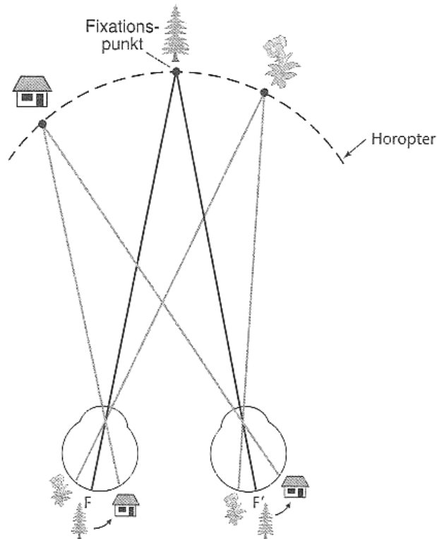
4.25 Korrespondierende Netzhautpunkte und Horopter Bei Fixierung eines Gegenstandes (Tanne) mit beiden Augen fallen die Abbilder desselben in beiden Augen auf korrespondierende Netzhautpunkte, die mit derselben Stelle im visuellen Cortex verbunden sind. Dasselbe trifft zu für alle Objekte, die auf einem gedachten Kreis, dem Horopterkreis, liegen, der laut Definition durch den Fixationspunkt und den optischen Mittelpunkt beider Augen geht (aus Gründen der Übersichtlichkeit ist dies in unserer Darstellung nicht berücksichtigt).
