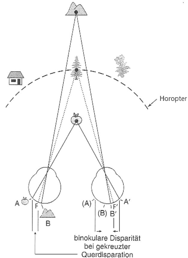
4.26 Zusammenhänge zwischen Querdisparation und binokularer Disparität in Abhängigkeit von der Lage des Beobachtungsobjektes vor oder hinter dem Horopter. Die korrespondierenden Netzhautpunkte A-A' und B-B' im gleichen Auge erhält man, indem man gedanklich beide Netzhautquerschnitte übereinander legt.
