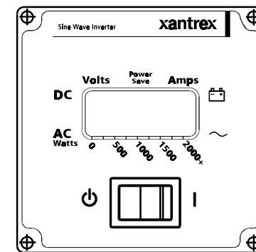
Figure 7. Panneau de contrôle du Sine Wave
