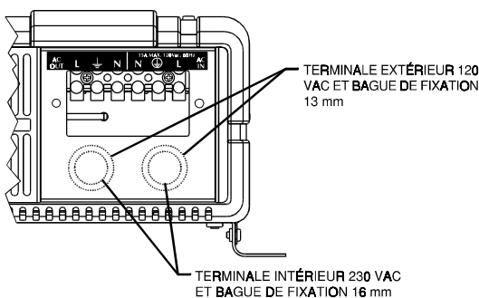
Figure 3. Branchement de l'alternatif sur le convertisseur version bornier à vis
