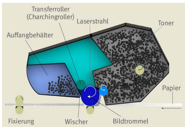
Abb. 38 Prinzip des Laserdruckers
