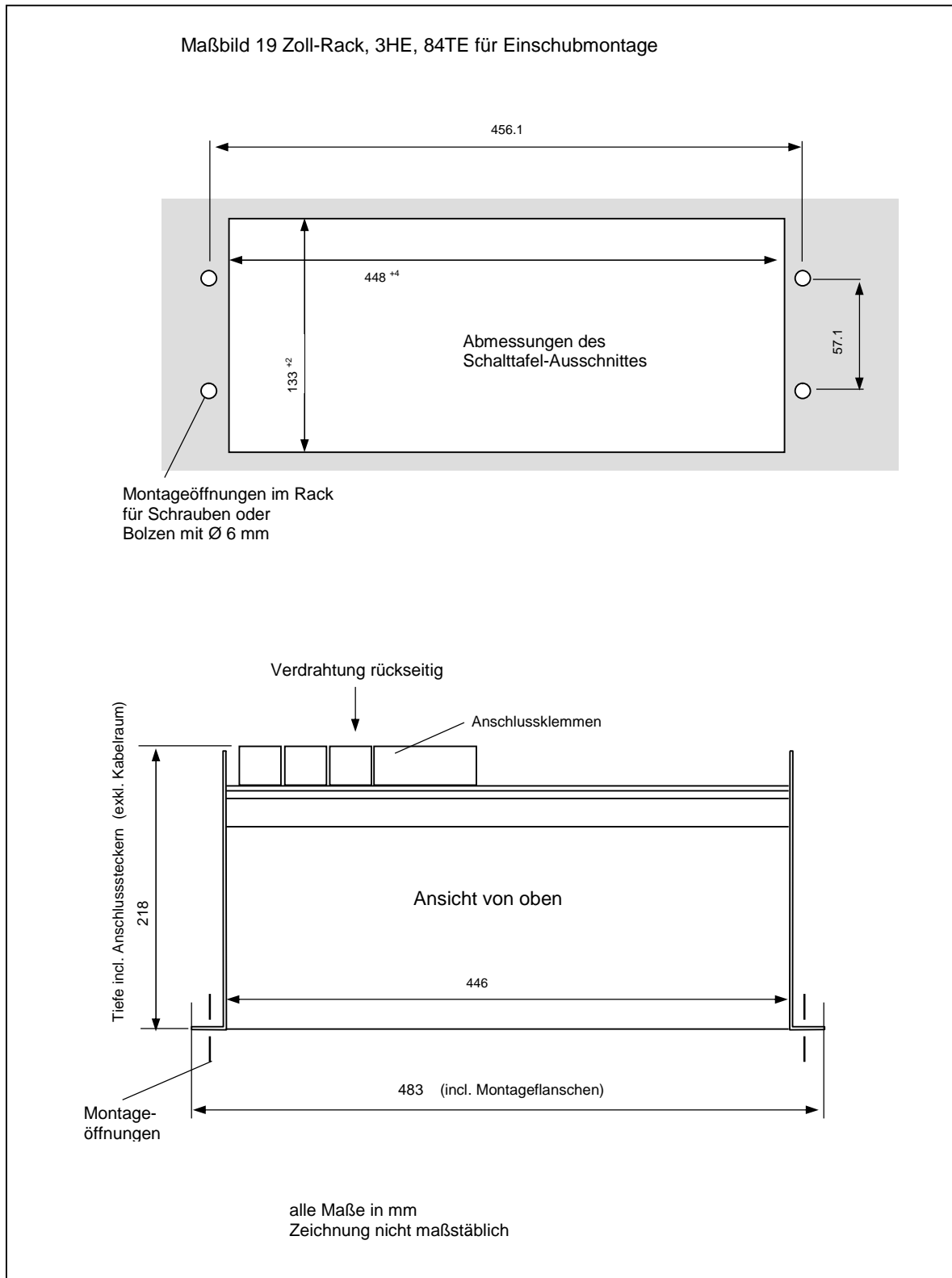
Abbildung 8: Abmessungen des Systems E16E446
