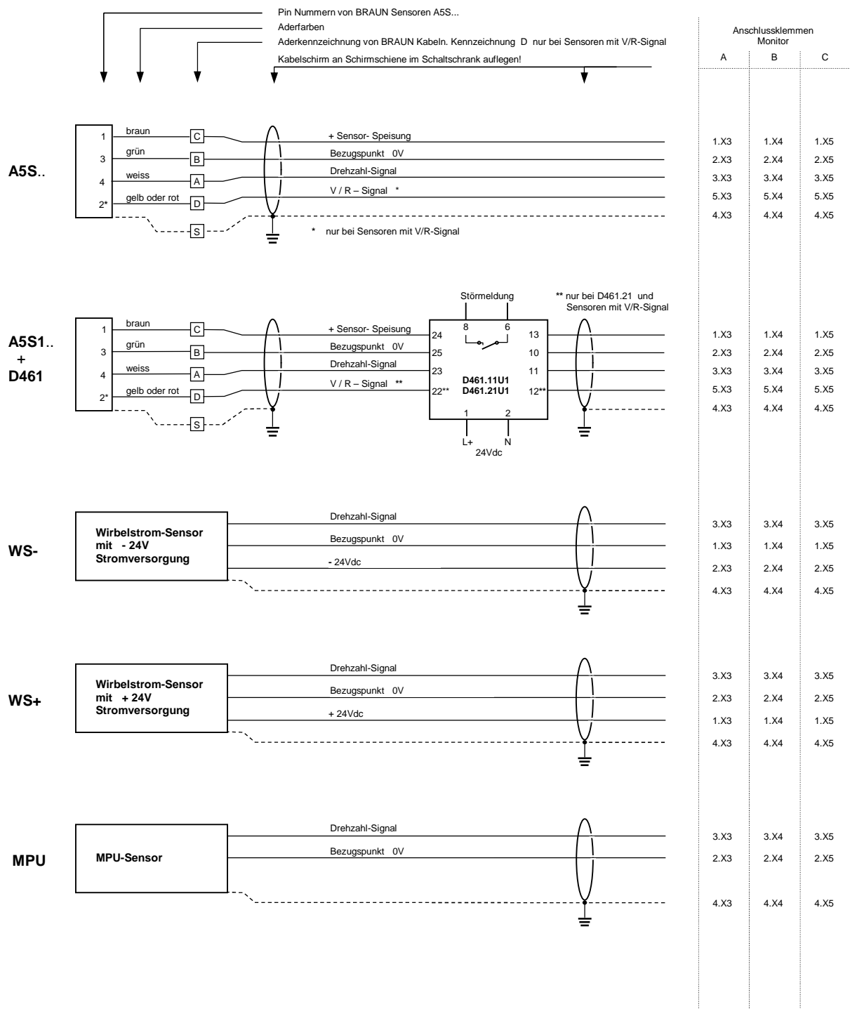
Abbildung 6: E16x446 System-Anschlussplan 3 von 3
