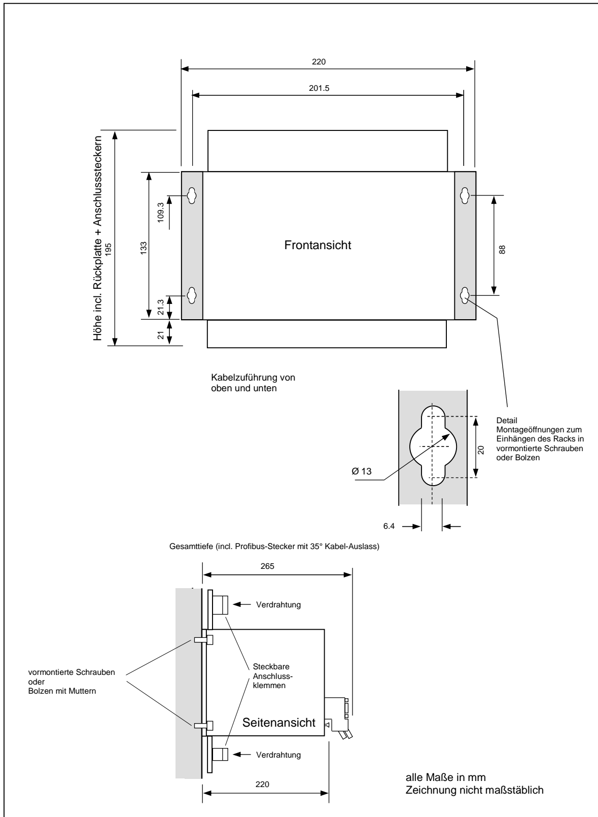
Abbildung 7: Abmessungen des Systems E16A446
