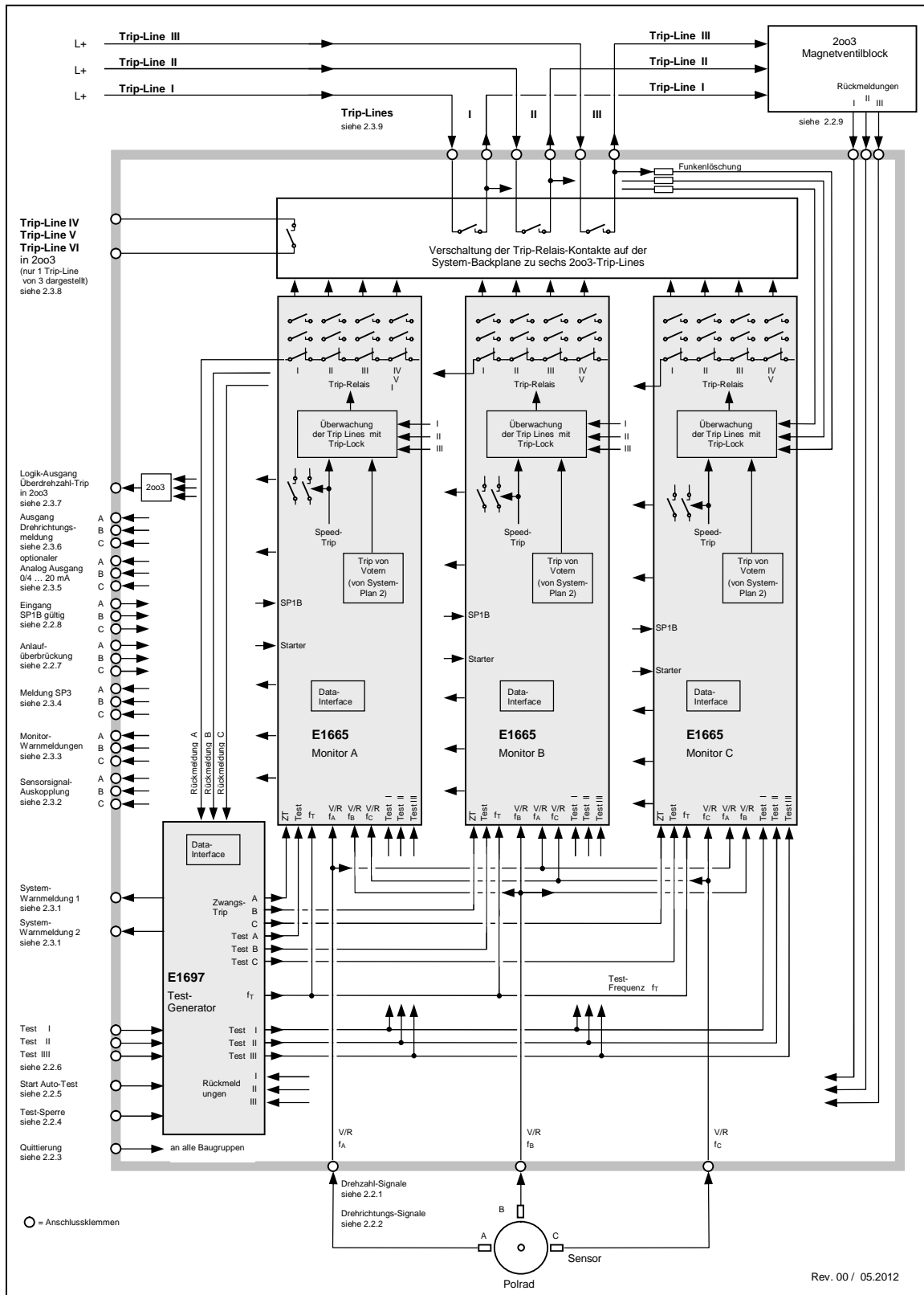
Abbildung 2: E16x446 Systemaufbau 1 von 2 - Drehzahl und Testgenerator
