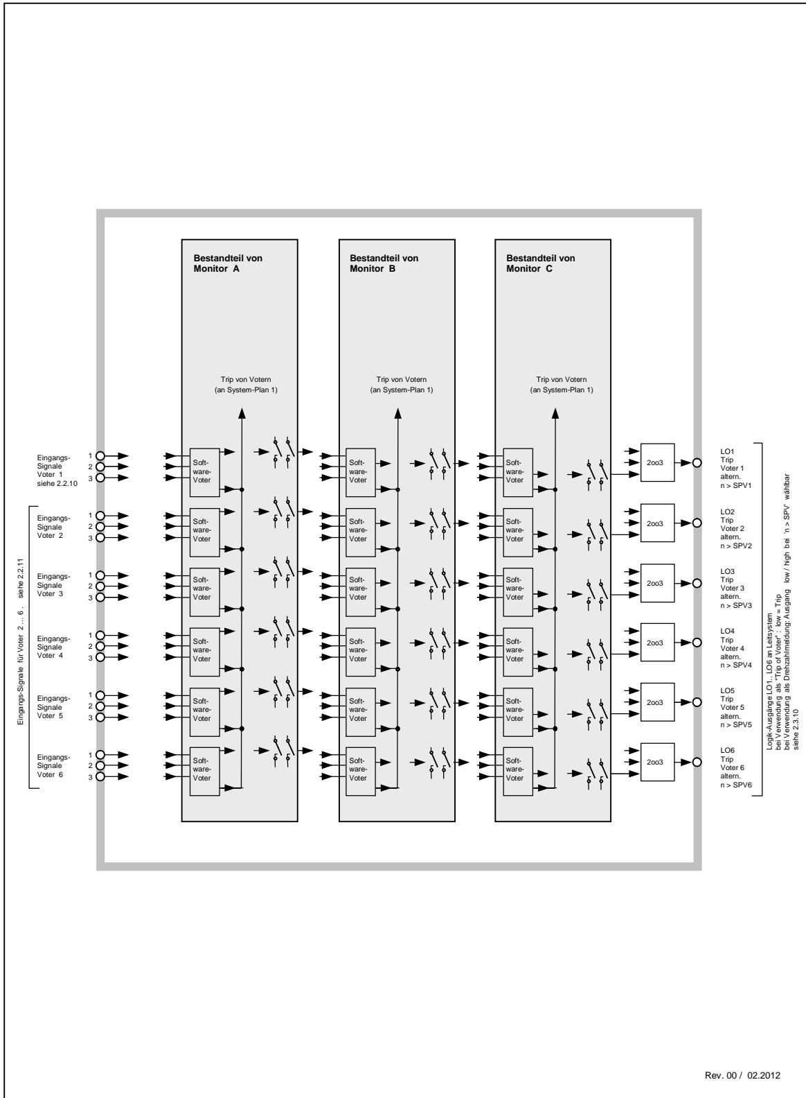
Abbildung 3: E16x446 Systemaufbau 2 von 2 - Voter
