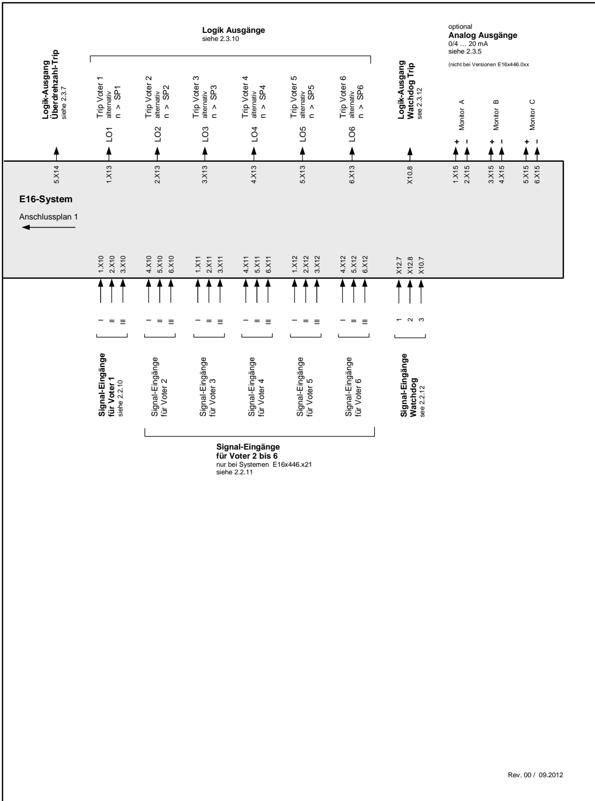
Abbildung 5: E16x446 System-Anschlussplan 2 von 3
