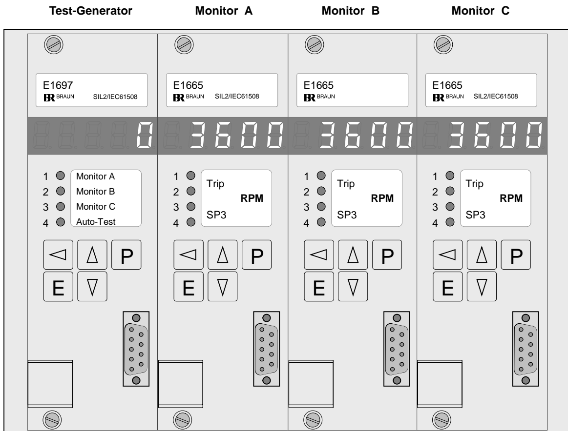
Abbildung 1: E16x446 System Frontansicht
