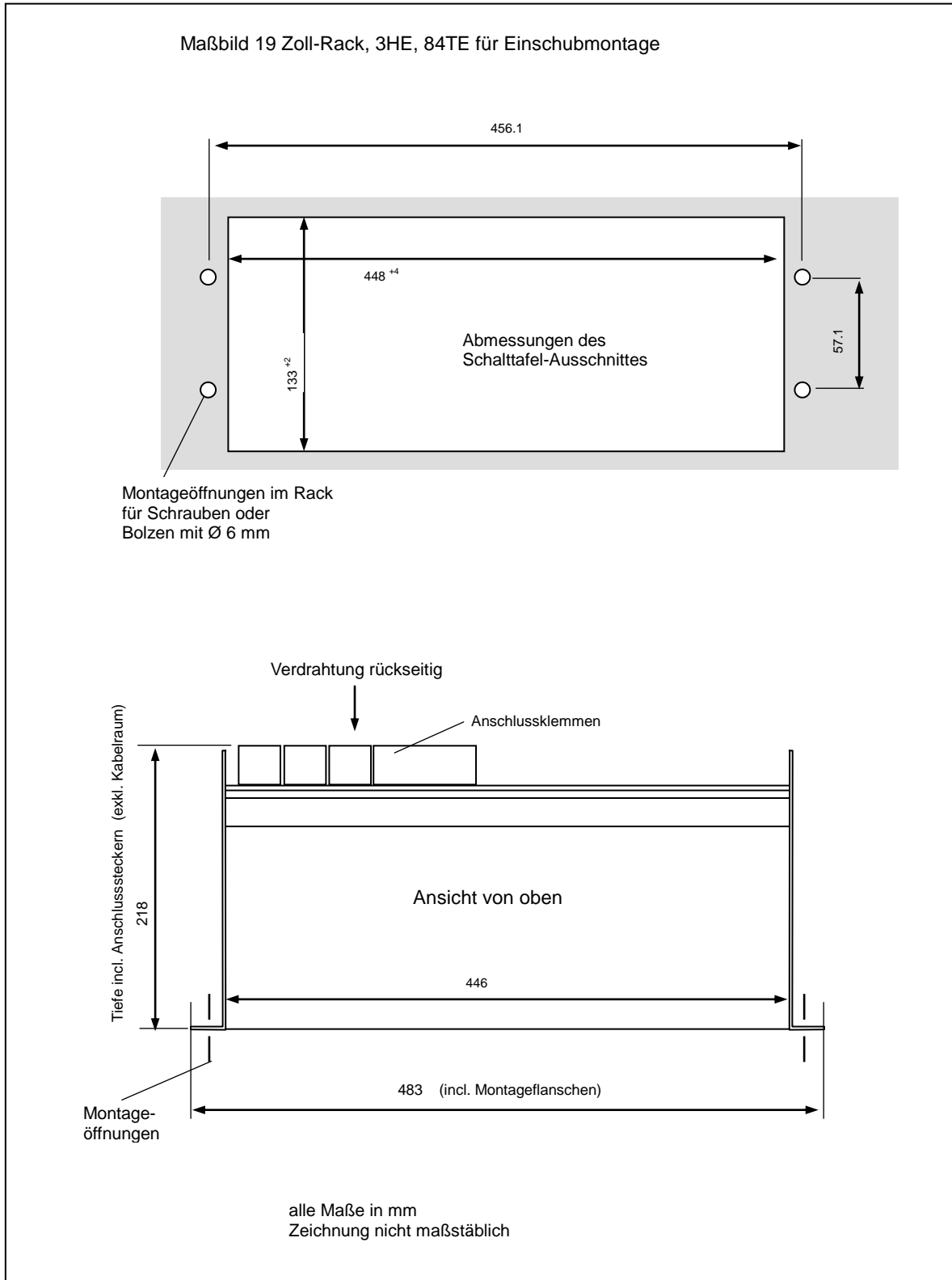
Abbildung 8: Abmessungen des Systems E16EA452
