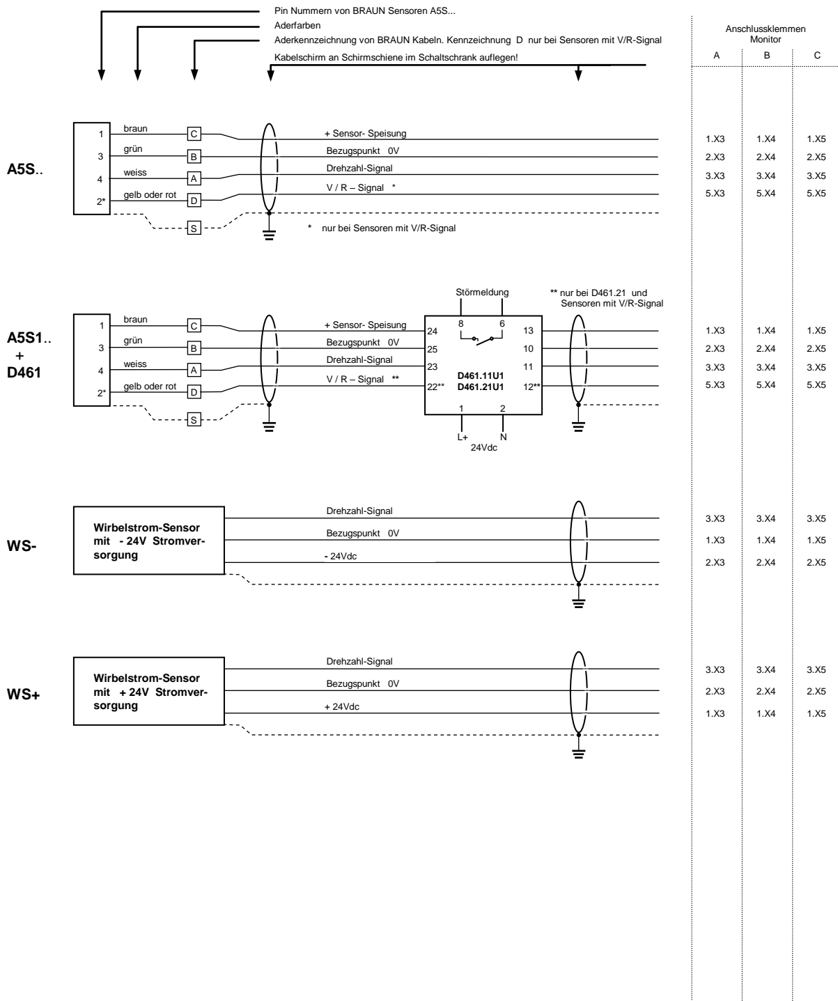
Abbildung 6: E16x452 System-Anschlussplan 3 von 3
