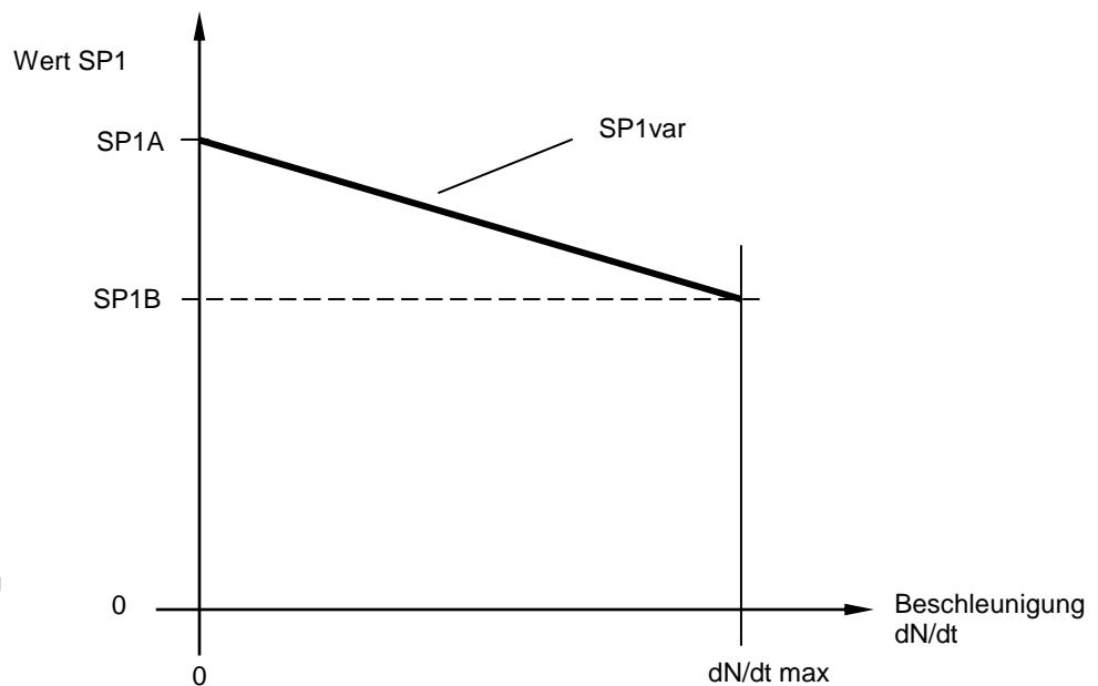
Abbildung 11: Abhängigkeit SP1 von der Beschleunigung
