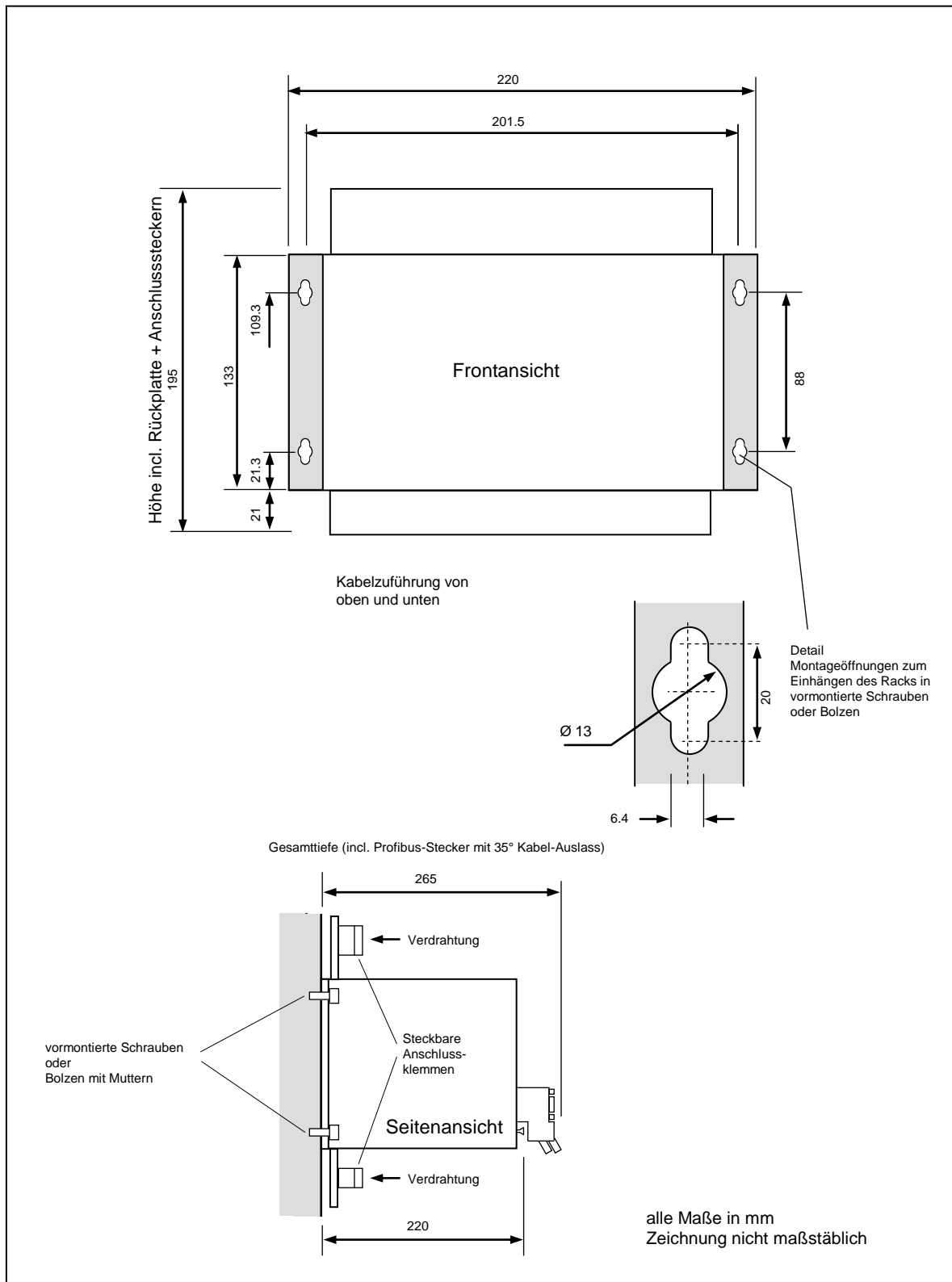
Abbildung 7: Abmessungen des Systems E16X452
