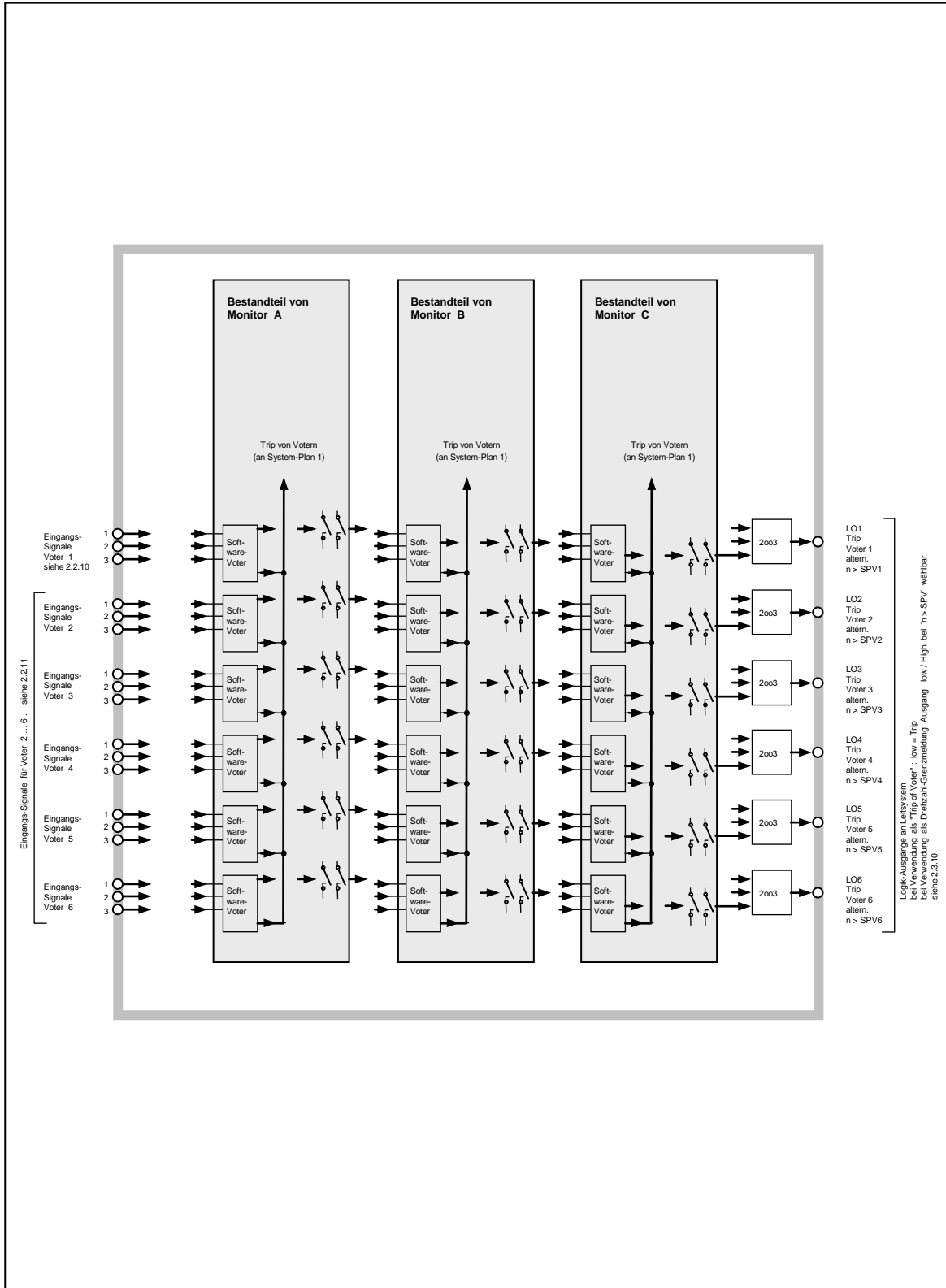
Abbildung 3: E16x452 Systemaufbau-Darstellung 2 von 2
