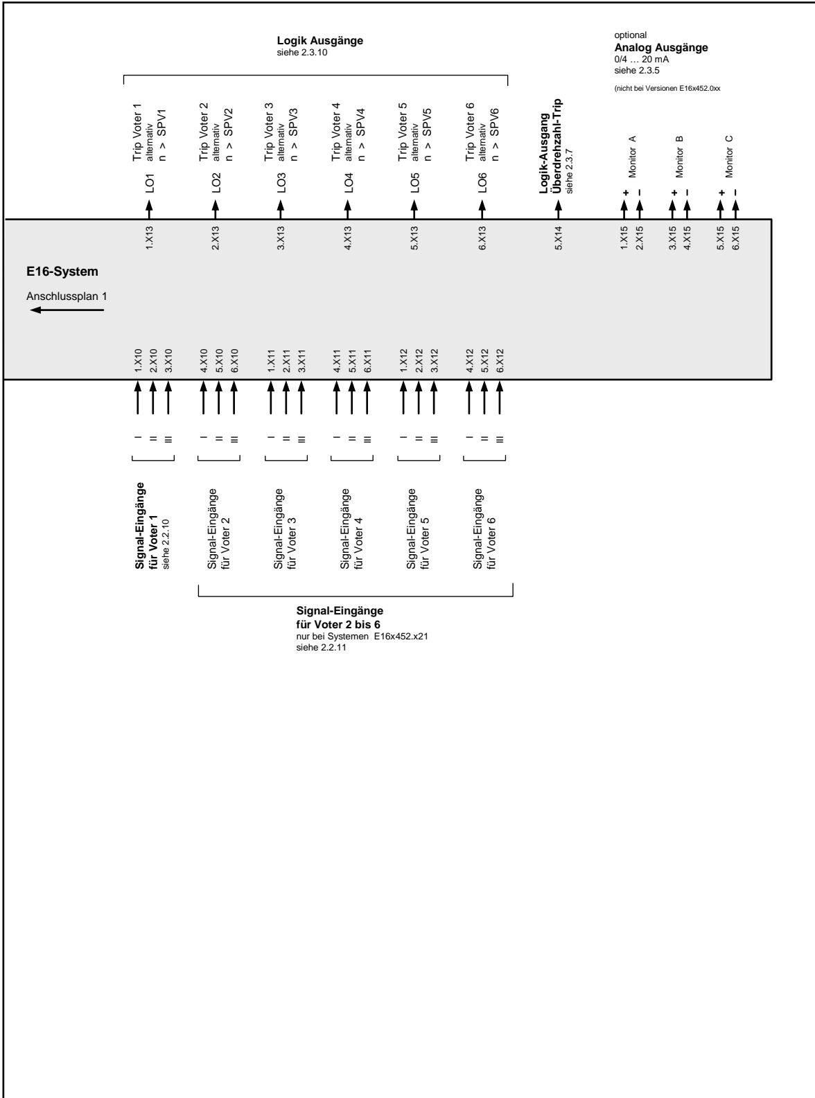
Abbildung 5: E16x452 System-Anschlussplan 2 von 3
