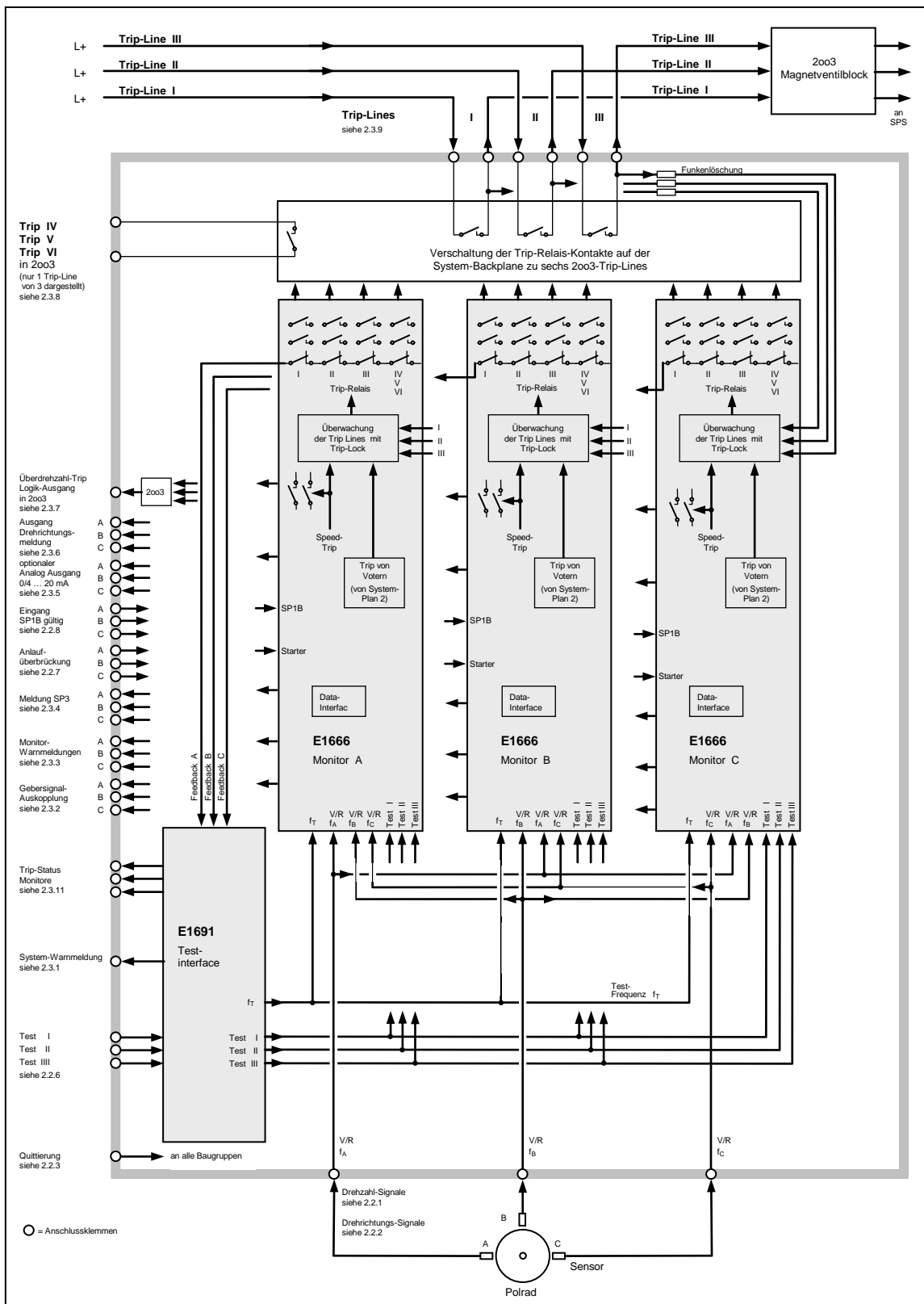
Abbildung 2: E16x452 Systemaufbau-Darstellung 1 von 2
