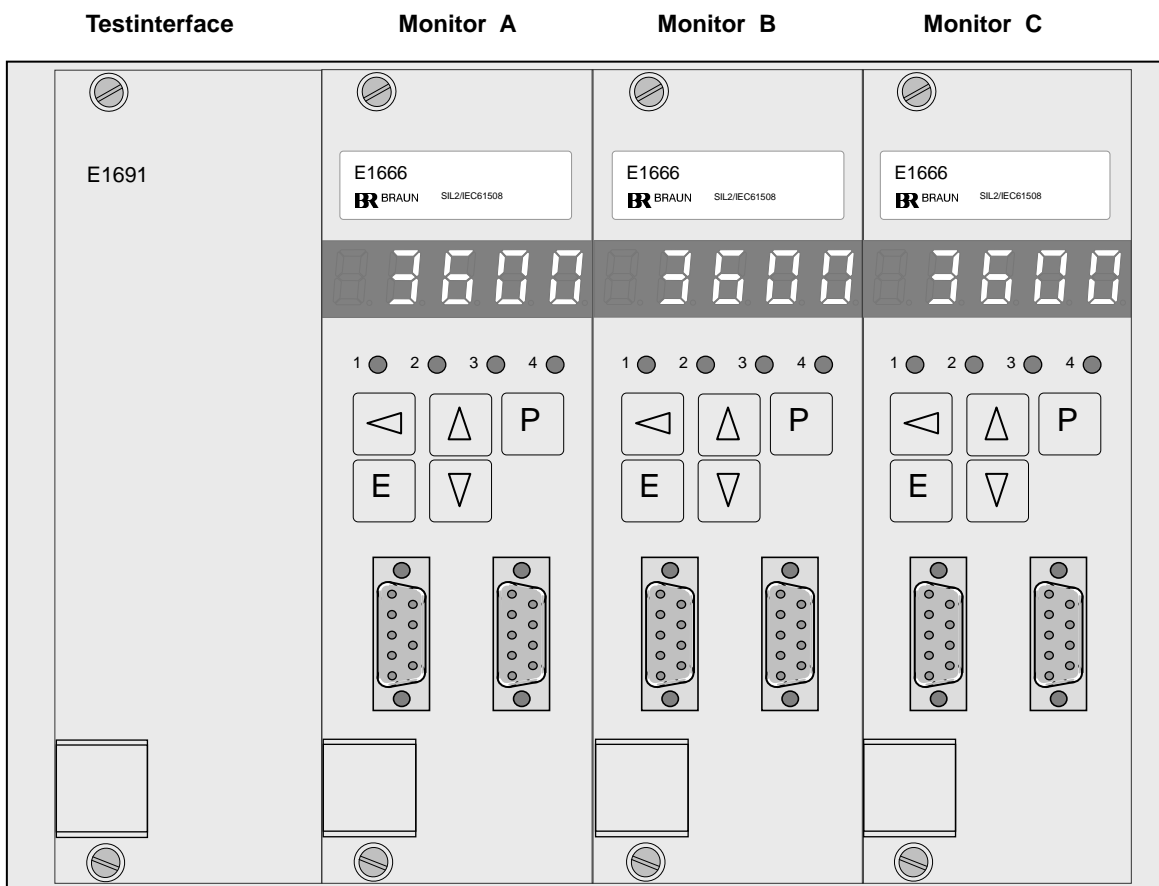
Abbildung 1: E16x452 System Frontansicht
