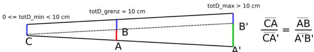
Abbildung 5.5: Anwendung des zweiten Strahlensatzes an einem Totholzstück
