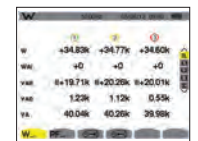
Leistungsmessung
