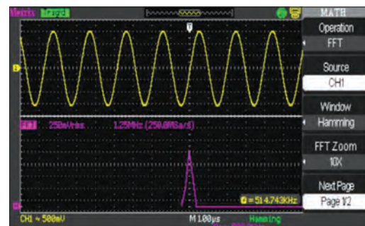
Einfache MATH-Funktionen: +/-/x/\div und FFT-Funktion in Echtzeit mit gleichzeitiger Anzeige der Kurven
