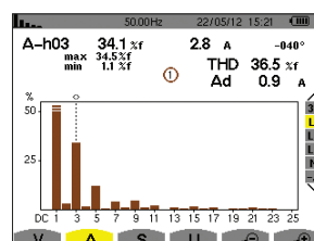
Oberschwingungsanalyse
