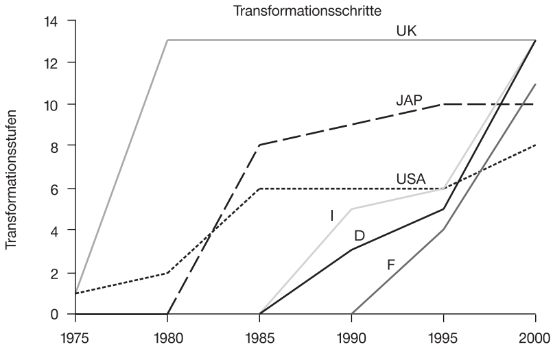
Abbildung 3-11 Ungleiche Transformationsschritte und wachsende Konvergenz
