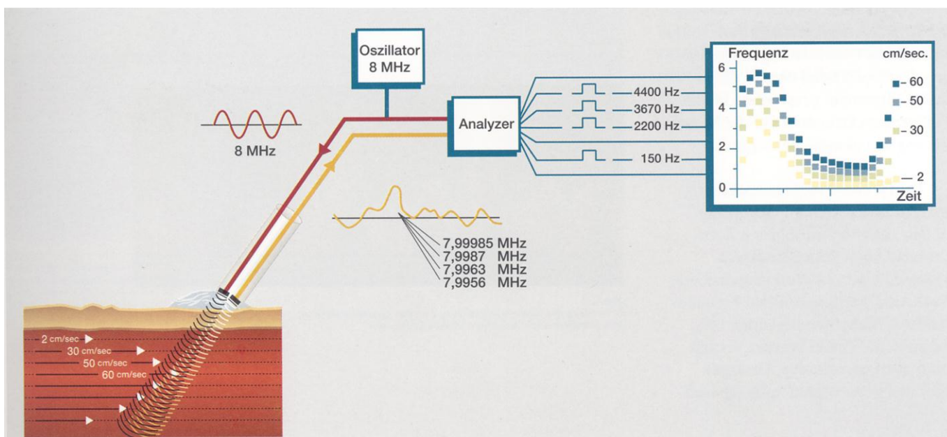
Abb. 2.3.1 Funktionsschema einer Frequenzspektrumanalyse
