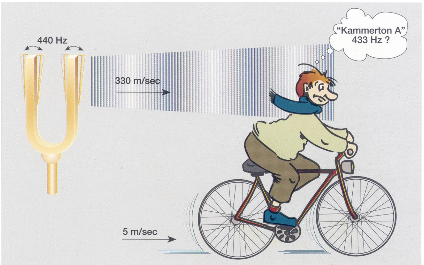
Abb. 1.3.4 Negative Frequenzverschiebung bei Relativbewegung des Empfängers vom Sender fort
