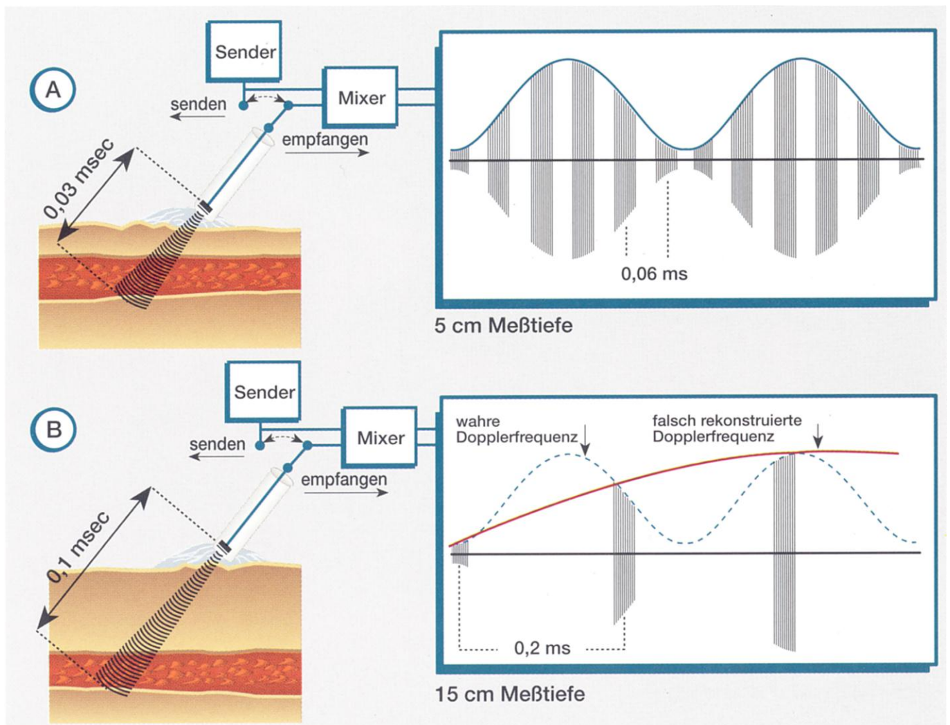
Abb. 2.4.3 Abhängigkeit der PRF von der gewünschten Messtiefe und daraus resultierende Rekonstruktion der Dopplerfrequenz
