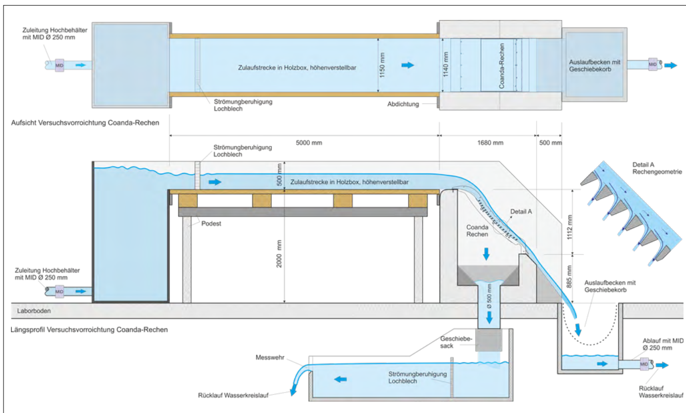
Bild 1: Versuchsvorrichtung.
