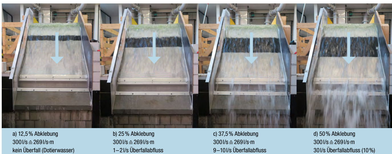
Bild 4: Ermittlung der Fassungskapazität bei schrittweiser Verlängerung der Beschleunigungsstrecke am Standardrechen der Firma Wild Metal GmbH mit 1,0 mm Spaltweite.
