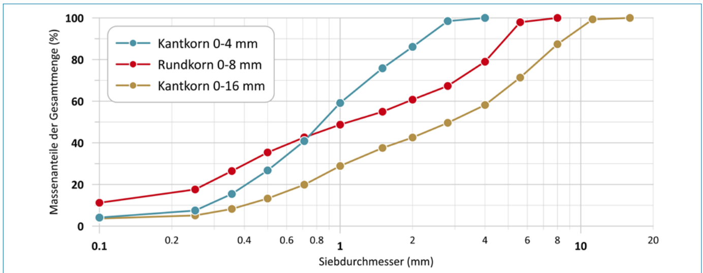
Bild 3: Gemittelte Kurven des Ausgangsmaterials.
