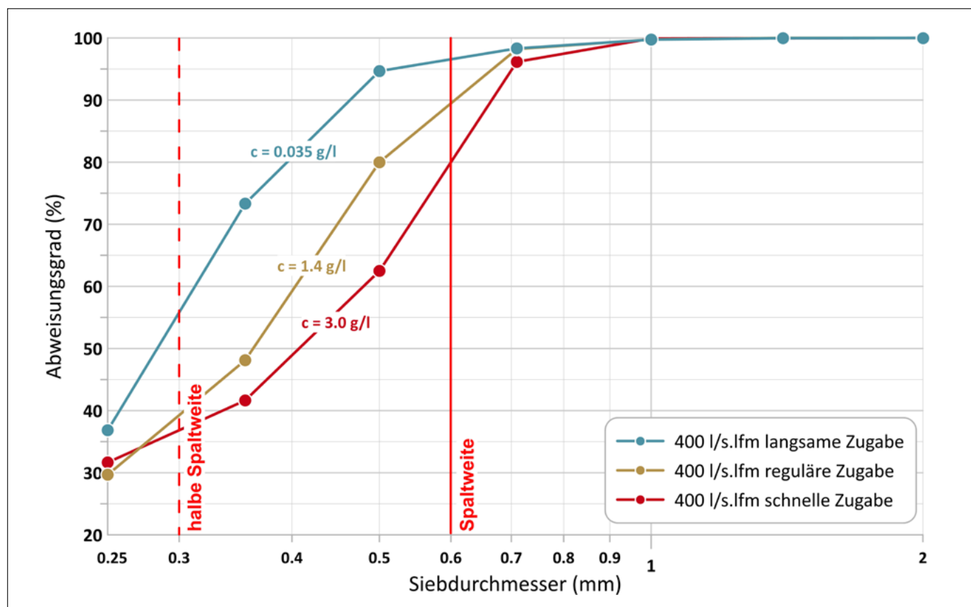
Bild 5: Vergleich der Abweisungsgrade für verschiedene Geschiebekonzentrationen bei einer spezifischen Durchflussrate von 400l/s·m in Abhängigkeit der Partikelgrösse für Kantkorn beim Standardrechen der Firma Wild Metal GmbH mit 0,6mm Spaltweite.
