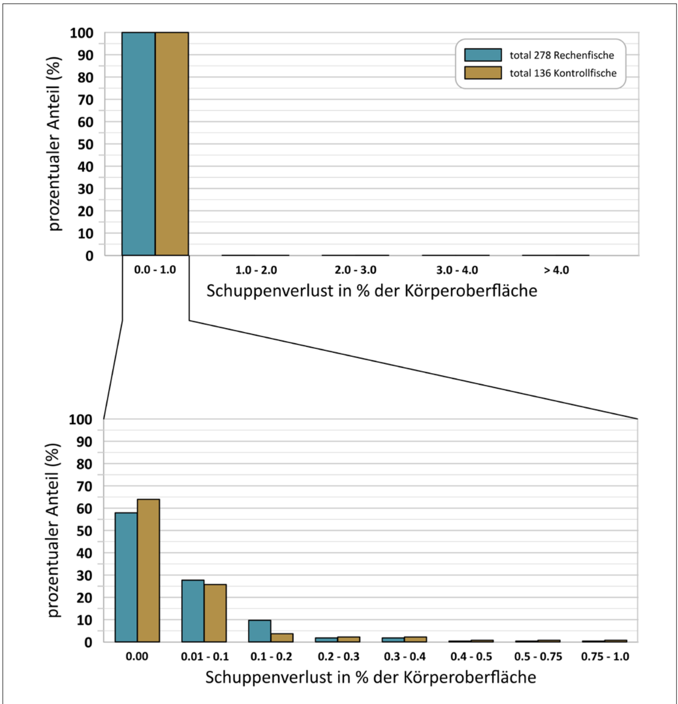
Bild 8: Gesamtheit der Schuppenverluste aller Fische bei zwei spezifischen Durchflussraten von 100 und 300l/(s·m) an den zwei Rechentypen Nr. 2 und 3 nach Tabelle 1.
