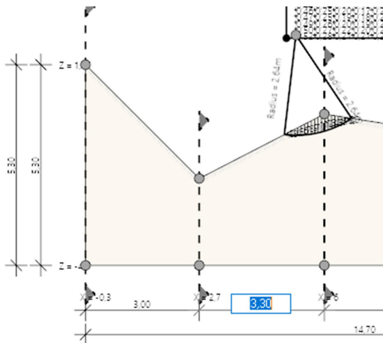
Abb.: Ändern einer Abschnittslänge durch Editieren der Maßkette in der Grafik
