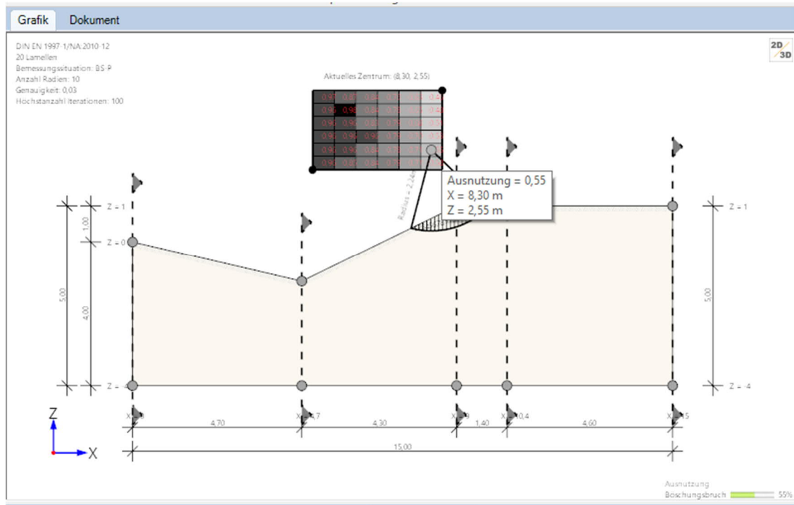
Abb.: Verschieben des Gleitkreismittelpunktes und entsprechende Darstellung der zugehörigen Ausnutzung und des Gleitkreis
