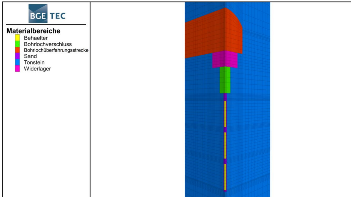
Abb. 8: Im Modell verwendete Materialbereiche zur Modellierung der thermischen Ausbreitung im Nahfeld
