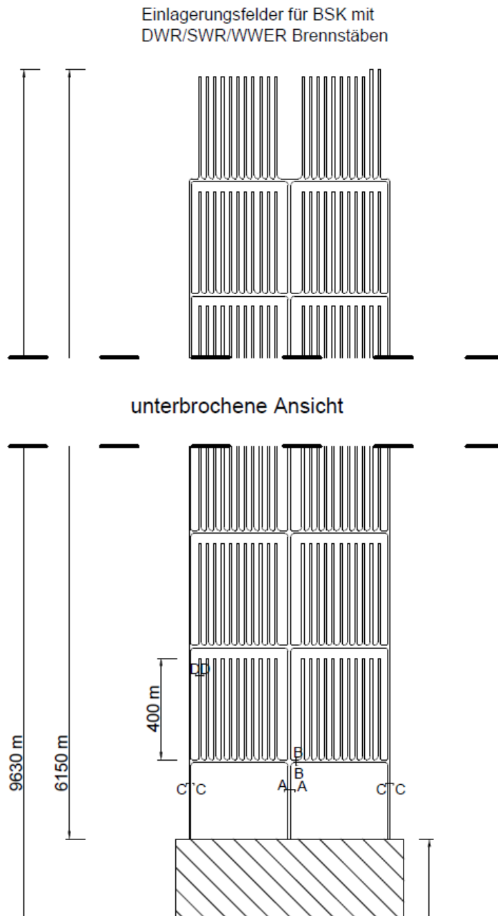
Abb. 16: Skizze des Grubengebäudeteils mit Einlagerungsbereichen für ausgediente Brennelemente (unten schraffiert: Beginn des Infrastrukturbereichs)
