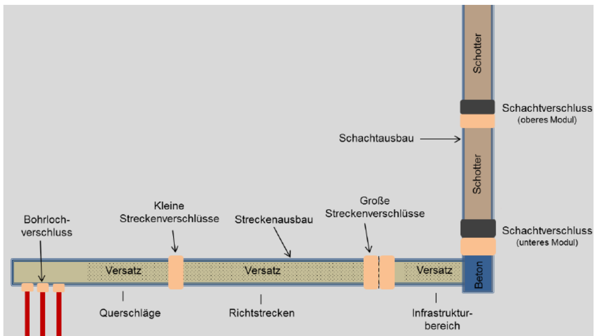
Abb. 18: Schematisierte Skizze der hydraulisch wirksamen Elemente des Verschlussystems
