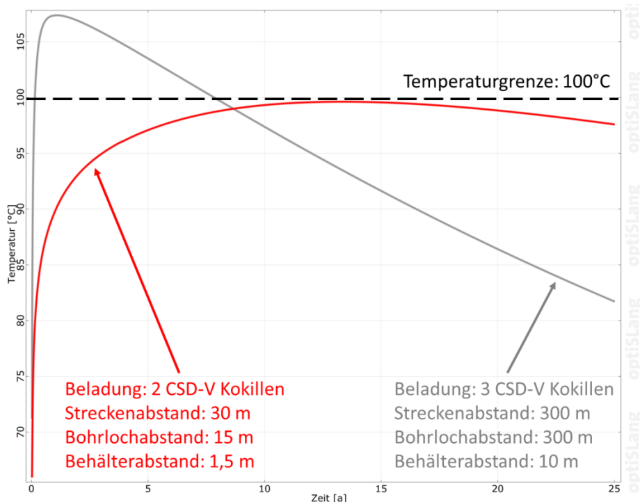
Abb. 12: Temperaturverlauf im Auslegungspunkt für verglaste Abfälle (CSD-V)
