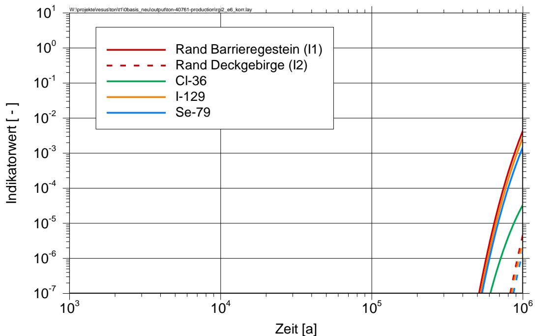
Abb. 40: Zeitverlauf der Indikatoren I1 und I2 am Rand des Barrieregesteins und in der Modelleinheit S1 für den Basisfall
