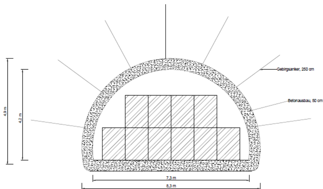
Abb. 15: Skizze der Einlagerungsstrecke für Brennelementstrukturteile (s. Abb. 16 für die Lage der Strecke anhand der Querschnittbezeichnung)
