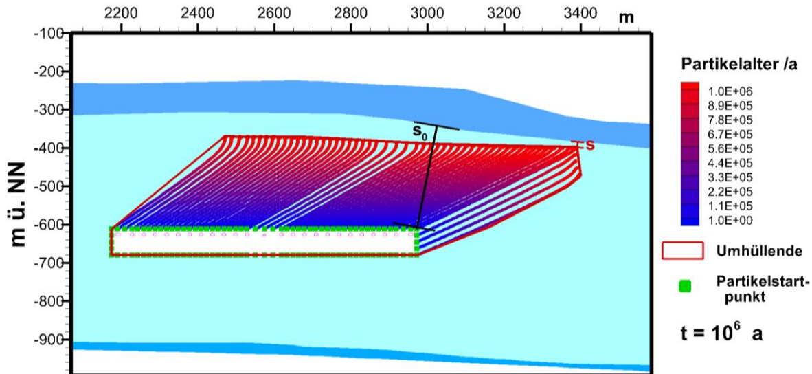
Abb. 47: Variante P2: Auswertung des Indikators Advektion im Wirtsgestein anhand der Verfolgung von Partikeln. Dargestellt sind alle Partikel zum Zeitpunkt 1 Million Jahren
