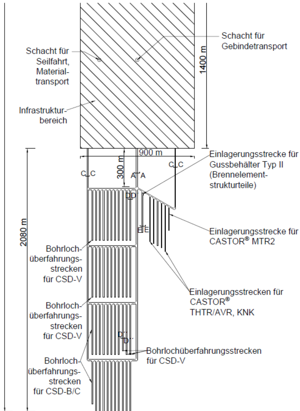
Abb. 17: Skizze des Grubengebäudeteils mit Infrastrukturbereich und Einlagerungsbereichen für Abfälle aus der Wiederaufarbeitung, Brennelementstrukturteile und Abfälle aus Versuchs- und Prototypkernkraftwerken sowie Forschungsreaktoren
