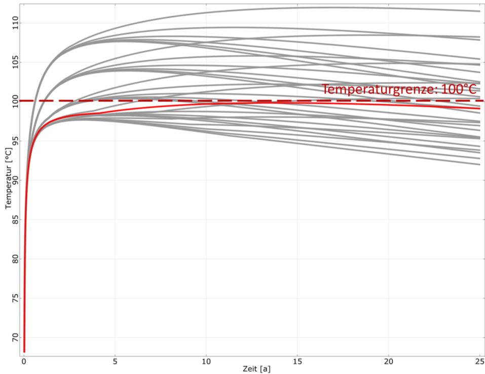
Abb. 10: Temperaturverläufe im Auslegungspunkt für DWR-Mix BE, gewählter Temperaturverlauf (rote Kurve)
