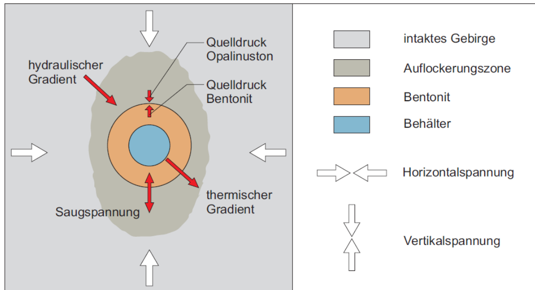
Abb. 20: Prinzipskizze zur Illustration der Prozesse im Bereich eines verfüllten Grubenbaus (ohne geochemische Prozesse) (Nagra, 2002b)
