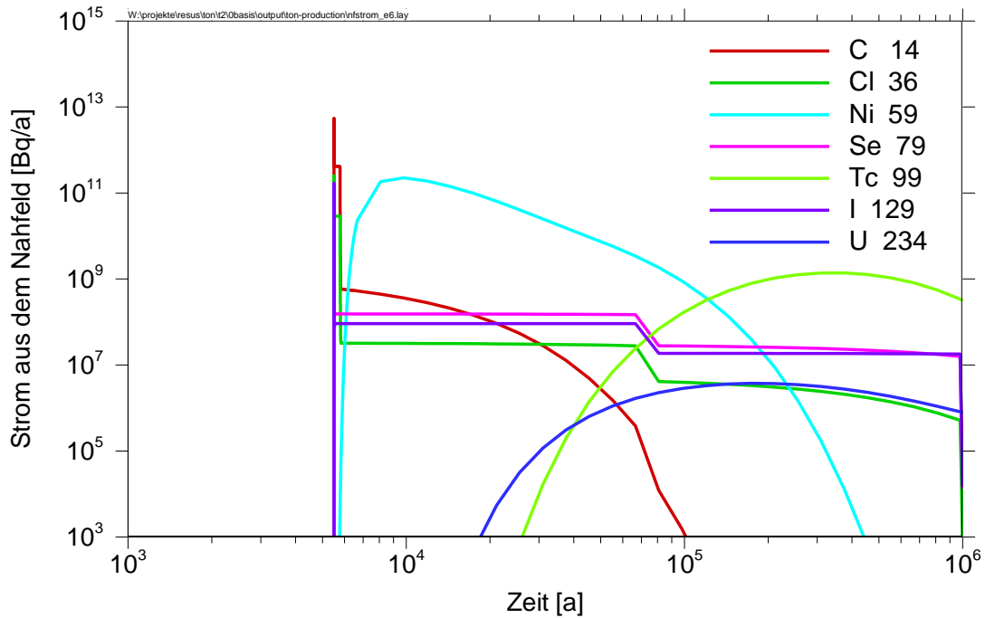
Abb. 39: Radionuklidstrom aus dem Nahfeld in das Wirtsgestein
