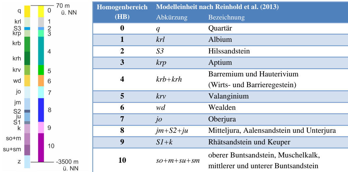
Abb. 24: Modelleinheiten: links: nach geologischer Beschreibung; daneben: für Modellberechnungen mit den Homogenbereichen (HB) 0 bis 10
