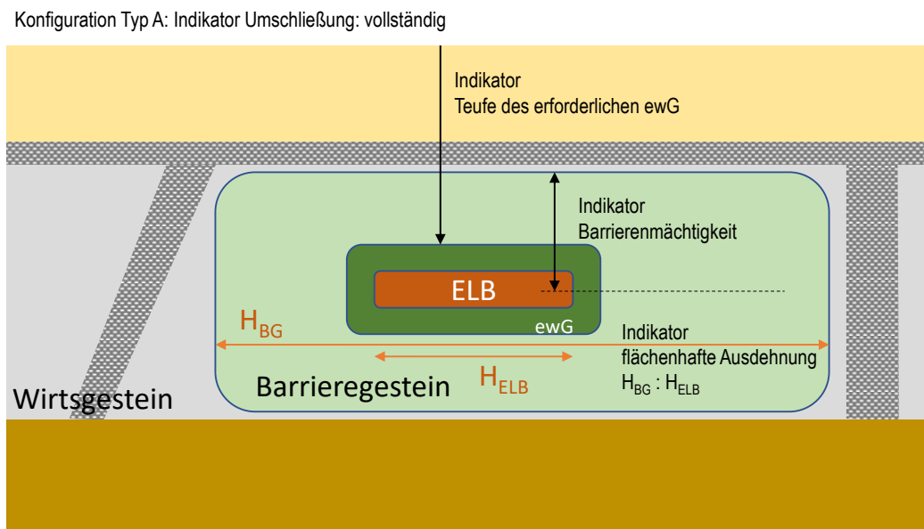
Abb. 50: Indikatoren bei der Konfiguration „ewG im Wirtsgestein“ (Typ A in Anlehnung an die im AkEnd und im Kommissionsbericht abgebildeten und erläuterten Konfigurationstypen); H_{BG} = horizontale Ausdehnung des Barrieregesteins; H_{ELB} = horizontale Ausdehnung des Einlagerungsbereichs; schraffierte Bereiche stellen schematisch Zonen dar, die die Anforderungen an einen ewG nicht erfüllen
