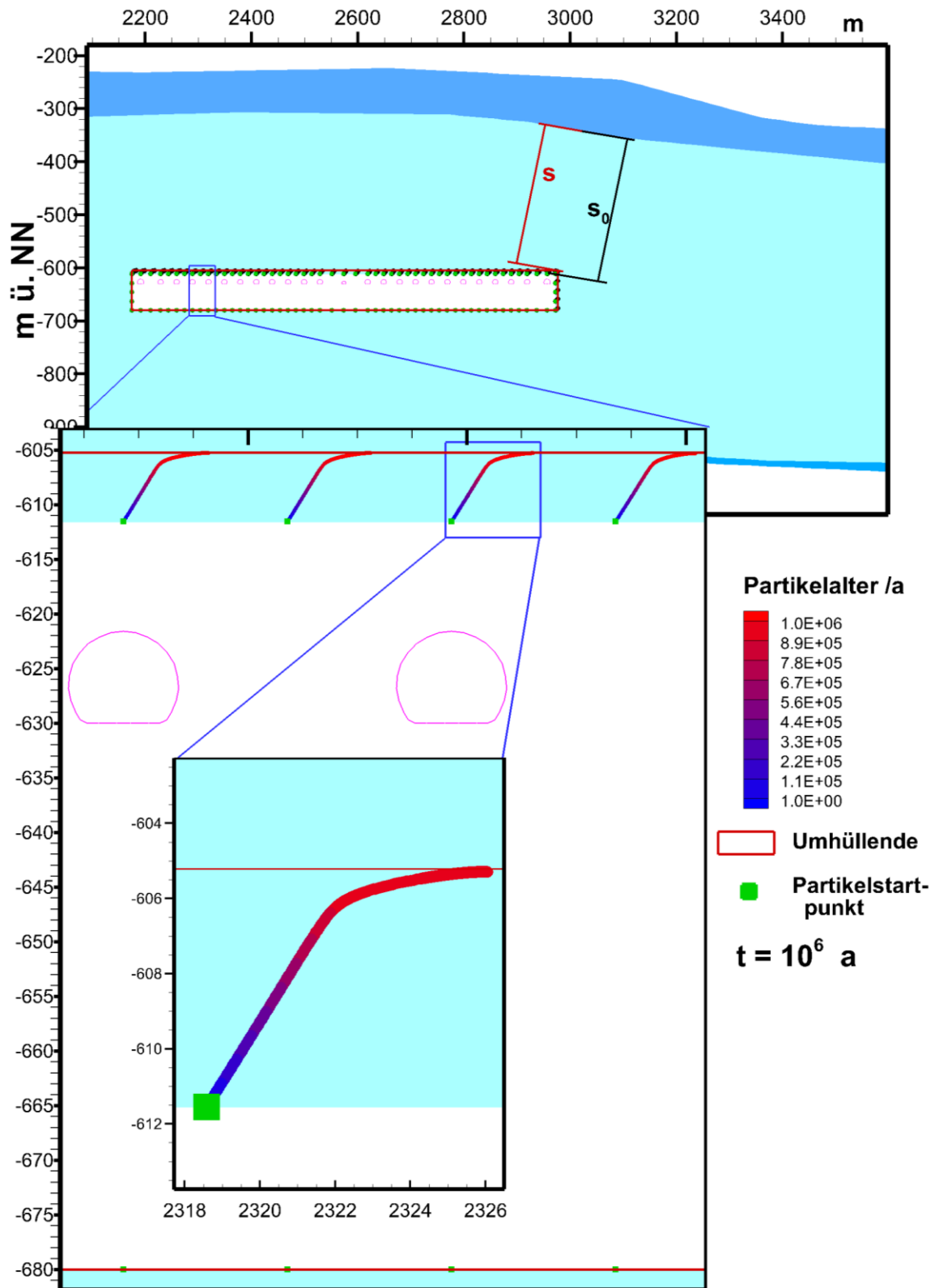
Abb. 46: Variante P1: Auswertung des Indikators Advektion im Barrieregestein anhand der Verfolgung von Partikeln. Dargestellt sind alle Partikel 1 Million Jahre nach Einlagerungsbeginn
