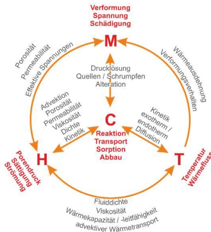
Abb. 23: Prozesse (rot) und deren Kopplungen (orange bzw. schwarz) (Maßmann & Ziefle 2017)
