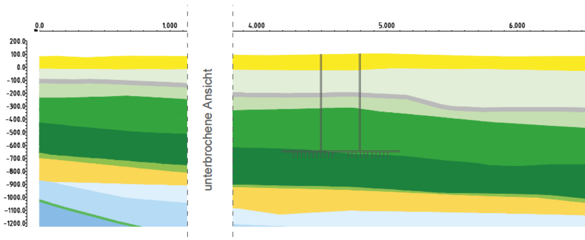
Abb. 6: Ausschnitt aus dem geologischen Modell mit Position des Endlagerbergwerkes
