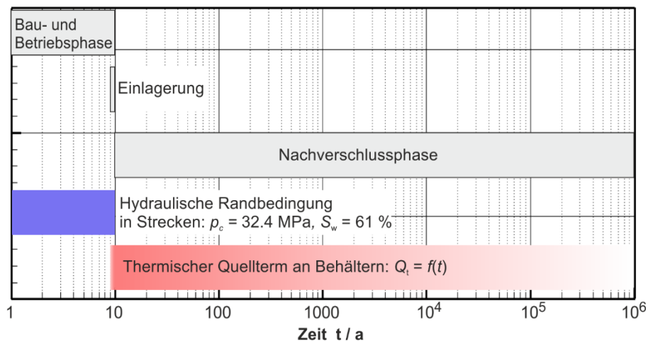
Abb. 27: Zeitliche Phasen des Endlagers und der Randbedingungen des numerischen Modells
