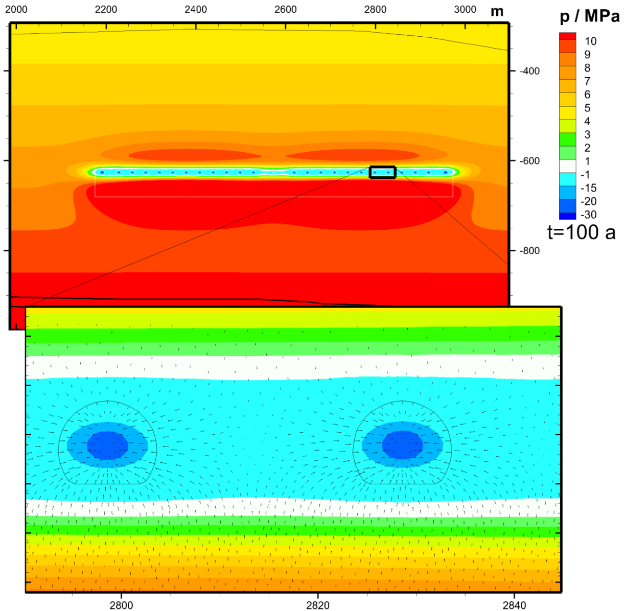
Abb. 30: Porenwasserdruck nach 100 Jahren. Negative Werte entsprechen Saugspannungen in der ungesättigten Zone. Die Vektoren zeigen die Strömungsrichtung und qualitativ die Strömungsgeschwindigkeit
