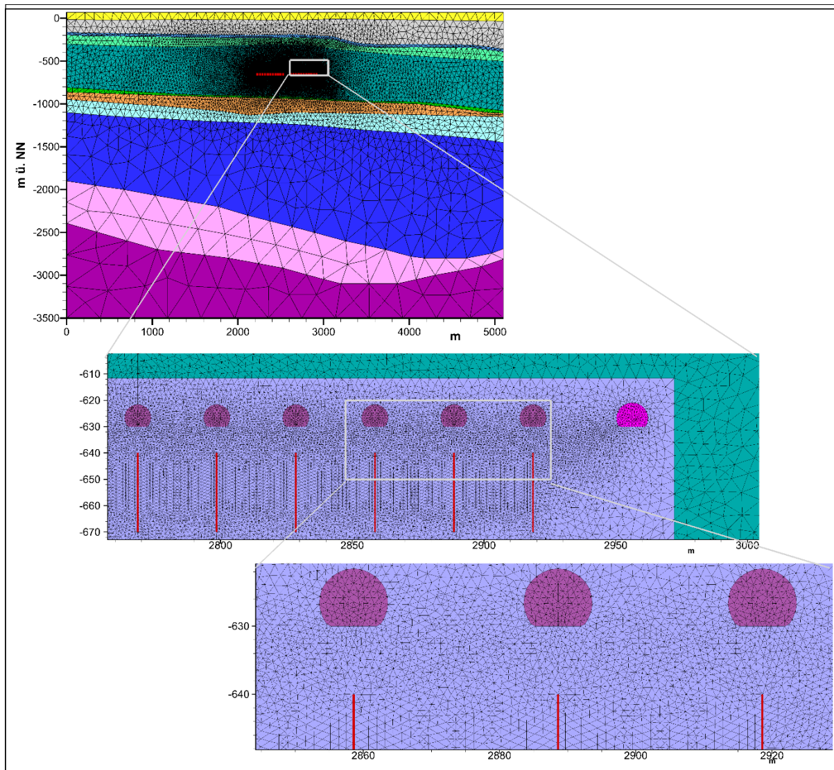
Abb. 26: Numerisches Modell für THM-Berechnungen (Farbgebung der geologischen Einheiten siehe Abb. 26)
