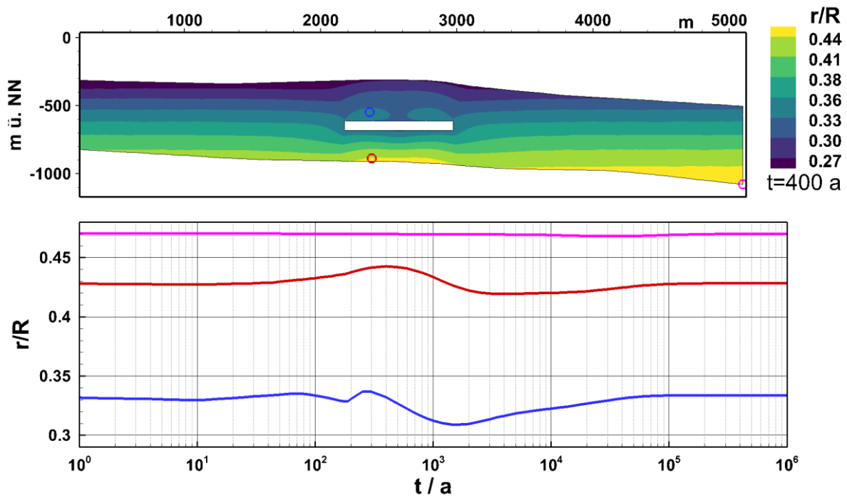
Abb. 42: Variante P1: Örtliche und zeitliche Entwicklung des Indikators Dilatanz (Durchlässigkeitsbeiwert = 1 \cdot 10^{-12} m/s)
