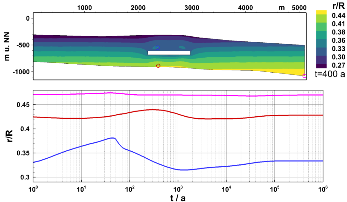
Abb. 43: Variante P2: Örtliche und zeitliche Entwicklung des Indikators Dilatanz (Durchlässigkeitsbeiwert = 1 \cdot 10^{-10} m/s)
