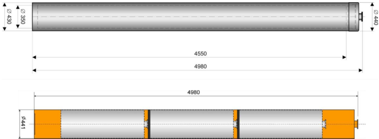
Abb. 9: BSK mit Brennelementen (oben), Triple-Pack mit CSD-V (unten) (Bollingerfehr et al., 2011)
