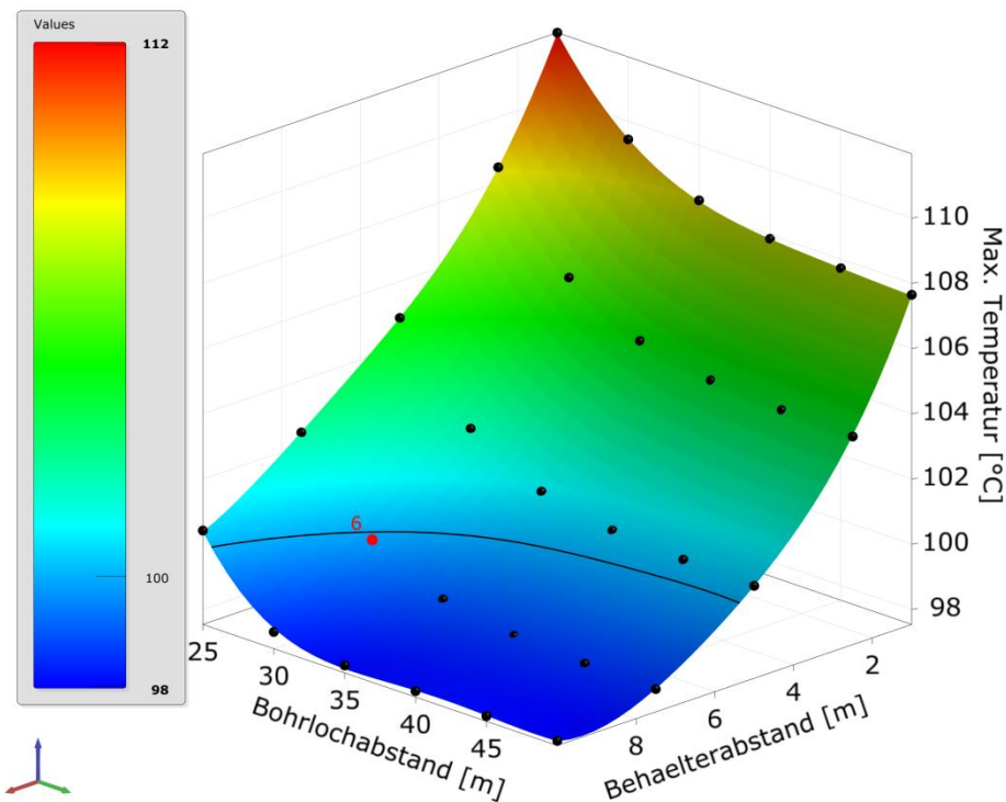
Abb. 11: Temperaturmaximum in Abhängigkeit vom Bohrloch- und Behälterabstand, gewähltes Maximum aus Simulationsfall N° 6 (roter Punkt), schwarze Linie kennzeichnet 100°C-Isotherme
