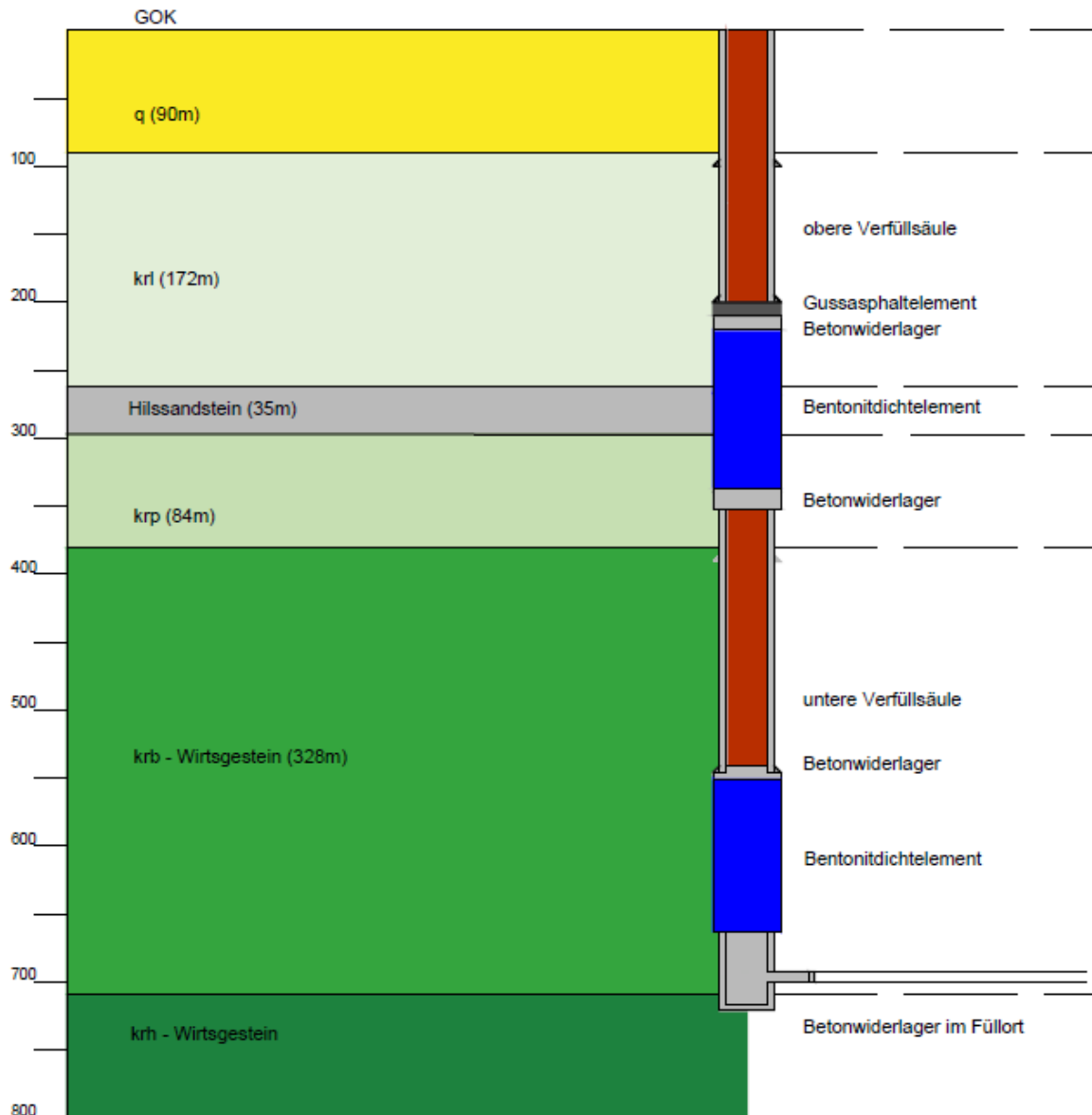
Abb. 19: Schachtverschlusskonzept für das Referenzprofil
