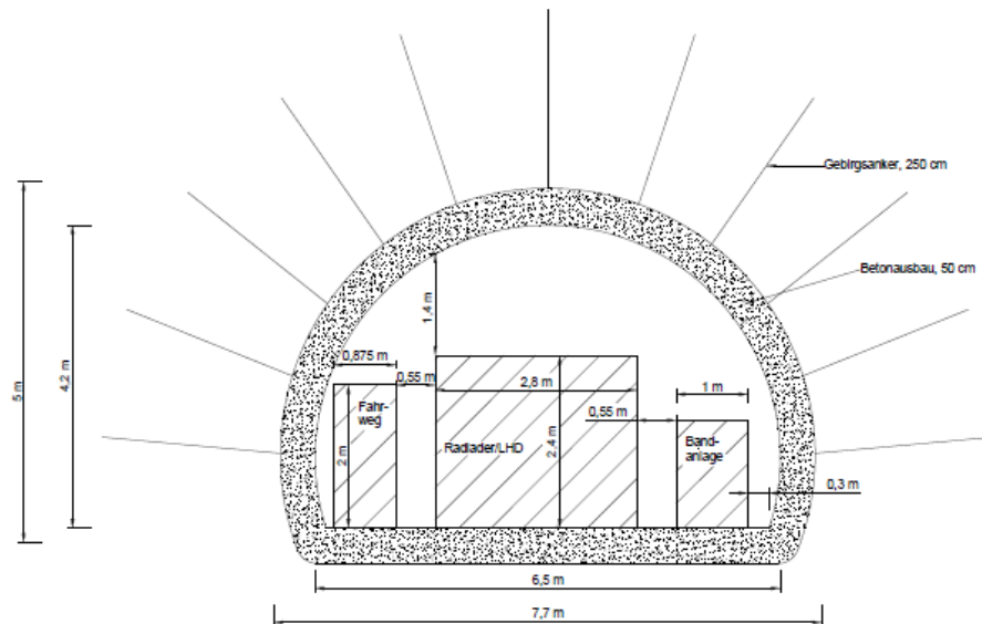
Abb. 13: Skizze der Richtstrecken des Endlagerbergwerks (s. Abb. 16 und Abb. 17 fur die Lage der Strecken anhand der Querschnittbezeichnungen)
