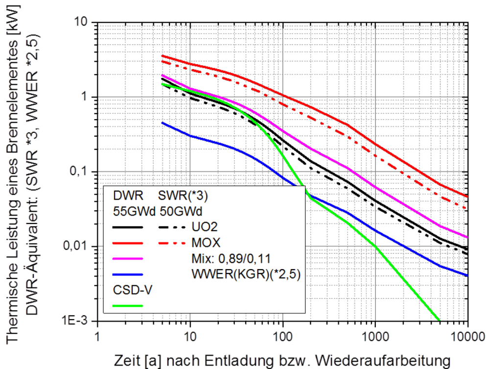
Abb. 7: Thermische Leistung eines DWR-Brennelementes in Abhängigkeit von der Zeit, beladungsäquivalent zu einem DWR-BE (3 SWR-BE oder 2,5 WWER-BE)
