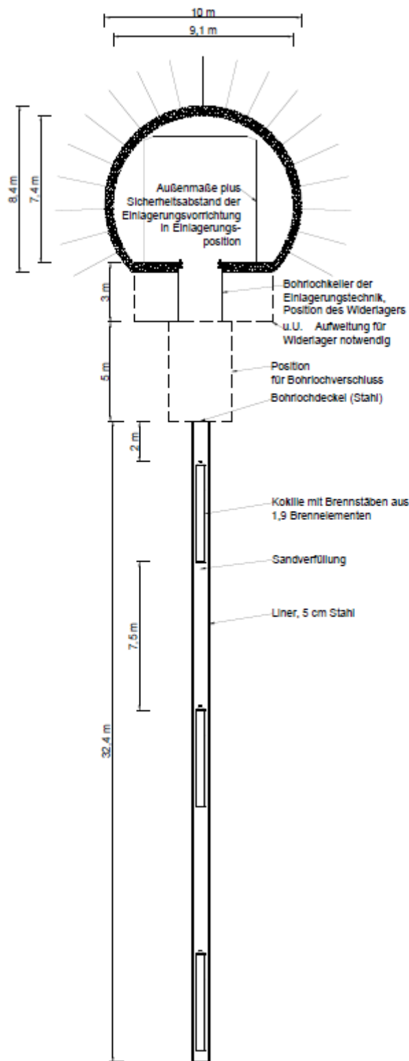
Abb. 14: Skizze des Querschnitts einer Bohrlochüberfahrungsstrecke und eines Bohrloch (s. Abb. 16 und Abb. 17 für die Lage der Strecken anhand der Querschnittbezeichnungen)
