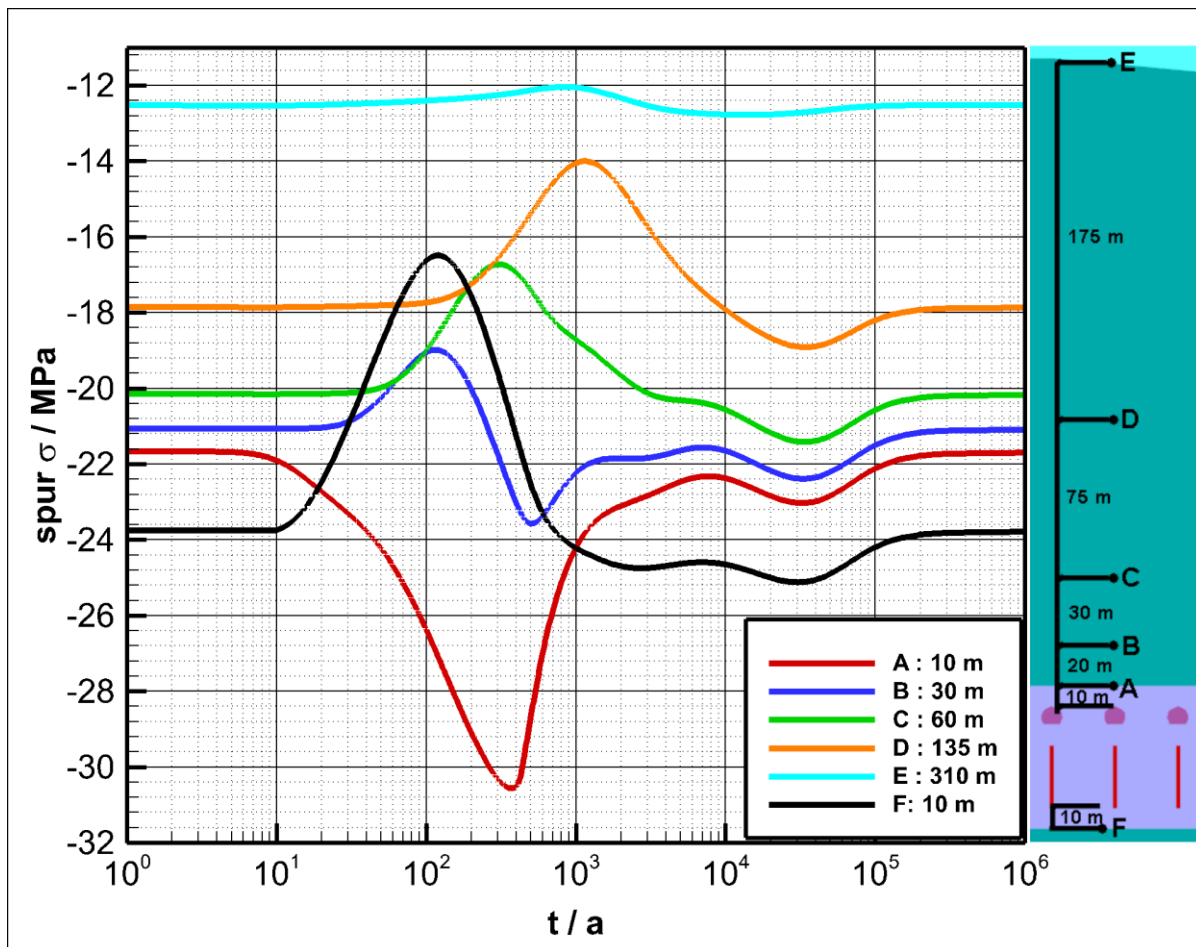
Abb. 34: Zeitliche Entwicklung der Spannungen an ausgewählten Punkten über dem Einlagerungsbereich. Angegeben sind die Entfernungen zur Firste der Strecken, bzw. dem Bohrlochtfesten (Punkt E entspricht der Oberkante des Barrieregesteins)
