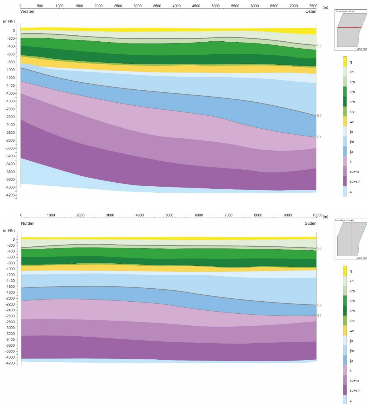
Abb. 3: Schnitt Richtung W-E (oben) und N-S (unten) durch das generische geologische Modell für das Endlagersystem T1 (Abkürzungen siehe Abb. 2) (aus Reinhold et al., 2016)
