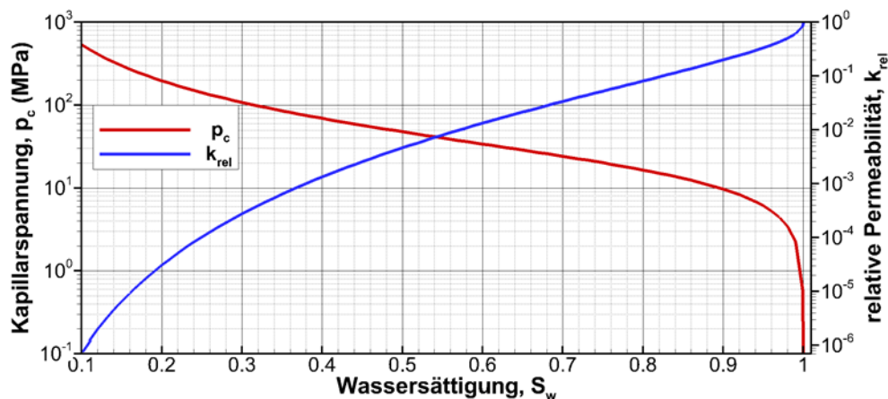
Abb. 25: Kapillardruck-Sättigungsbeziehung und relative Permeabilität-Sättigungsbeziehung im Barrieregestein
