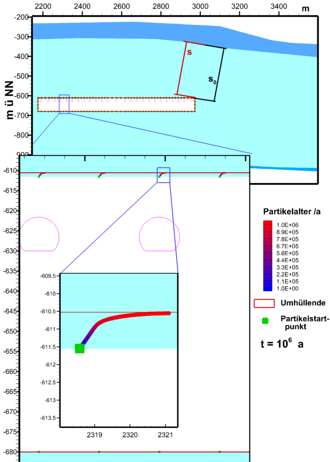
Abb. 37: Auswertung des Advektions-Kriteriums im Barrieregestein anhand der Verfolgung von Partikelbahnen. Dargestellt sind die Startpunkte (grün), die Umhüllende (rot) und die Partikel 1 Million Jahre nach Einlagerungsbeginn
