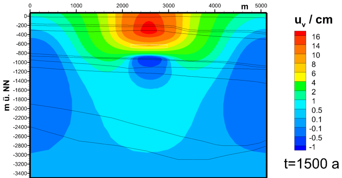
Abb. 33: Vertikale Verschiebungskomponente nach 1.500 Jahren
