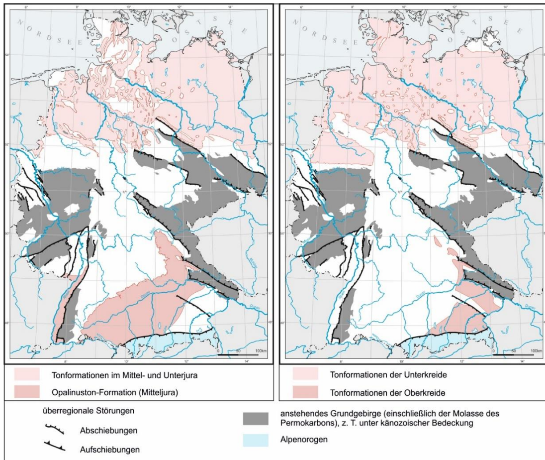
Abb. 1: Schematische Verbreitungsgebiete von Tonformationen in Deutschland ohne spezifische Bewertung, links: Mittel- und Unterjura, rechts: Unter- und Oberkreide (nach Hoth et al., 2007)
