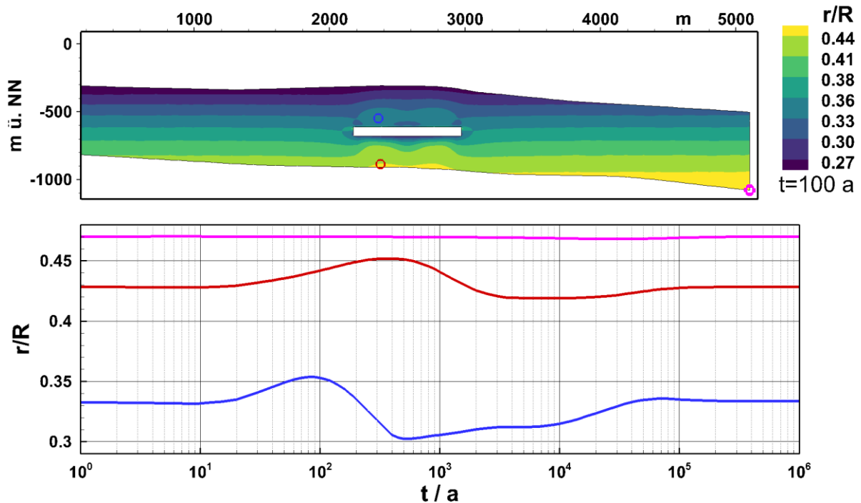
Abb. 35: Örtliche und zeitliche Entwicklung des Indikators Dilatanz im Barrieregestein
