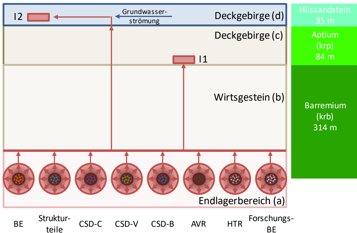
Abb. 38: Schematische Darstellung des Modells für das Endlager im Tongestein (links) und der Stratigraphie der Gesteine (rechts) (nicht maßstabsgerecht)
