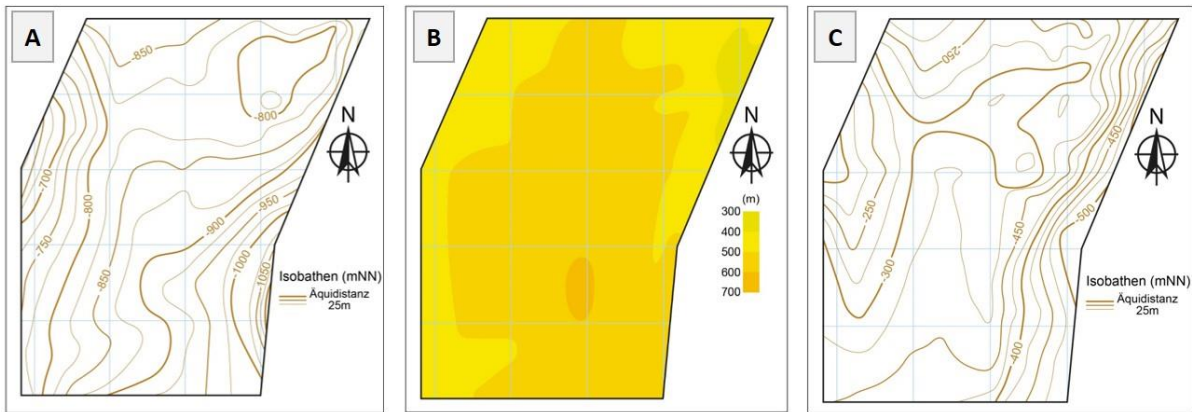
Abb. 4: A = Basis der Modelleinheit Hauterivium (Basis Wirts- bzw. Barrierestein), B = Mächtigkeit des Wirts- bzw. Barrierestein, C = Top der Modelleinheit Barremium (Top Wirts- bzw. Barrierestein) (Gitterlinienabstand 2 km), (aus Reinhold et al., 2016)
