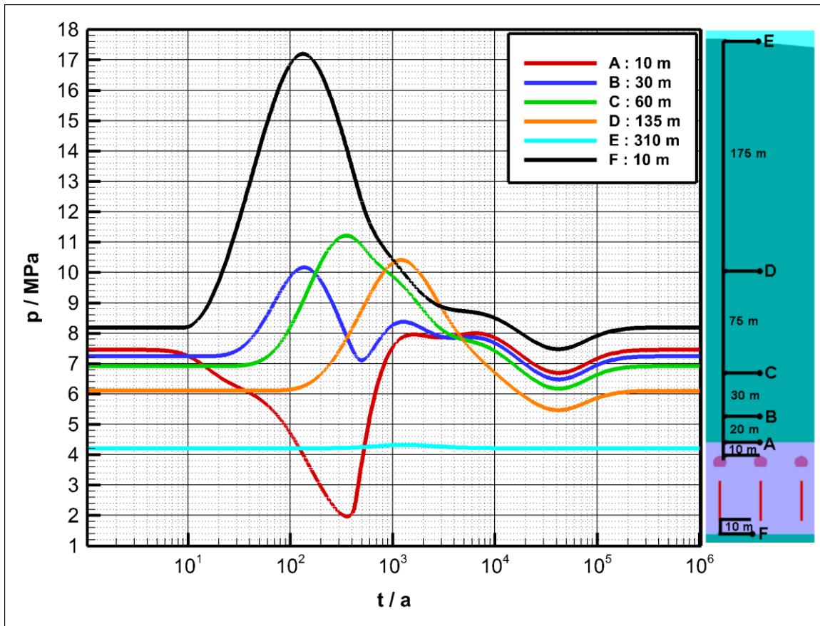
Abb. 31: Zeitliche Entwicklung der Porenwasserdrücke an ausgewählten Punkten über dem Einlagerungsbereich. Angegeben sind die Entfernungen zur Firste der Strecken, bzw. dem Bohrloch tiefsten (Punkt E entspricht der Oberkante des Barrieregesteins)
