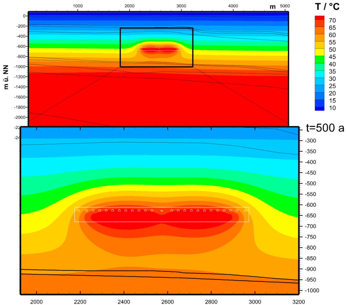
Abb. 29: Temperaturverteilung nach 500 Jahren
