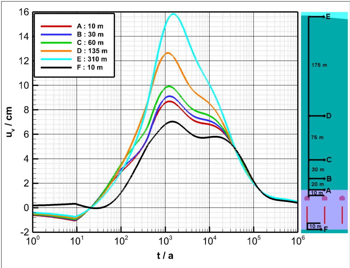
Abb. 32: Zeitliche Entwicklung der vertikalen Verschiebungen an ausgewählten Punkten im Barrieregestein. Angegeben sind die Entfernungen zur Firste der Strecken, bzw. dem Bohrloch tiefsten (Punkt E entspricht der Oberkante des Barrieregesteins)
