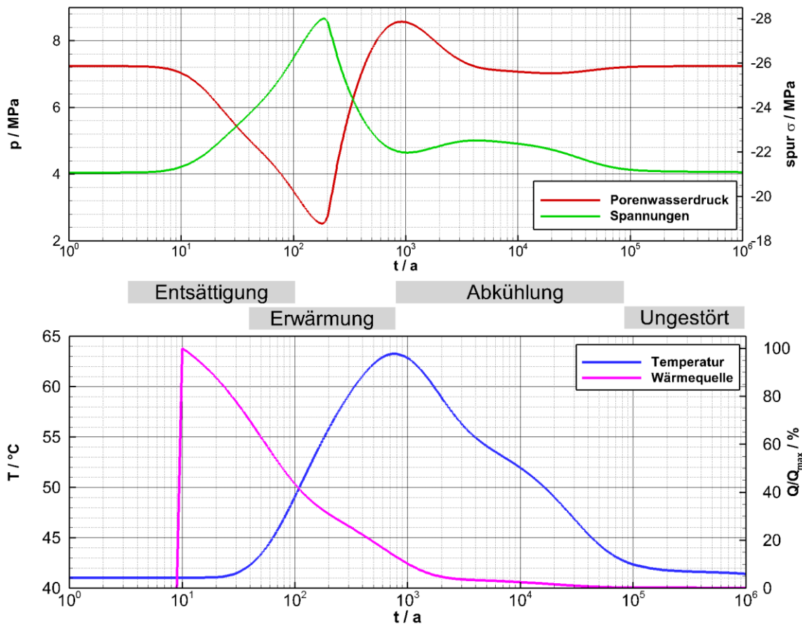
Abb. 41: Berechnete zeitliche Entwicklung des gekoppelten THM-Systems; beispielhaft dargestellt an einem Punkt im Wirtsgestein
