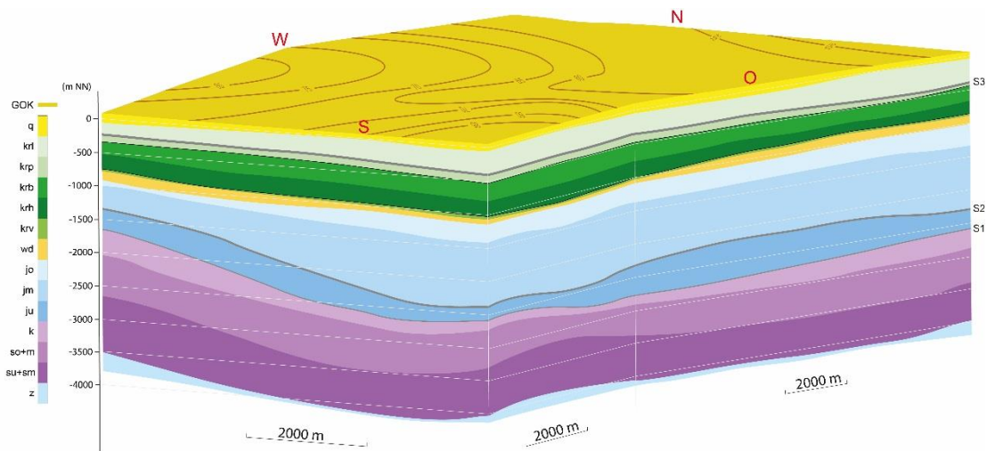
Abb. 2: 3D-Blockbild der Modelleinheiten im generischen geologischen Modell T1 „Tongestein größerer Mächtigkeit“ (Abk. z = Zechstein, su+sm = Unterer und Mittlerer Buntsandstein, so+m = Oberer Buntsandstein und Muschelkalk, k = Keuper, ju = Unterjura, jm = Mitteljura, jo = Oberjura, wd = Wealden, krw = Valanginium, krh = Hauterivium, krb = Barremium, krp = Aptium, krl = Albium, q = Quartär, GOK = Geländeoberkante, S1 = Rhätsandstein, S2 = Aalensandstein, S3 = Hilssandstein) (aus Reinhold et al., 2016)
