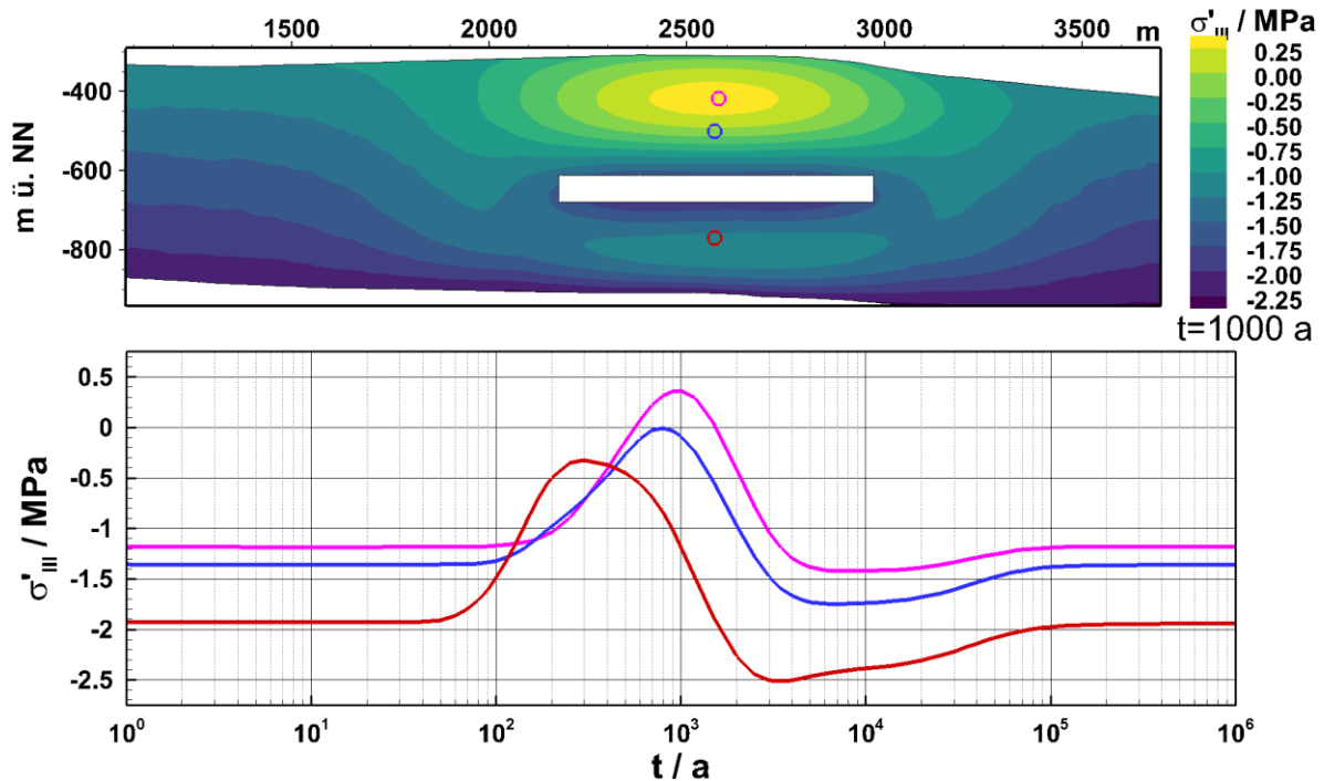
Abb. 44: Variante P1: Örtliche und zeitliche Entwicklung des Indikators Fluiddruck (Durchlässigkeitsbeiwert = 1 \cdot 10^{-12} m/s)
