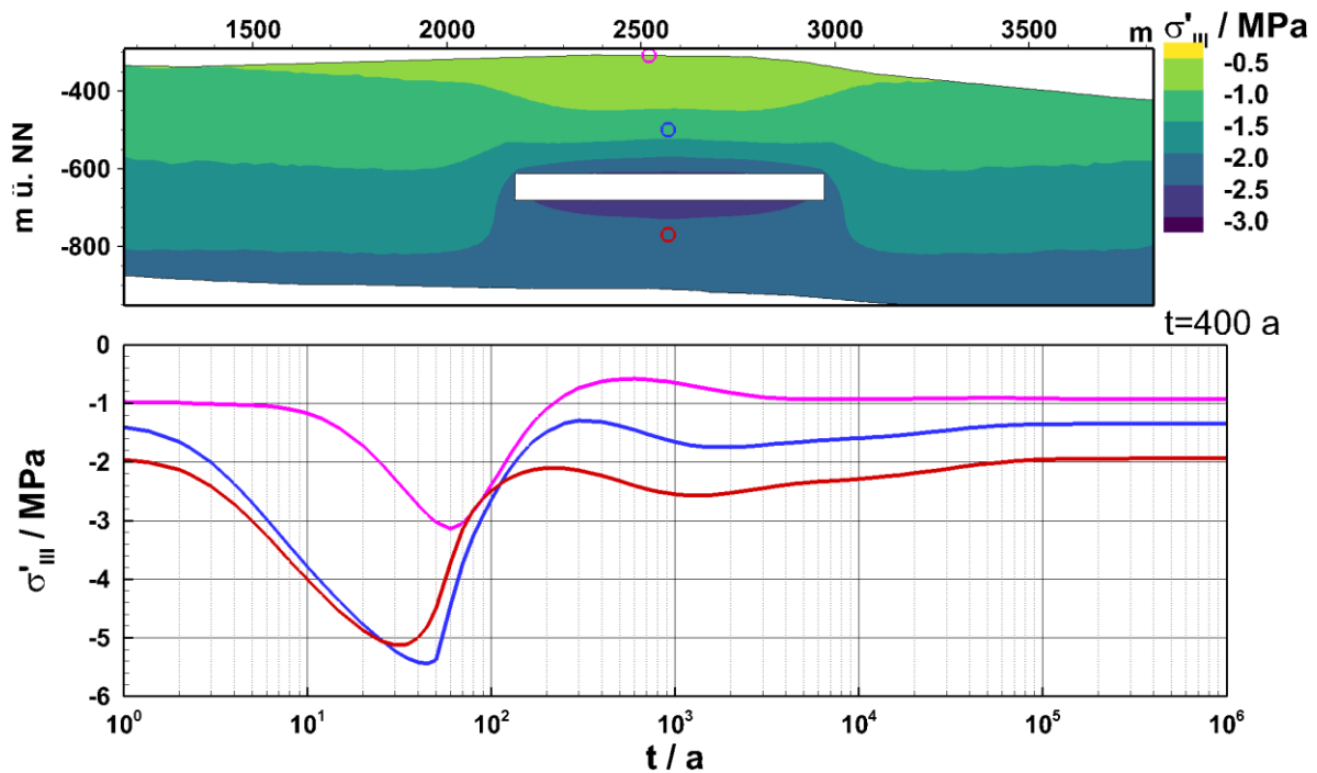
Abb. 45: Variante P2: Örtliche und zeitliche Entwicklung des Indikators Fluiddruck (Durchlässigkeitsbeiwert = 1 \cdot 10^{-10} m/s)
