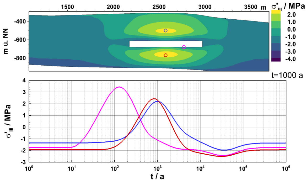
Abb. 36: Örtliche und zeitliche Entwicklung des Indikators Fluiddruck
