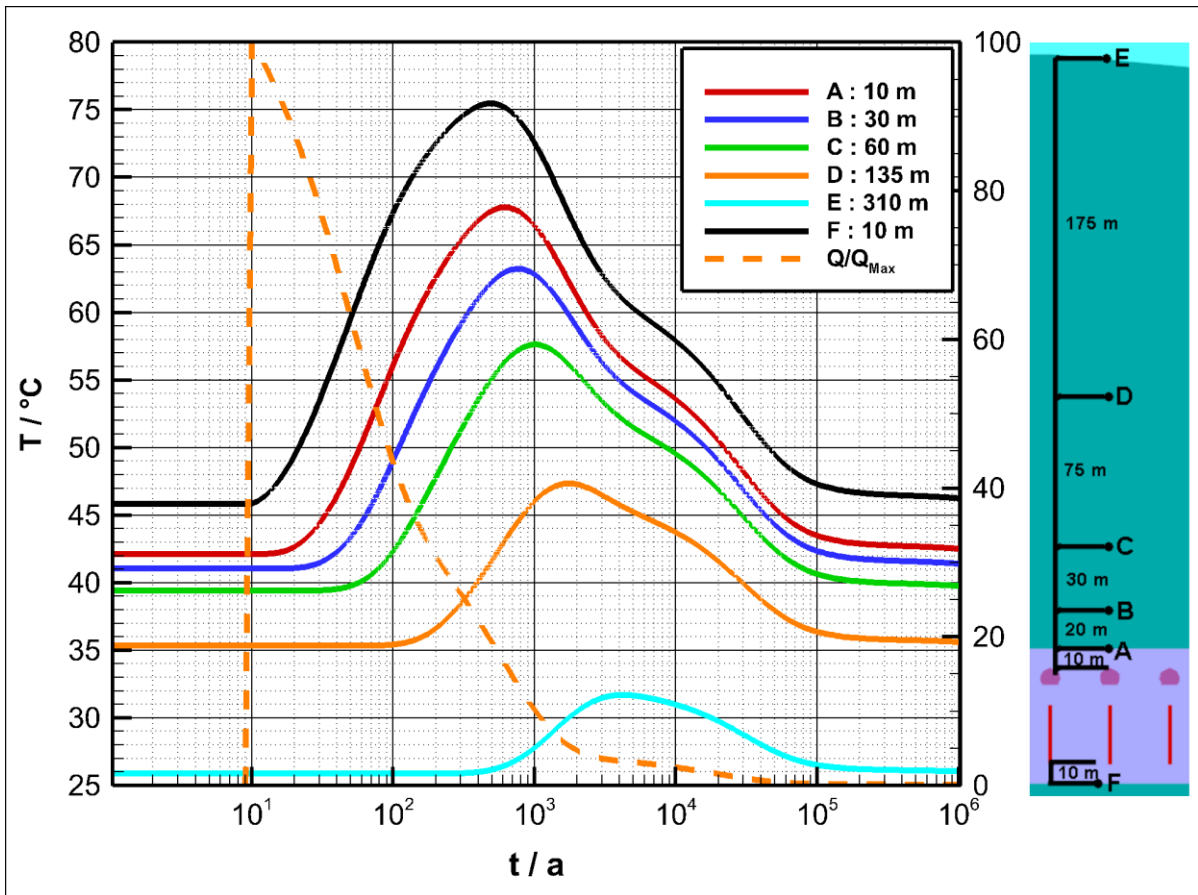
Abb. 28: Zeitliche Entwicklung der Temperatur an ausgewählten Punkten im Barrieregestein. Angegeben sind die Entfernungen zur Firste der Strecken, bzw. dem Bohrlochtiefsten (Punkt E entspricht der Oberkante des Barrieregesteins)
