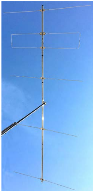
LFA-6M 5EL: $494.95
