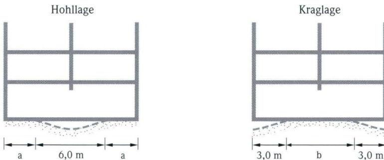
Abb. 40. Erdfall unter dem Haus Hinz (Bl. 4923 Altmorschen). Neben dem Wegbrechen ganzer Bauwerksteile erfahren die Gründung und das Bauwerk Verformungen durch starke Hohl- (Frei-) und Kraglagen (Foto: PICKEL 1963).
