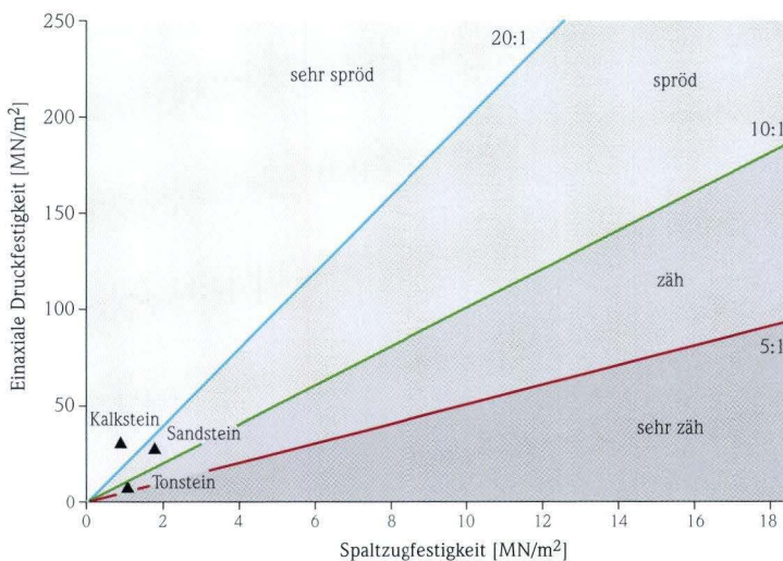
Abb. 7. Sprödes bzw. zähes Verhalten der untersuchten Gesteinsarten in Abhängigkeit vom Verhältnis \sigma_D/\sigma_Z .
