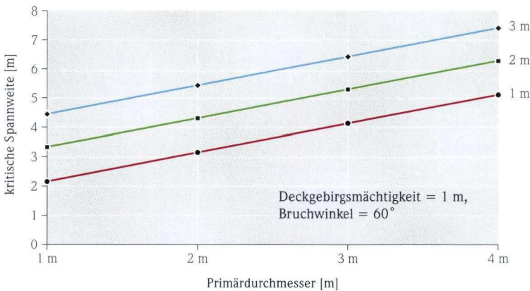
Abb. 16. Berechnete kritische Spannweiten in Abhängigkeit von der Deckgebirgsmächtigkeit zwischen 1 bis 3 m und den in Hessen am häufigsten vorkommenden Primärdurchmesser der Erdfälle.
