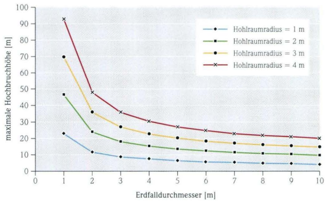
Abb. 10. Maximale Hochbruchhöhe eines Hohlraumes an die Erdoberfläche bei aus Naturbefunden bekannten primären Erdfalldurchmessern und Hohlraumhöhen.
