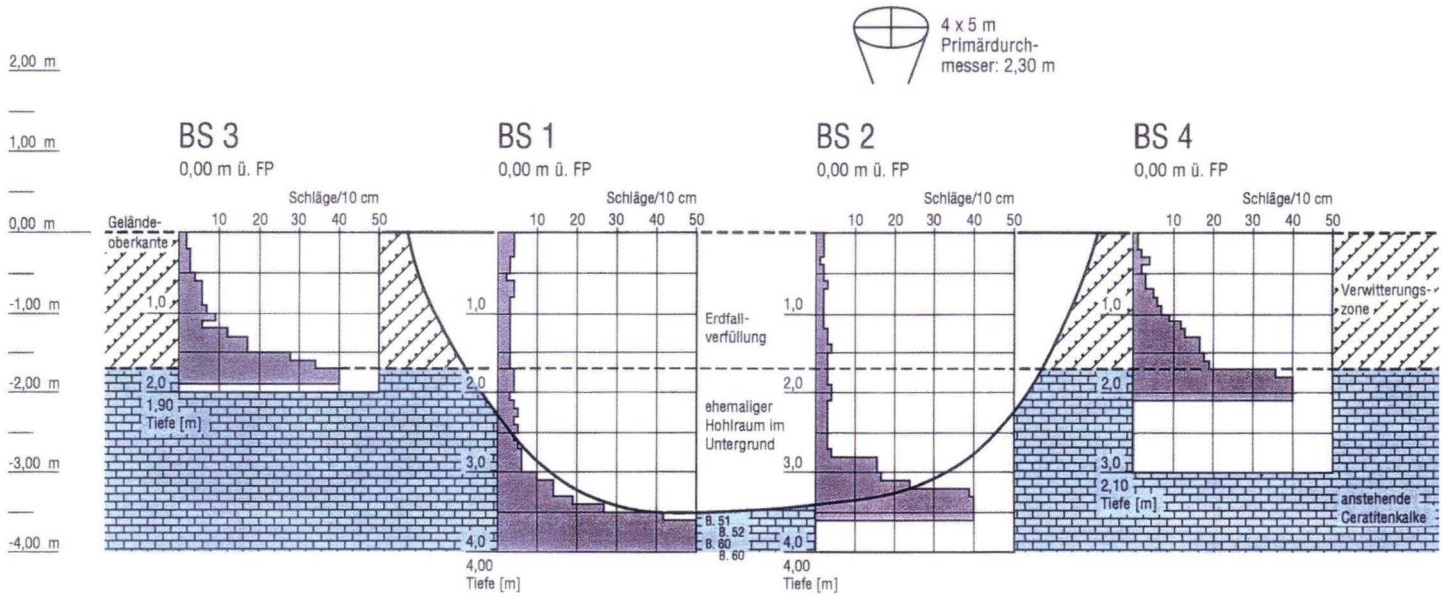
Abb. 18. Unterirdischer Hohlraum in Ceratitenschichten des mo2 unter 1,50 m mächtigem Verwitterungslehm. Die geringen Schlagzahlen charakterisieren den nachgebrochenen Lehm, die hohen Schlagzahlen den Übergang zum Ceratitenkalk.
