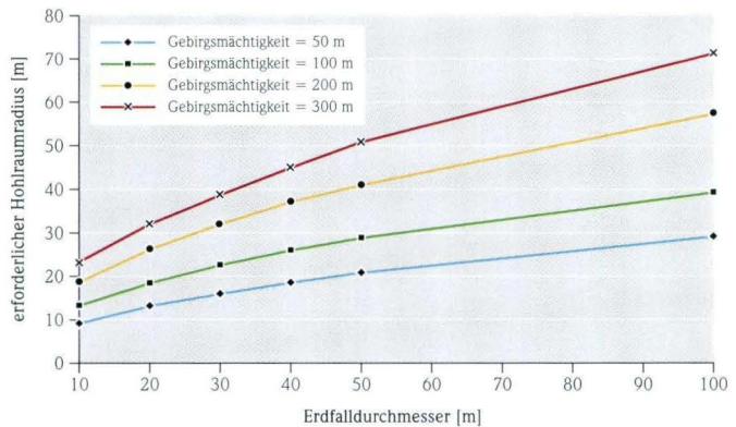
Abb. 11. Erforderlicher Hohlraumradius bei definierter Gebirgsmächtigkeit und primären Erdfalldurchmessern für den potenziellen Hochbruch an die Erdoberfläche.
