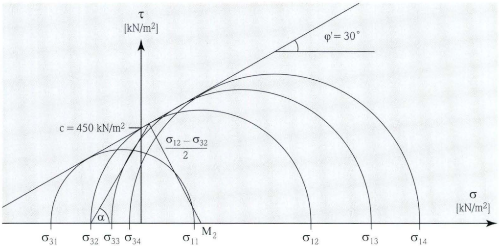
Abb. 8. Mohr'sches Bruchkriterium für spröde Sandsteine der Calförde-Folge für Überlagerungshöhen von 10, 30, 40 und 50 m. Die für die Berechnung angesetzten Scherparameter wurden in Triaxialversuchen im Labor ermittelt ( c' = 450 \text{ kN/m}^2 , \varphi' = 30^\circ , \gamma' = 27 \text{ kN/m}^3 ).
