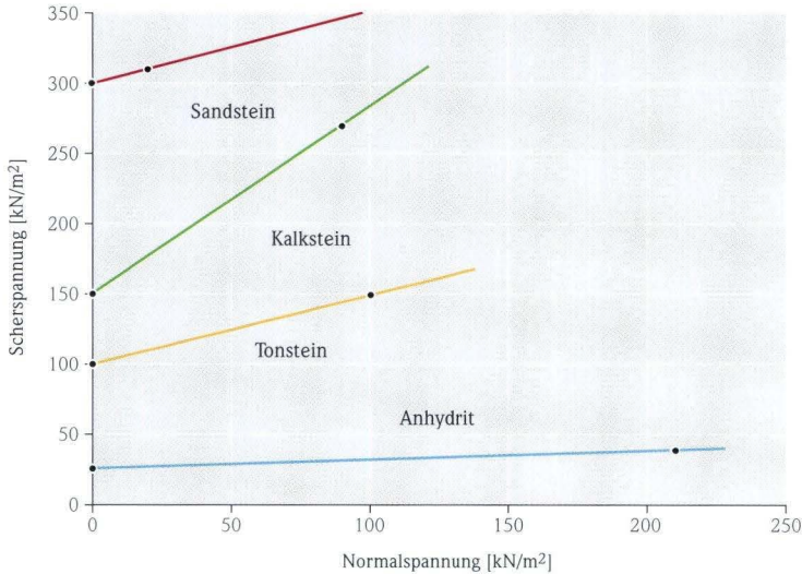
Abb. 6. Schergeraden der untersuchten Gesteinsserien.
