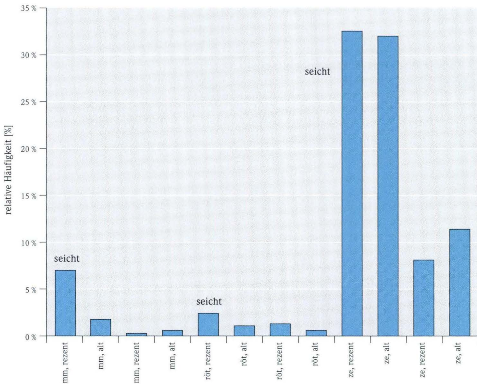
Abb. 25. Prozentuale Verteilung der Erdfallereignisse in Abhängigkeit von der Stratigraphie sowie der Tiefenlage des verkarstbaren Gesteins (n = 3.284).
