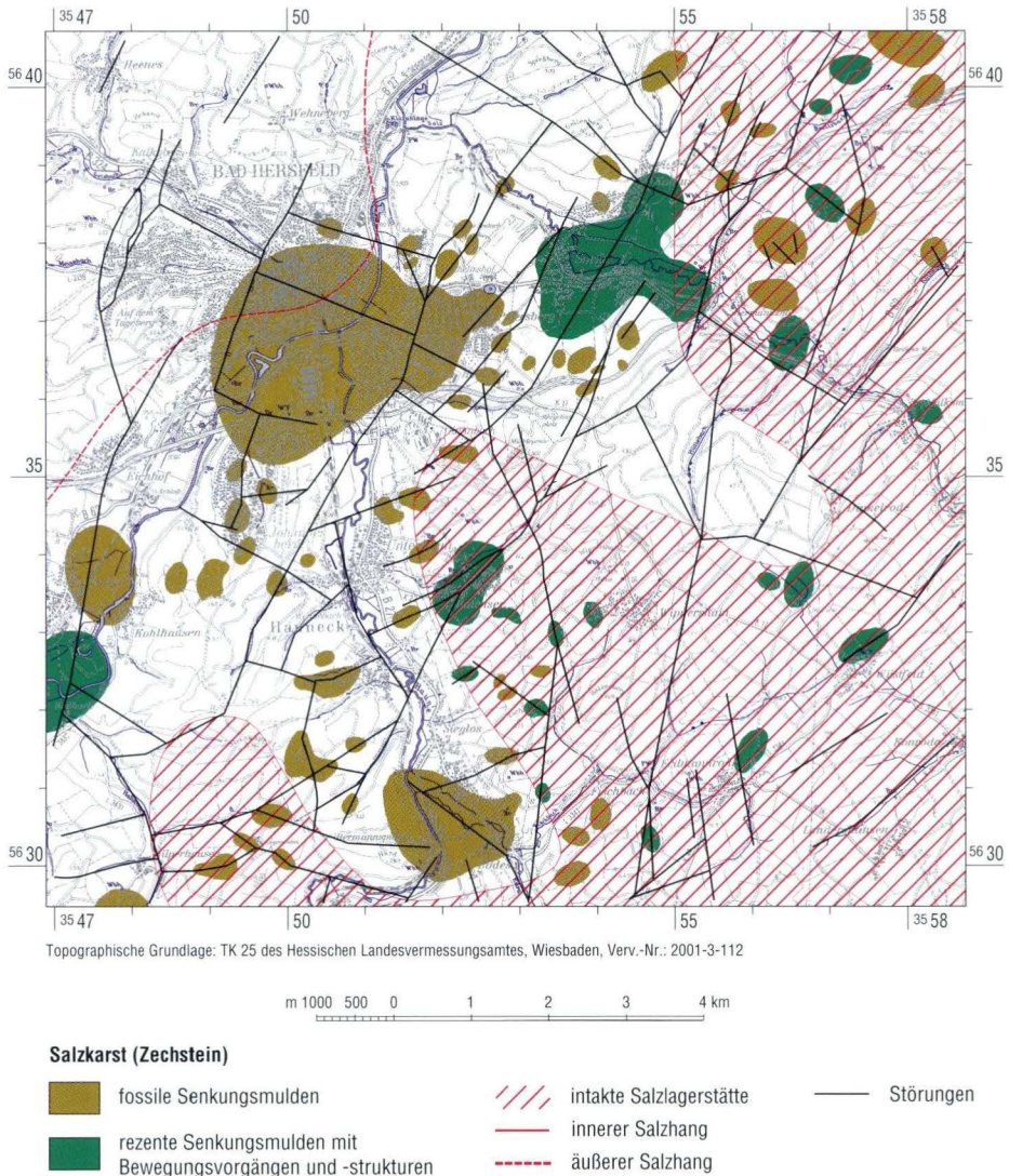
Abb. 27. Orientierung von Senkungsmulden entlang des Salzhanges sowie entlang von Störungen (beispielhaft für das Bl. 5124 Bad Hersfeld).
