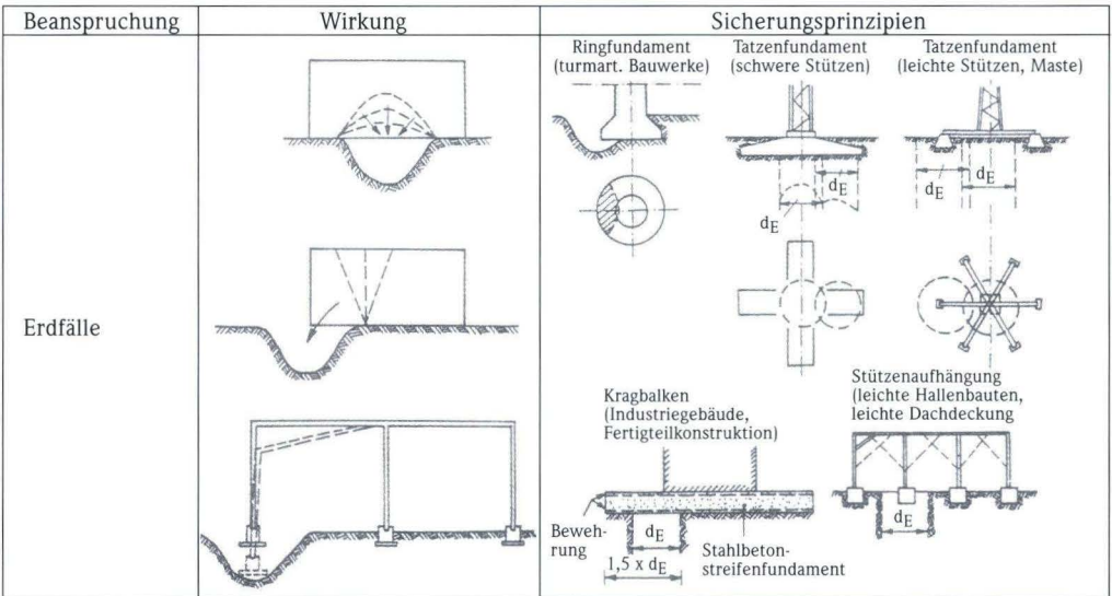
Abb. 46. Beeinflussung von Bauwerken und Sicherungsprinzipien bei Erdfällen (nach KAMMERER 1962).
