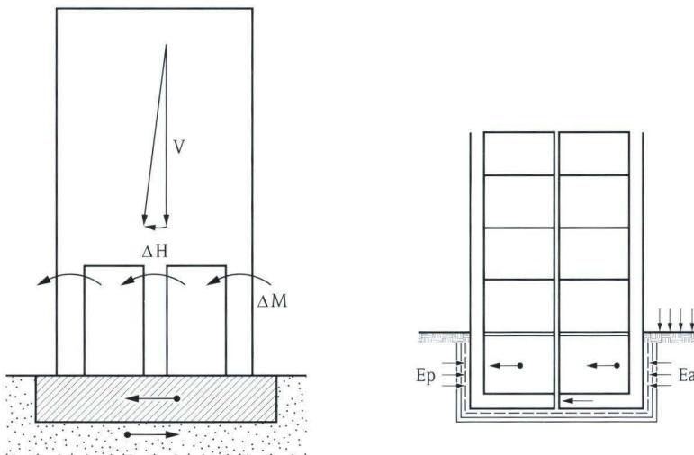
Abb. 38. Wirkung einer Schiefelage bei schlanken Gebäuden und Bauwerken in Dichtungswannen (SMOLTZYK 1992).
