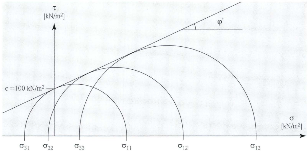
Abb. 9. Mohr'sches Bruchkriterium für plastische Tonsteine des Oberen Röt für Überlagerungshöhen von 5, 10 und 15 m. Die für die Darstellung angesetzten Scherparameter wurden in Triaxialversuchen im Labor ermittelt ( c' = 100 \text{ kN/m}^2 , \varphi' = 27^\circ , \gamma' = 28 \text{ kN/m}^3 ).
