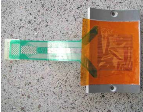
Bild 87: Druckmessfolie
